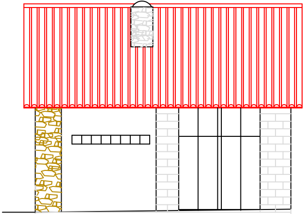
FAÇANA EST
