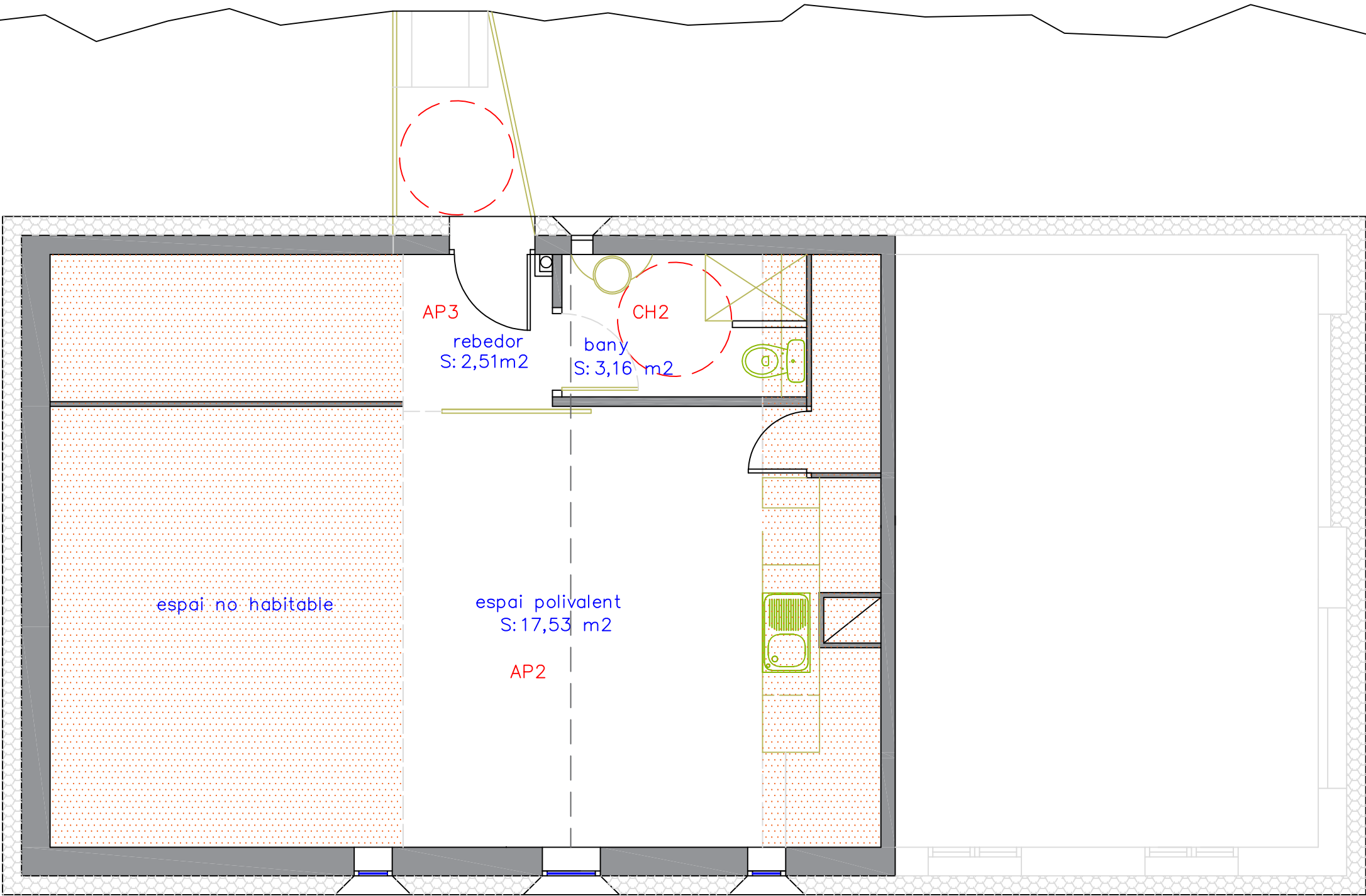
PLANTA PIS
