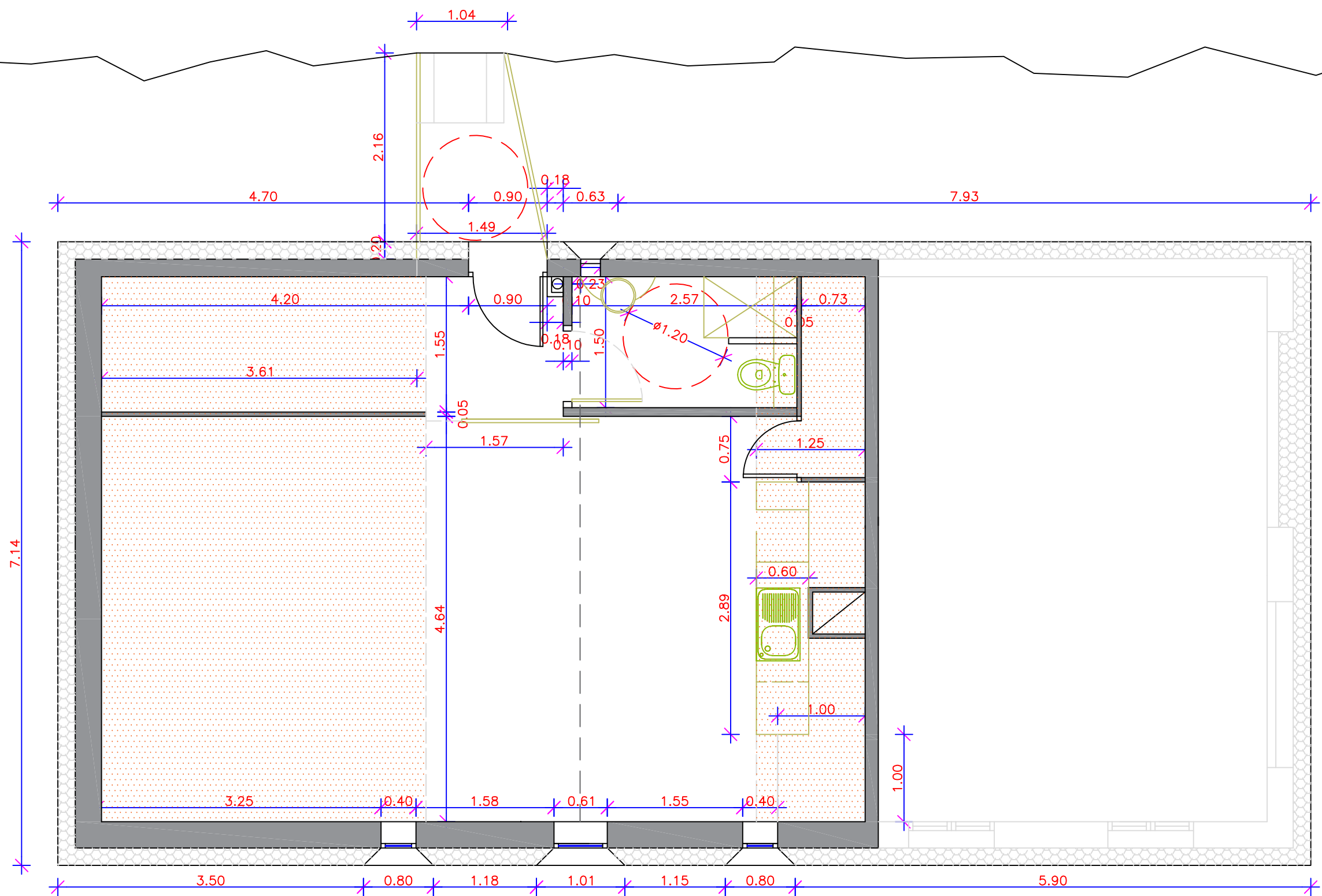
PLANTA PIS
