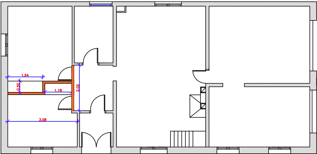
PLANTA BAIXA
