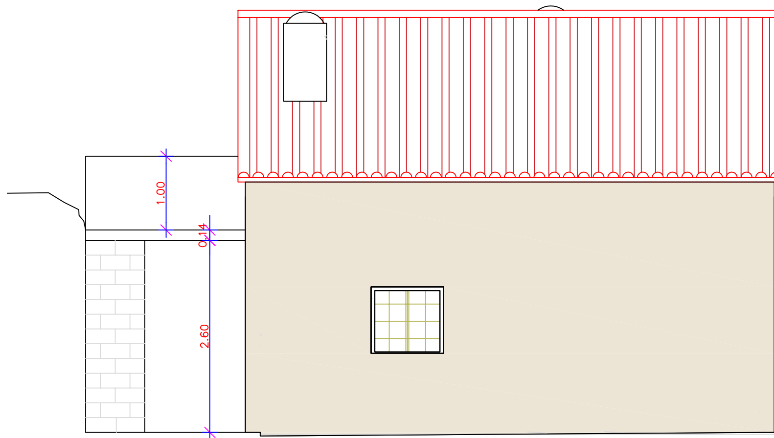
FAÇANA OEST
