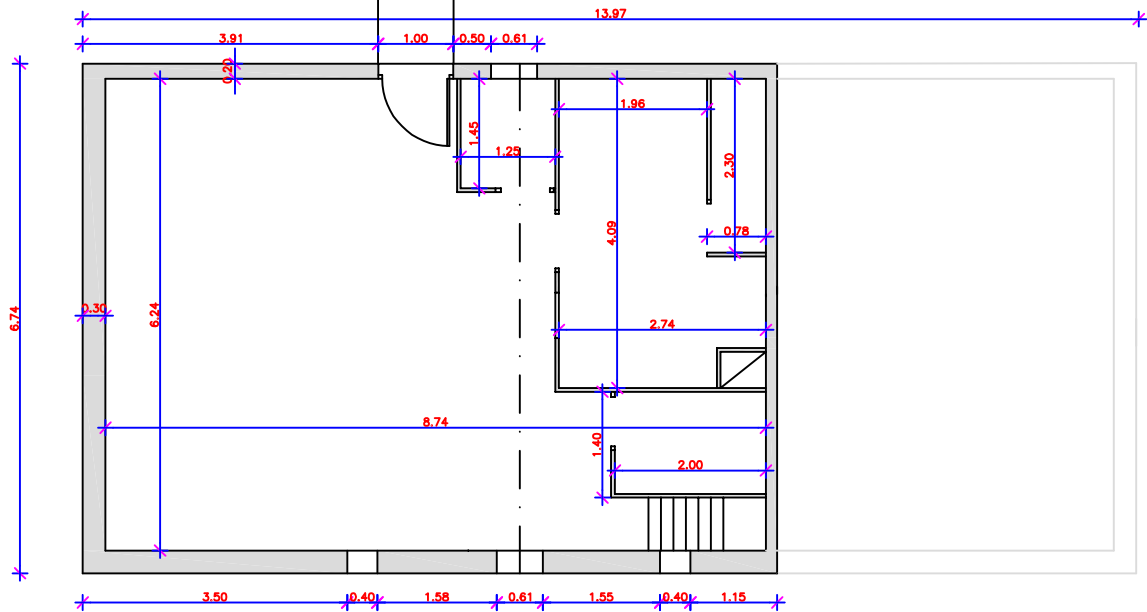
PLANTA PIS
