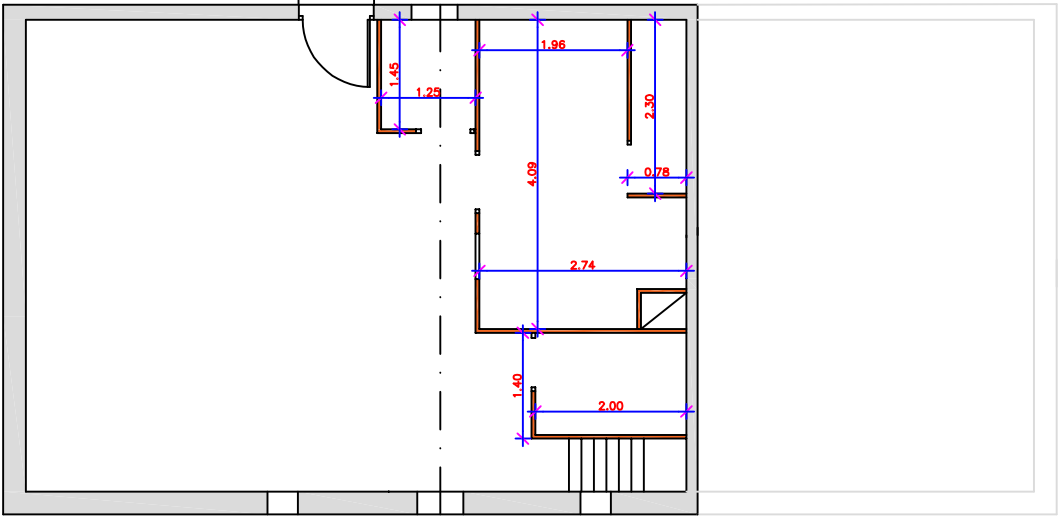
PLANTA PIS
