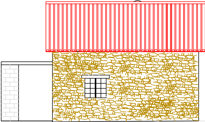
FAÇANA OEST
