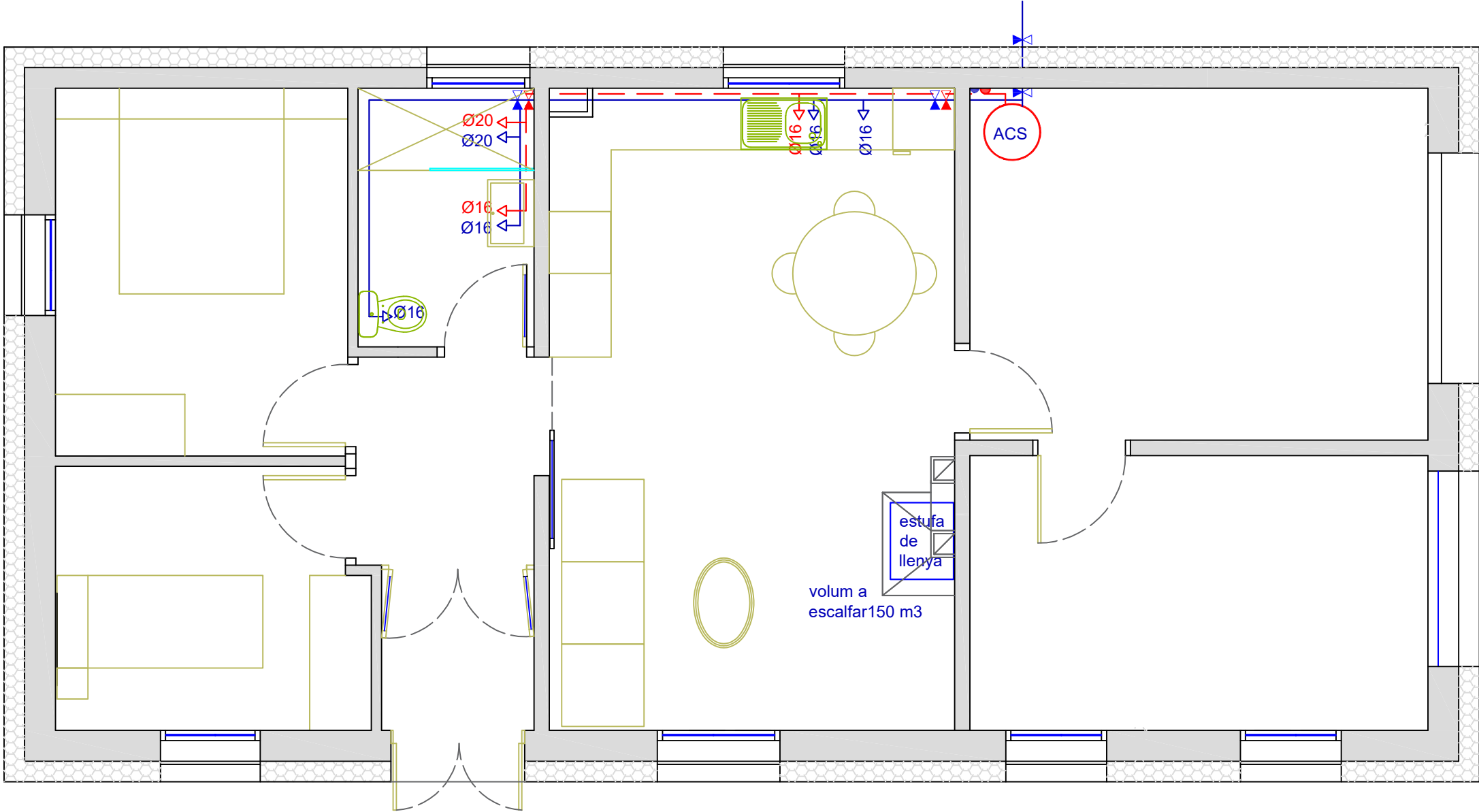
PLANTA BAIXA
