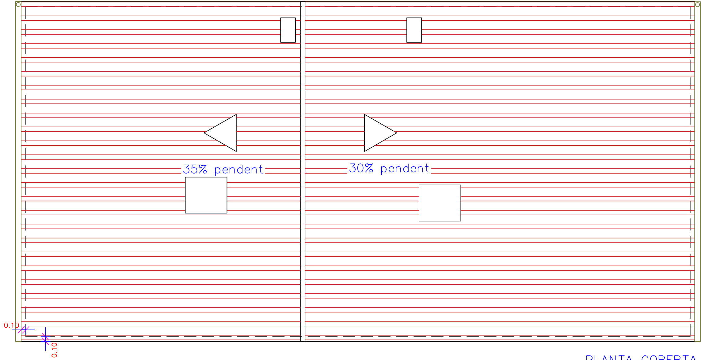
PLANTA COBERTA
