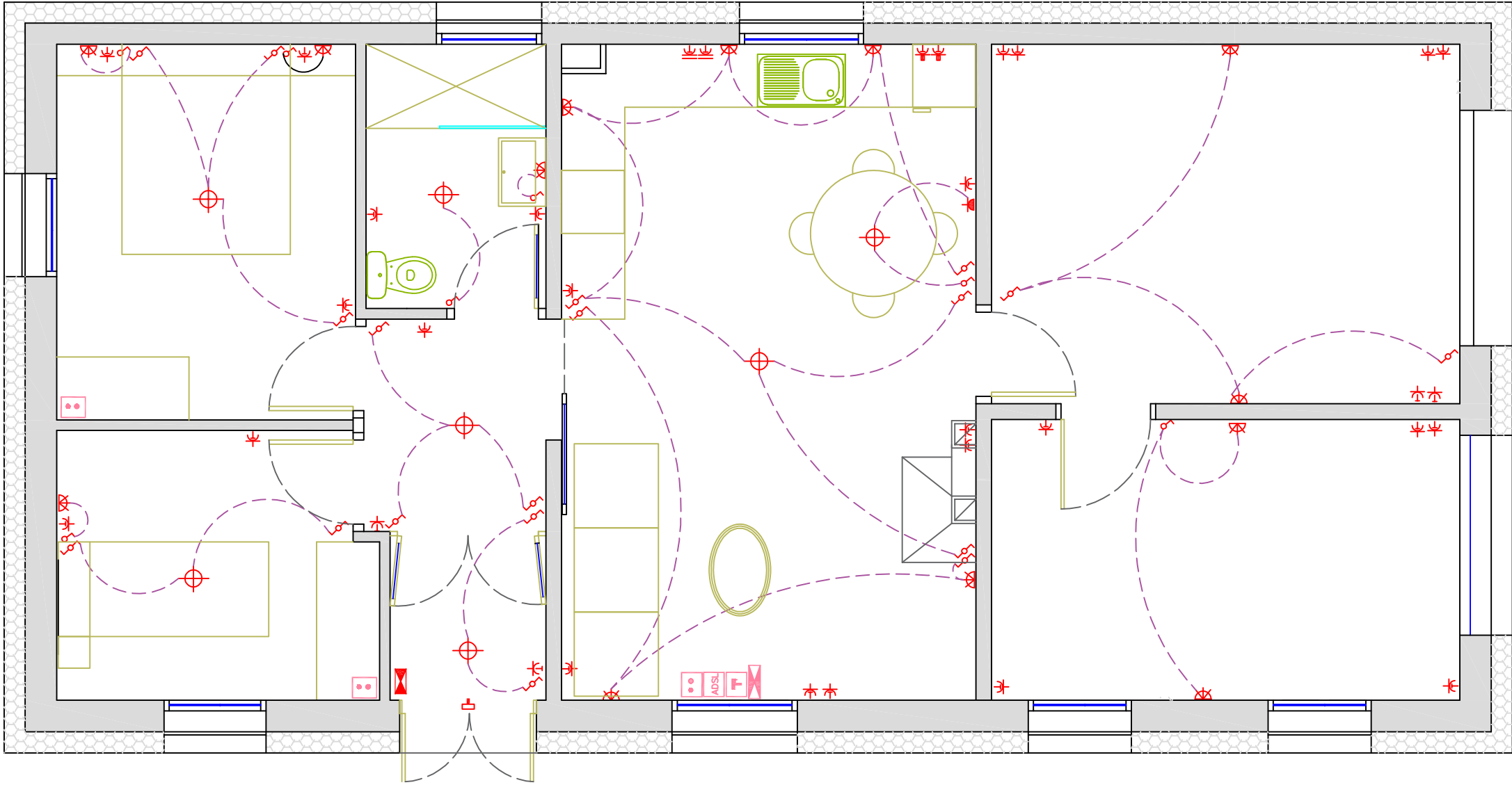
PLANTA BAIXA
