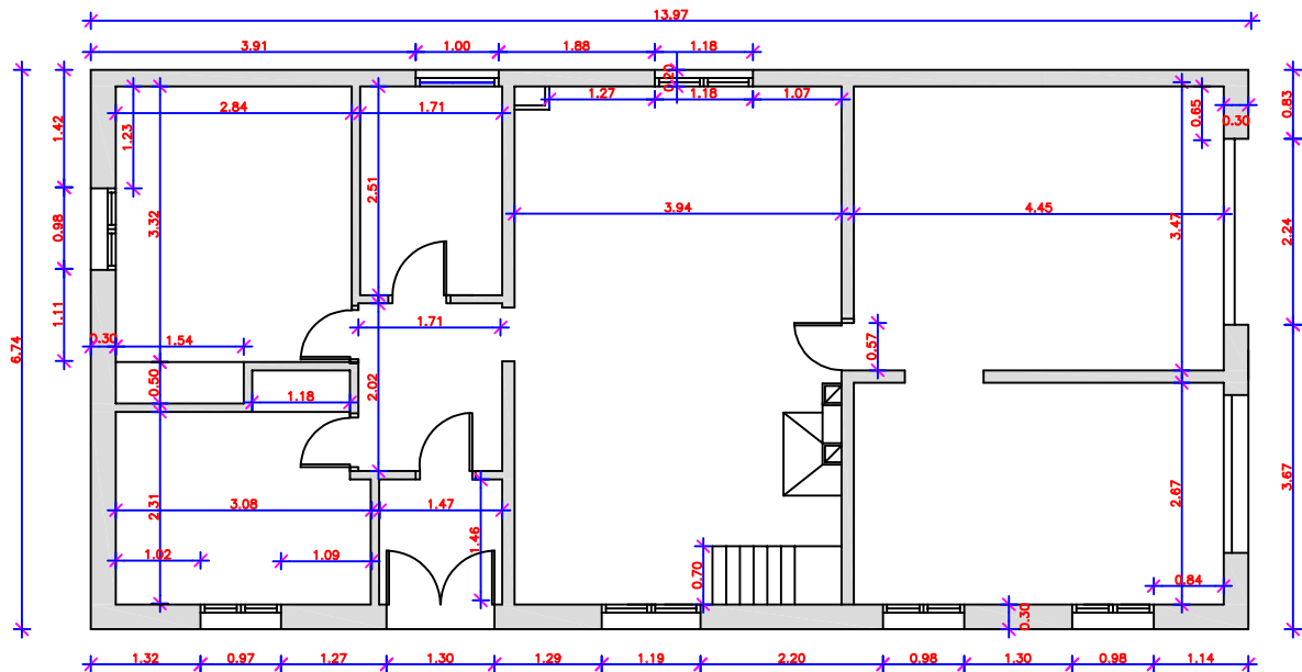
PLANTA BAIXA
