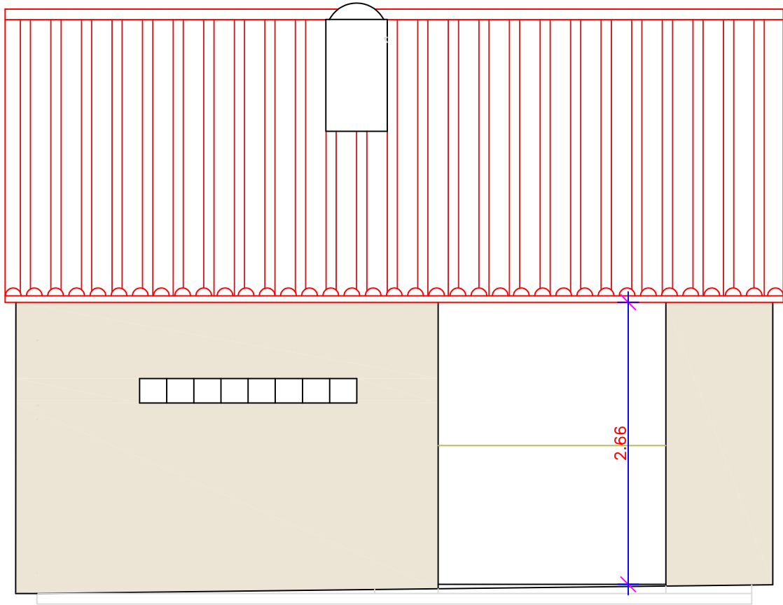
FAÇANA OEST
