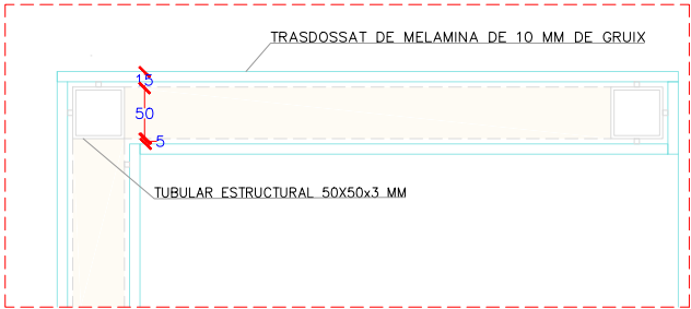
DETALL 1:5 (cotes en mm)
