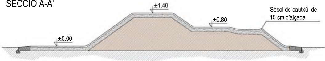
SECCIÓ A-A'
