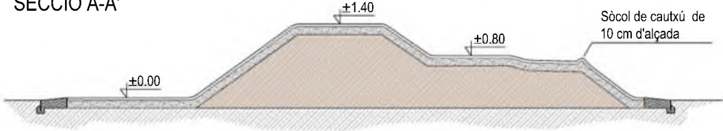
SECCIÓ A-A'
