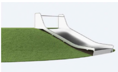
5 Tobogan metàl·lic ample per una alçada d'1.50 m. i una amplada de 2 m. per col·locar sobre turó.
