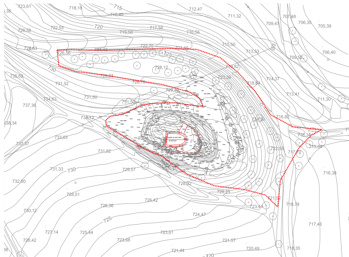
EMPLAÇAMENT Esc. 1/500
