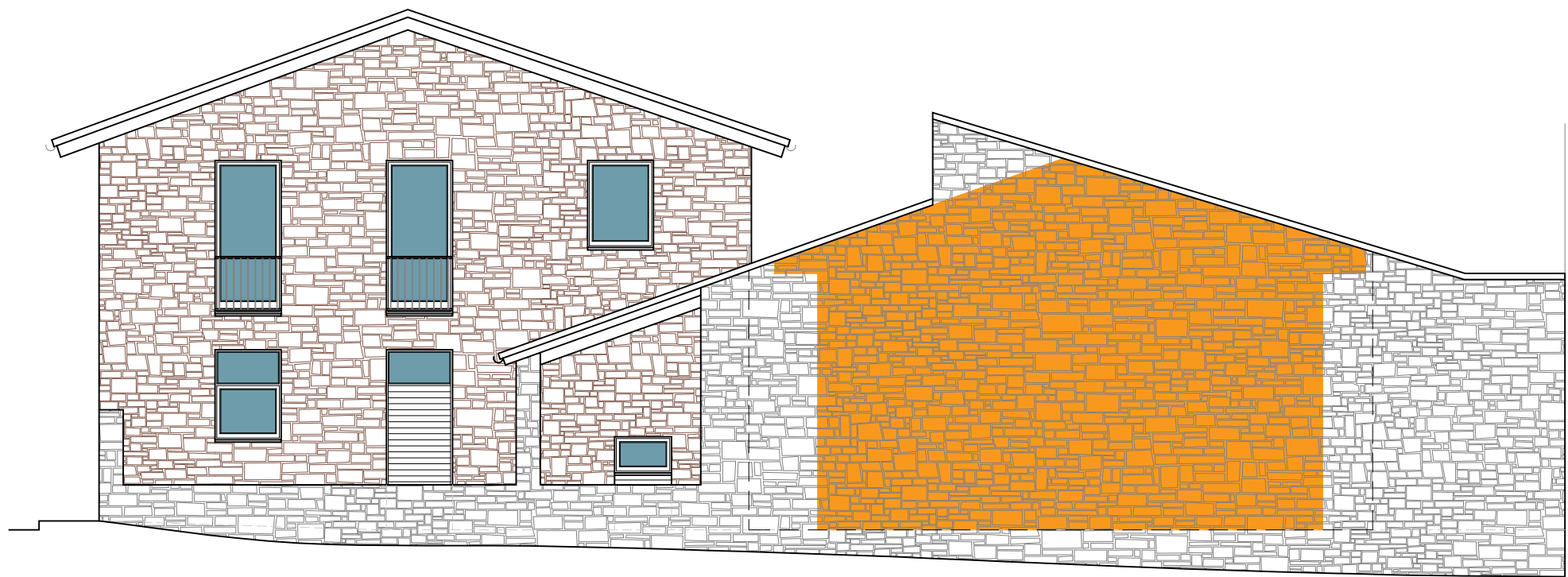
FAÇANA LATERAL
