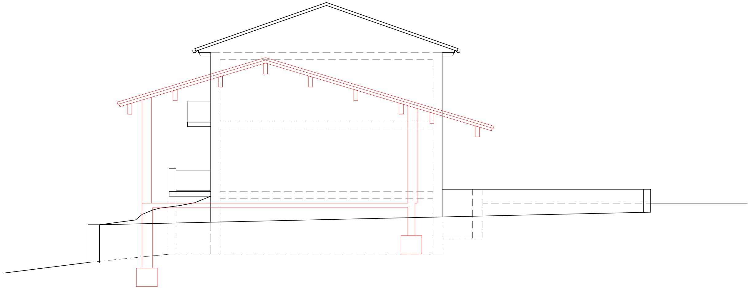
FAÇANA MITGERA VEÏNS
