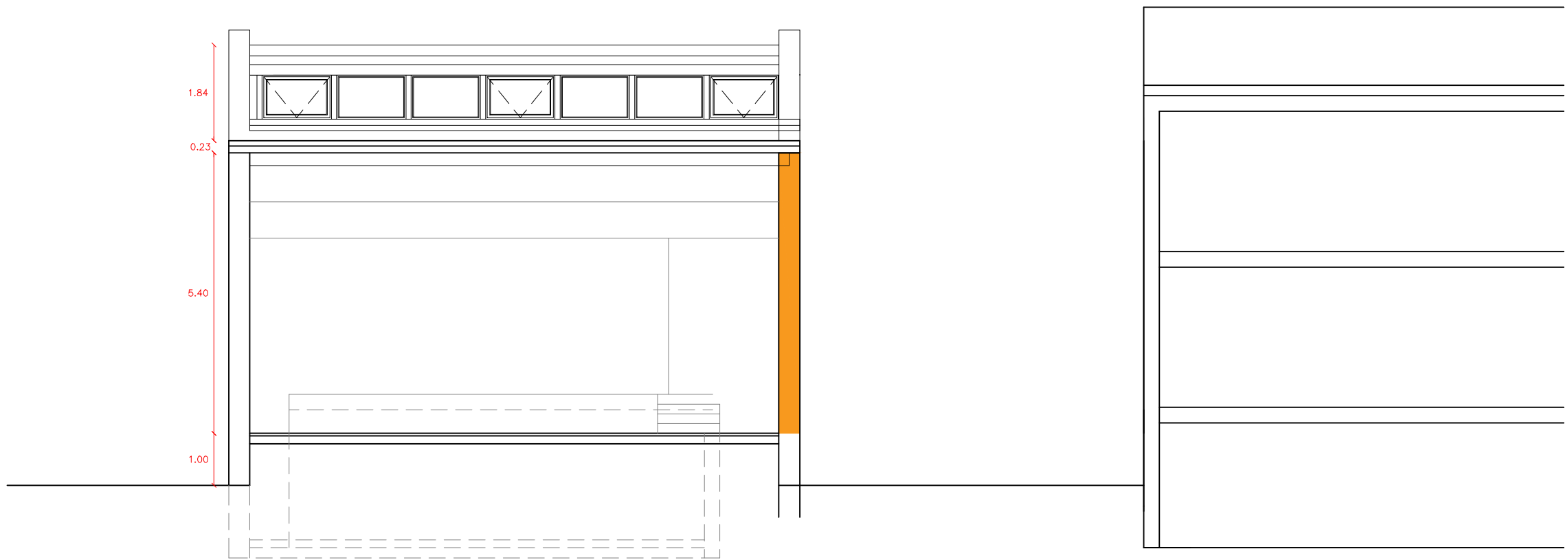
SECCIÓ TRANSVERSAL
