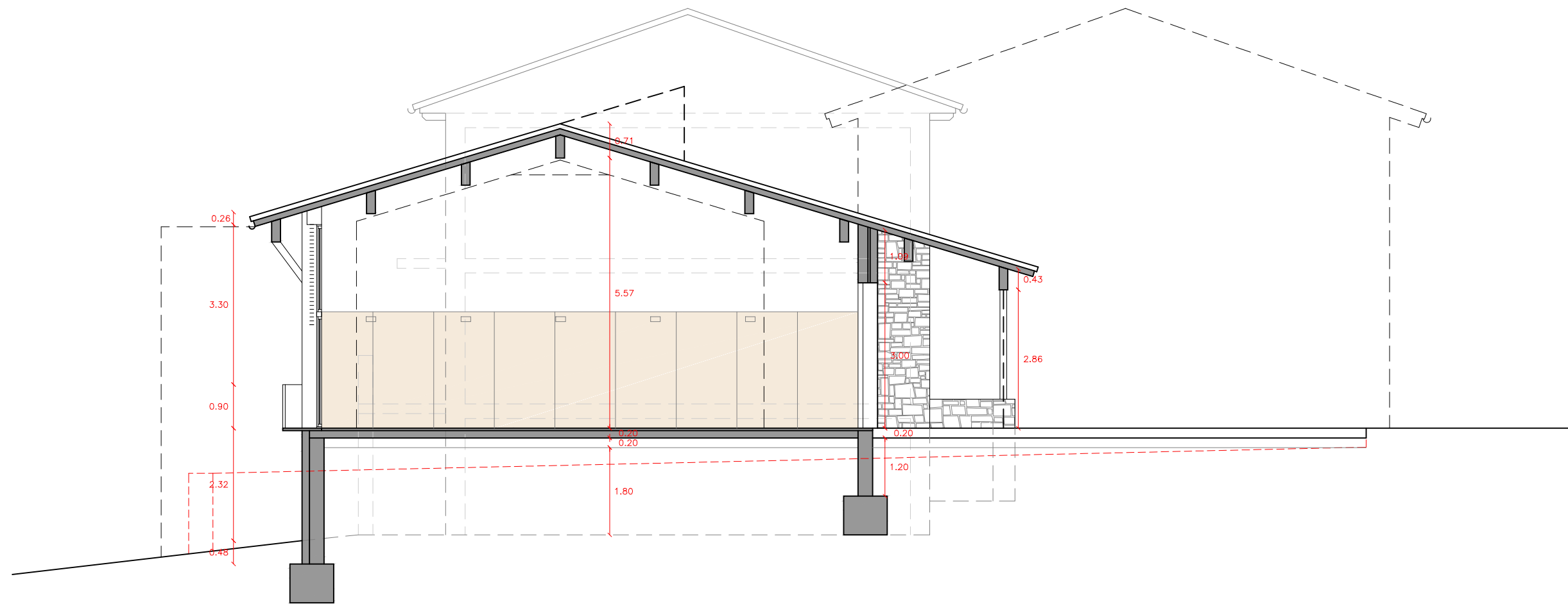
SECCIÓ LONGITUDINAL 1 - MITGERA
