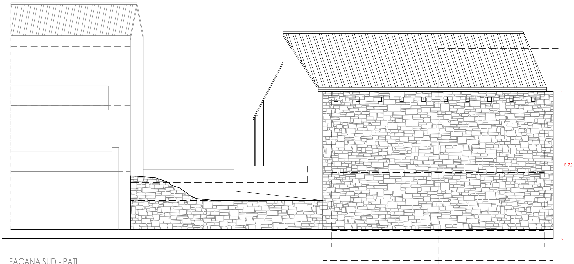
FAÇANA SUD - PATI
