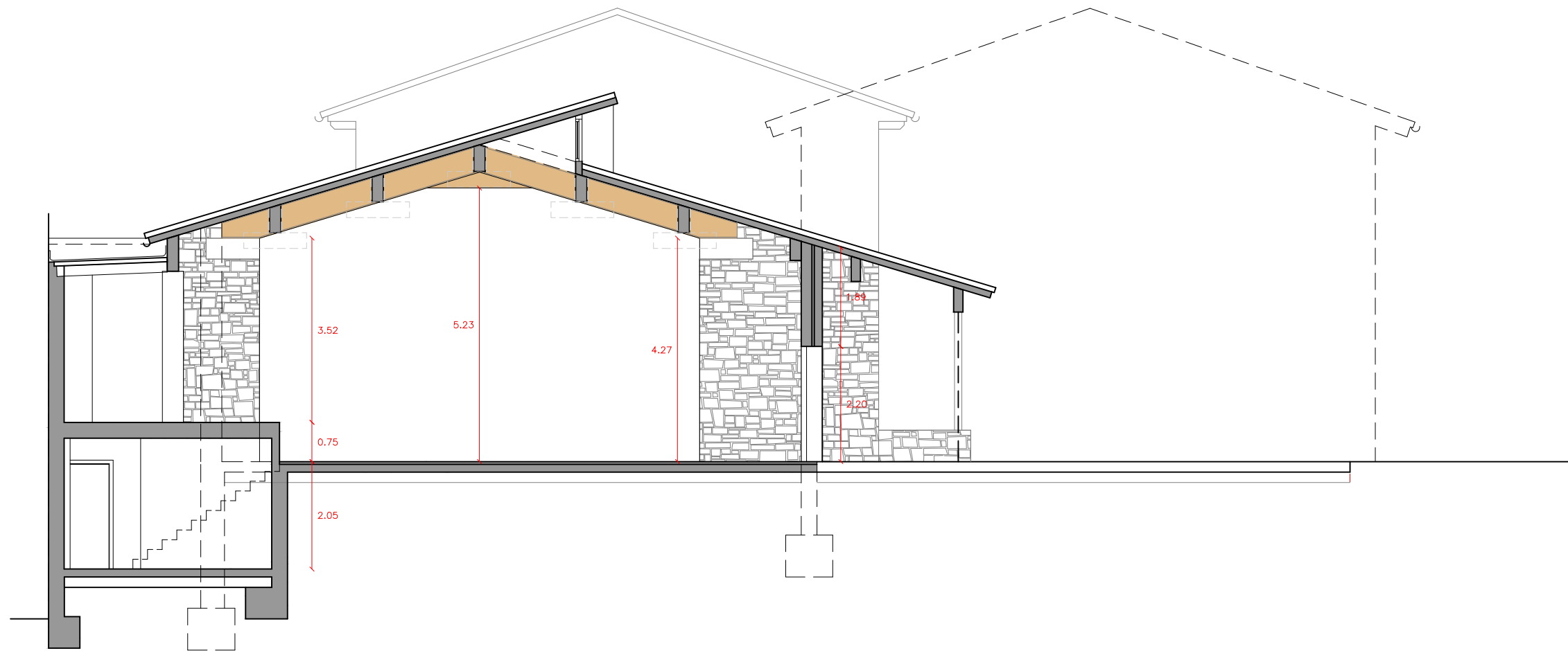
SECCIÓ LONGITUDINAL 2 - SALA EXISTENT
