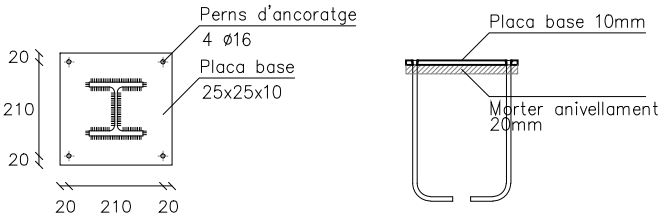
DETALL PILAR
