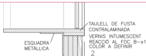
Detall 2 esc. 1/20
