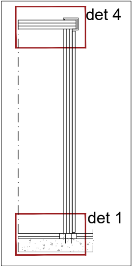
Secció 3 esc. 1/50
