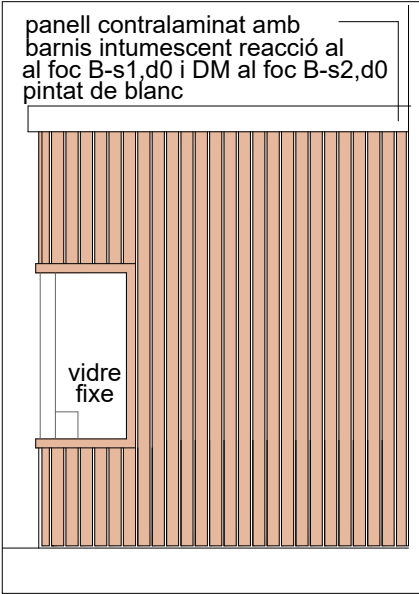
Alçat 2 esc. 1/50
