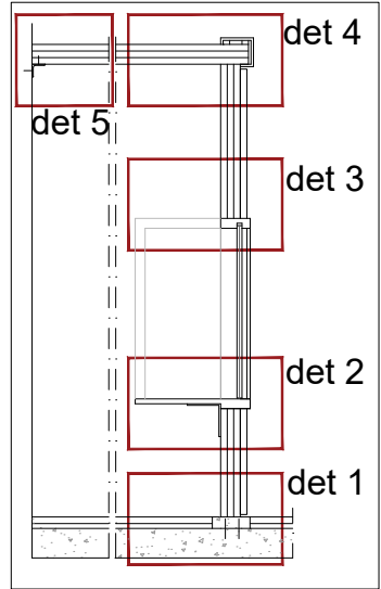
Secció 1 esc. 1/50
