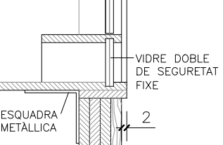
Detall 6 esc. 1/20
