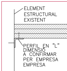
Detall 5 esc. 1/20
