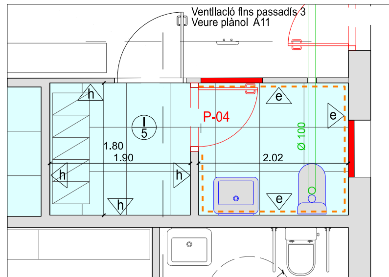
Planta proposta
