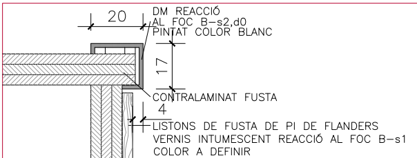
Detall 4 esc. 1/20
