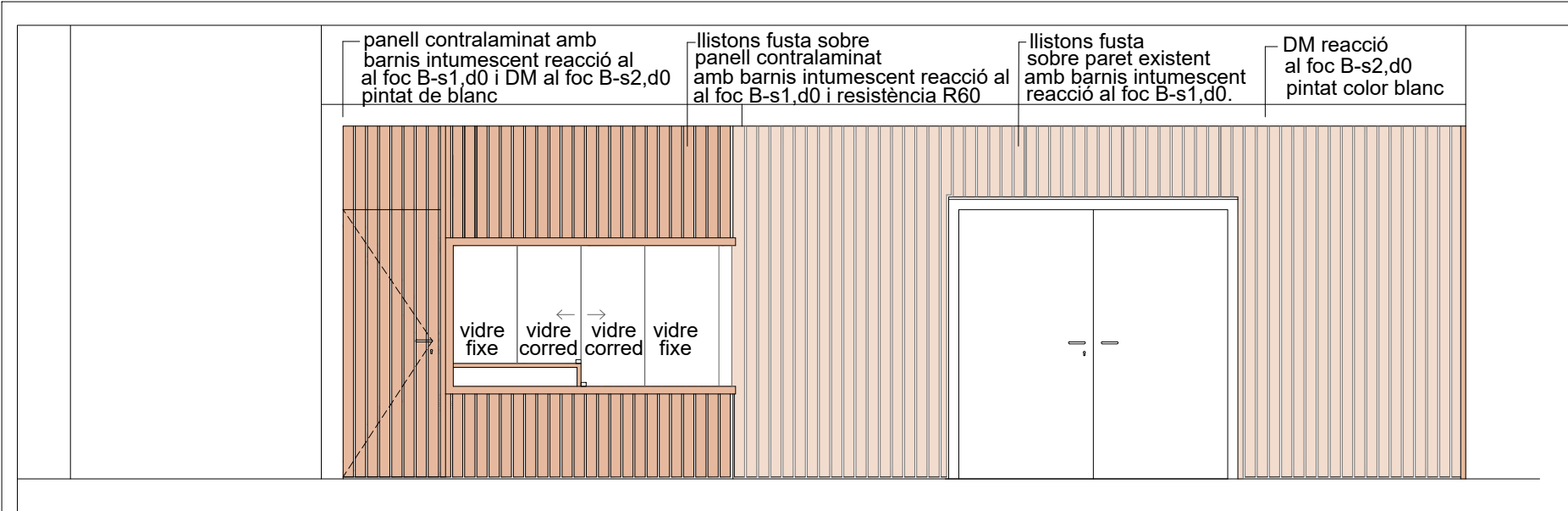
Alçat 1 esc. 1/50
