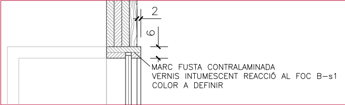
Detall 3 esc. 1/20
