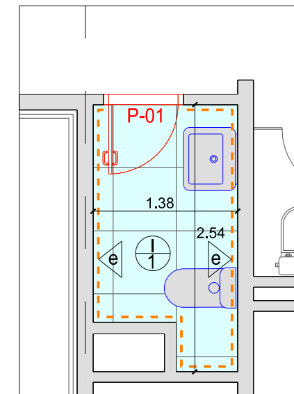
Planta proposta
