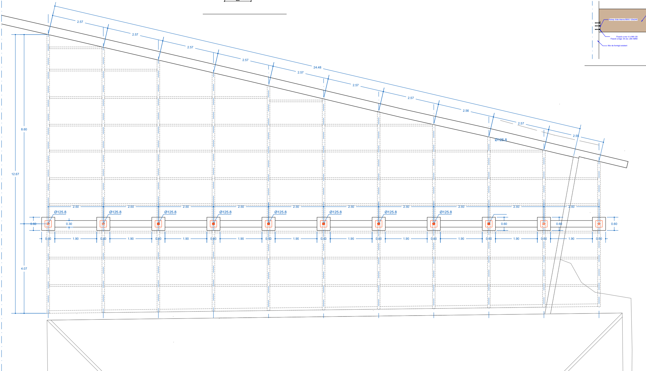
Sostre coberta
