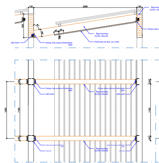
D.3 Detall secció coberta
