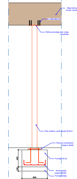
D.4 Detall sabata amb pilar metàl·lic
