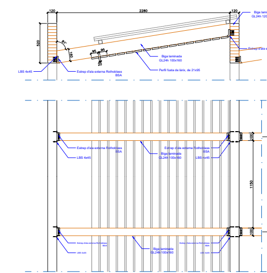
D.1 Detall secció coberta
