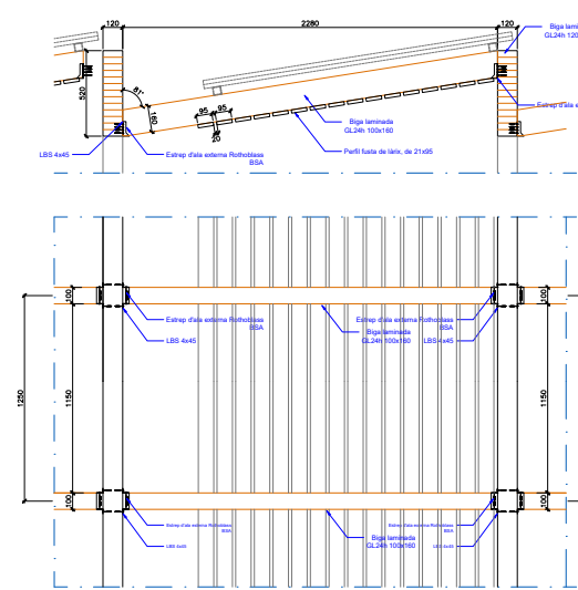
D.2 Detall secció coberta
