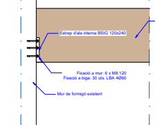
D.5 Detall entrega Jàssera-mur
