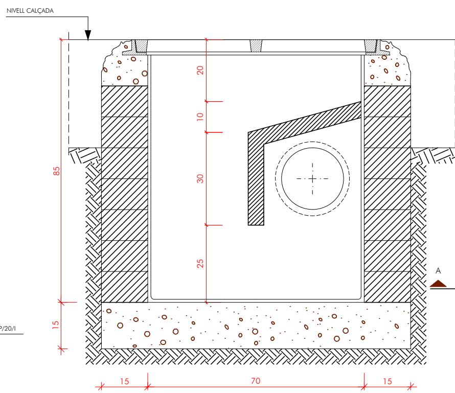
SECCIÓ C-C
