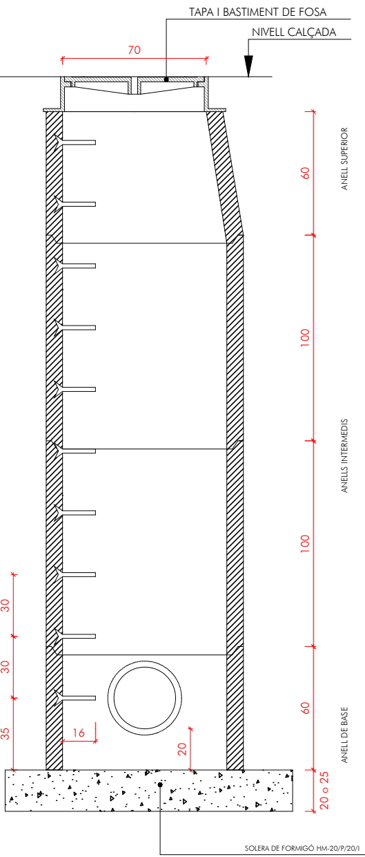
SECCIÓ A-A
