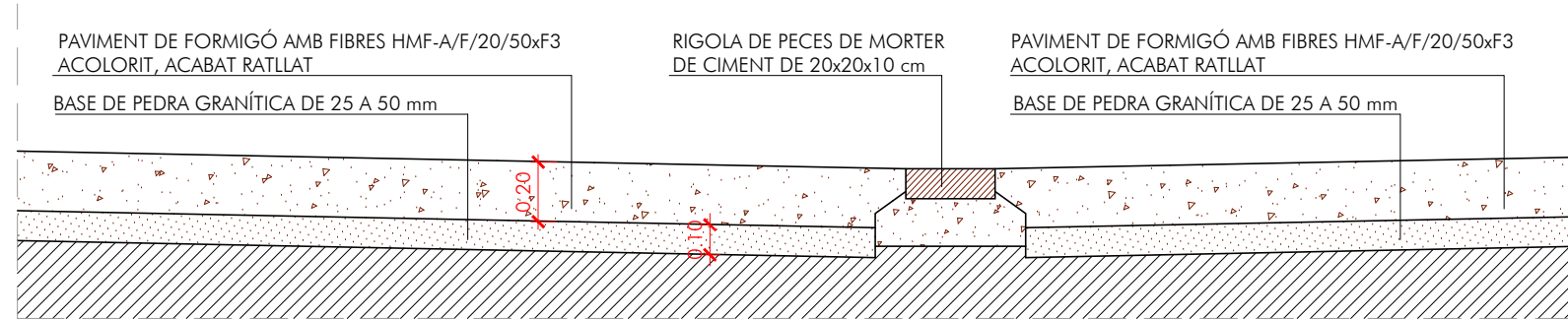
SECCIÓ 1. PAVIMENT DE FORMIGÓ ACOLORIT ESCALA 1/25
