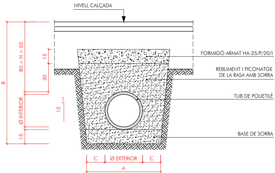
RASA TIPUS H > 50 i H < 80
