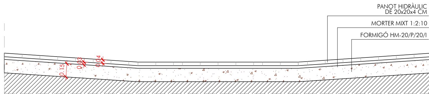
DETALL 2. SECCIÓ PAVIMENT DE PANOT HIDRÀULIC ESCALA 1/25
