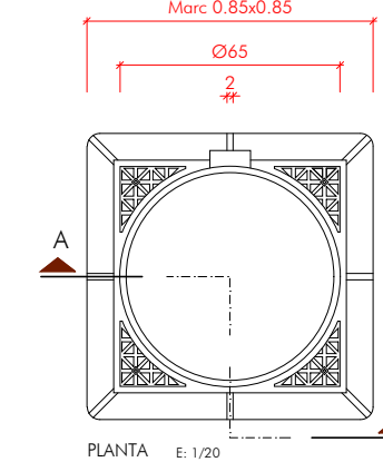
PLANTA E: 1/20
