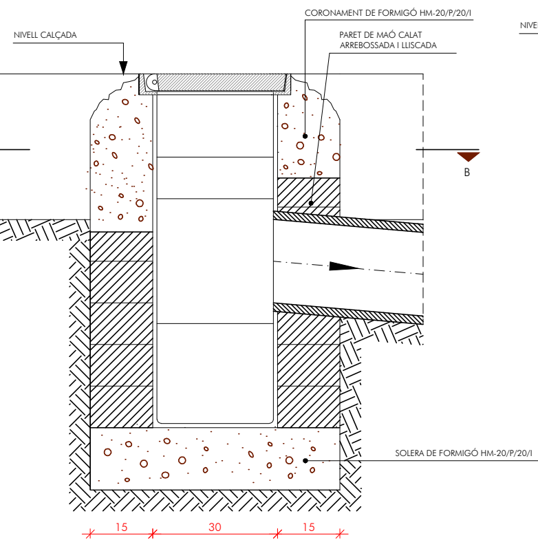
SECCIÓ A-A
