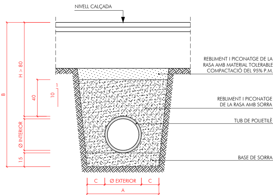
RASA TIPUS H > 80
