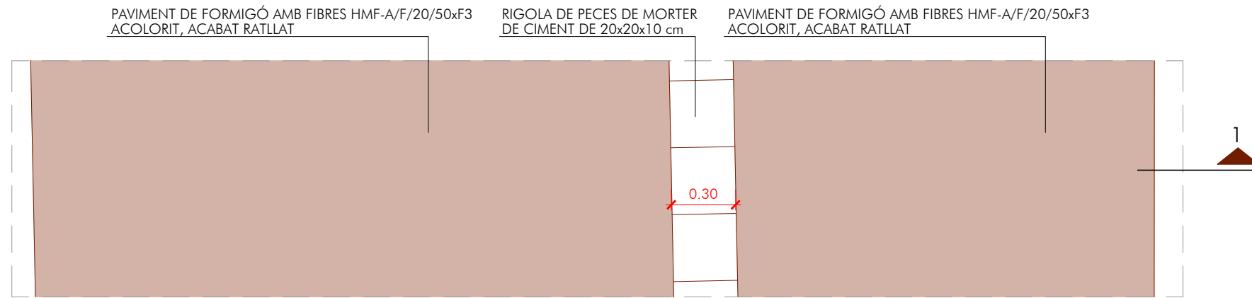
DETALL 1. PLANTA PAVIMENT DE FORMIGÓ ACOLORIT ESCALA 1/25
