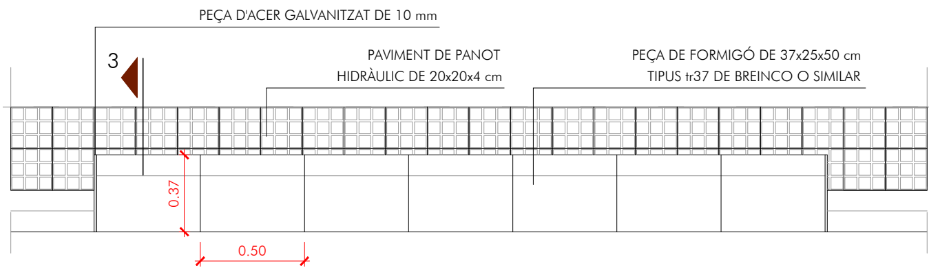
DETALL 3. REMUNTABLE ESCALA 1/25
