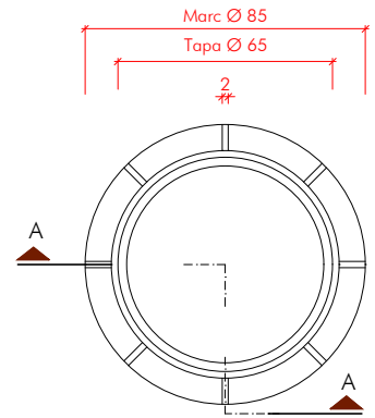
PLANTA E: 1/20
