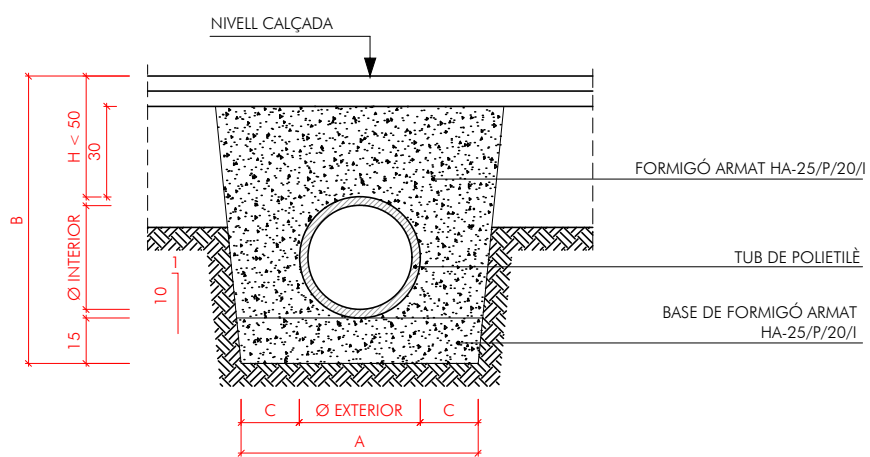
RASA TIPUS H < 50
