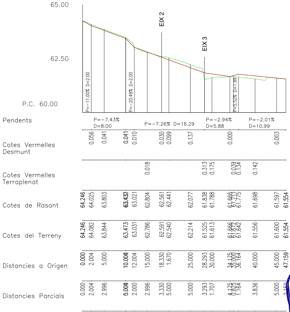
PERFIL LONGITUDINAL EIX 1
