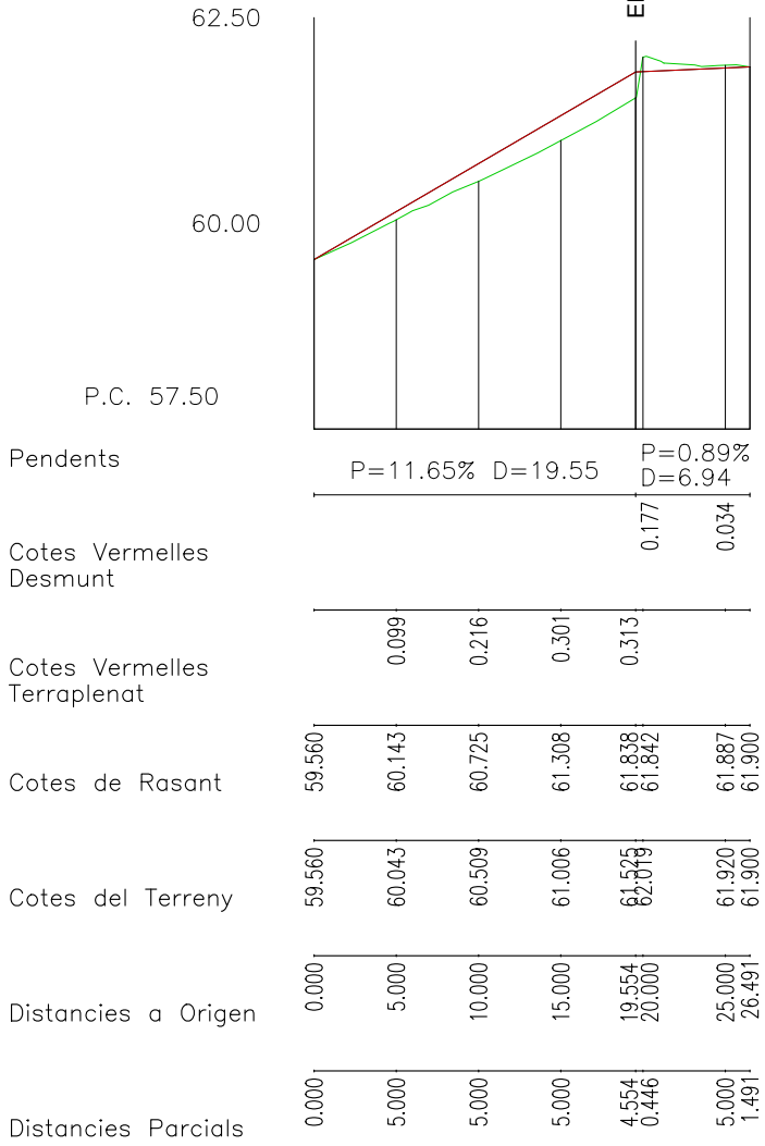
PERFIL LONGITUDINAL EIX 3
