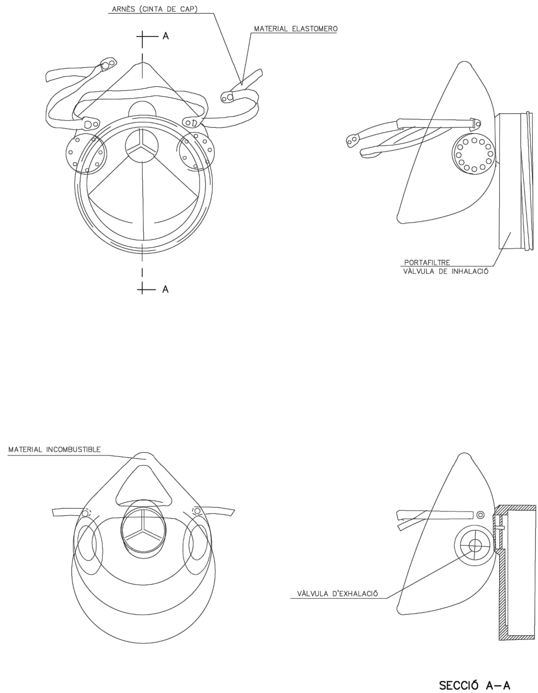
SECCIÓ A-A
