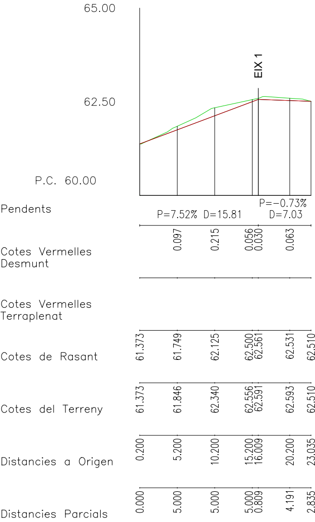
PERFIL LONGITUDINAL EIX 2
