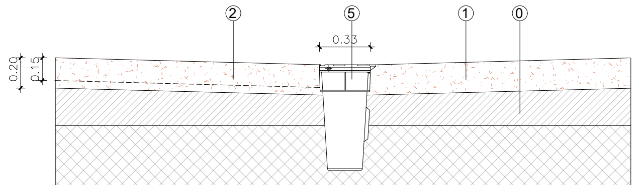
DETALL BB'
