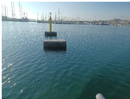
Fotografies 2. Estat actual piles antic moll benzinera
