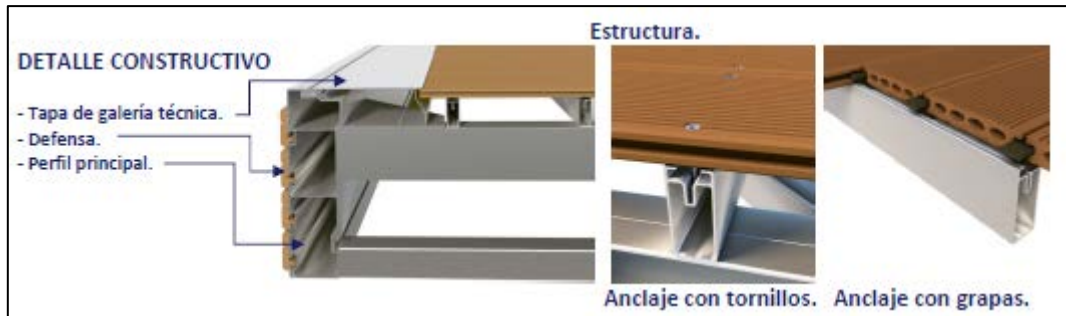
Imatge 2. Estructura i detall constructiu
