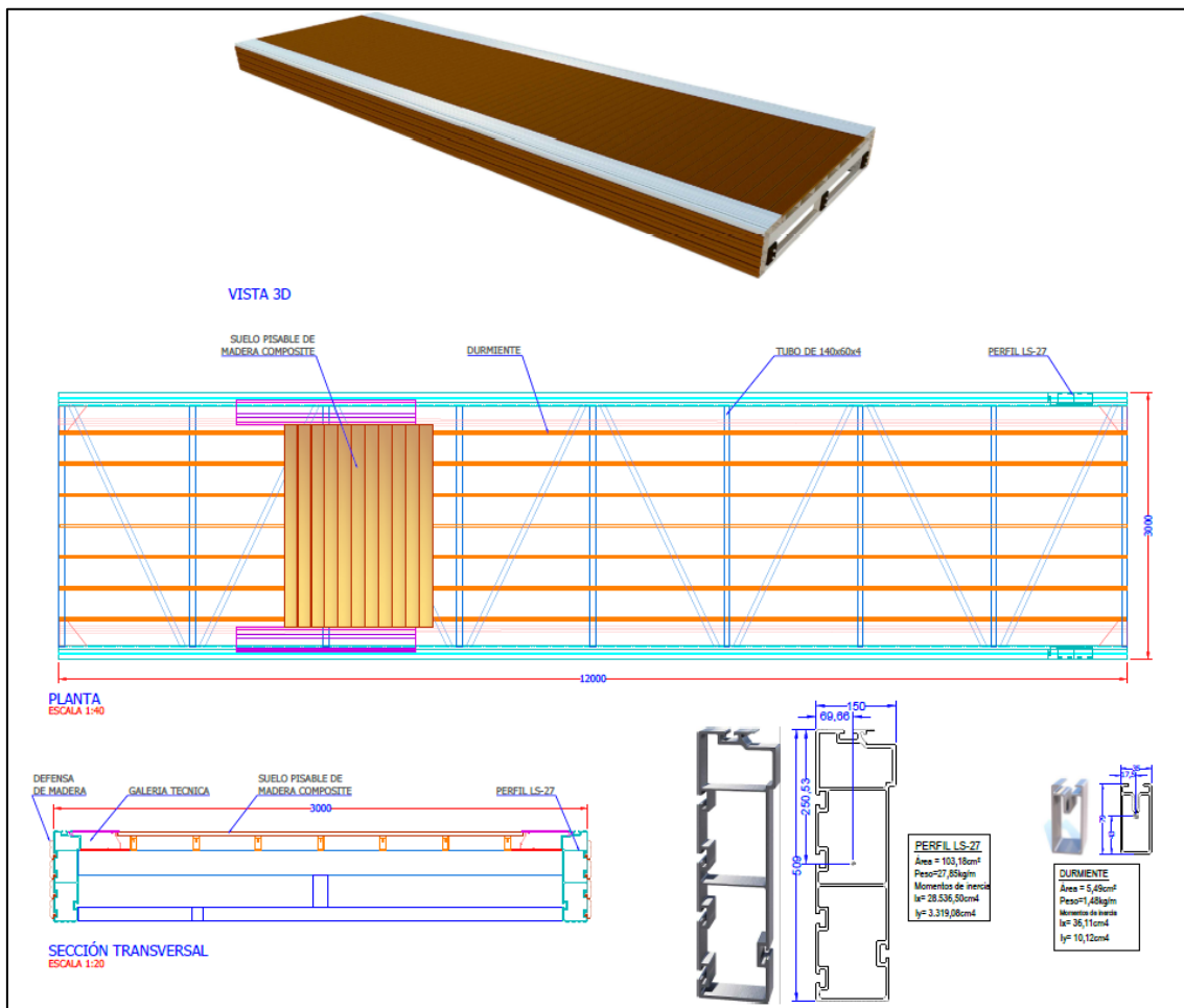
Imatge 3. Esquema tipus
