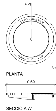
TAPA CIRCULAR REGISTRE ESCALA: 1/25
