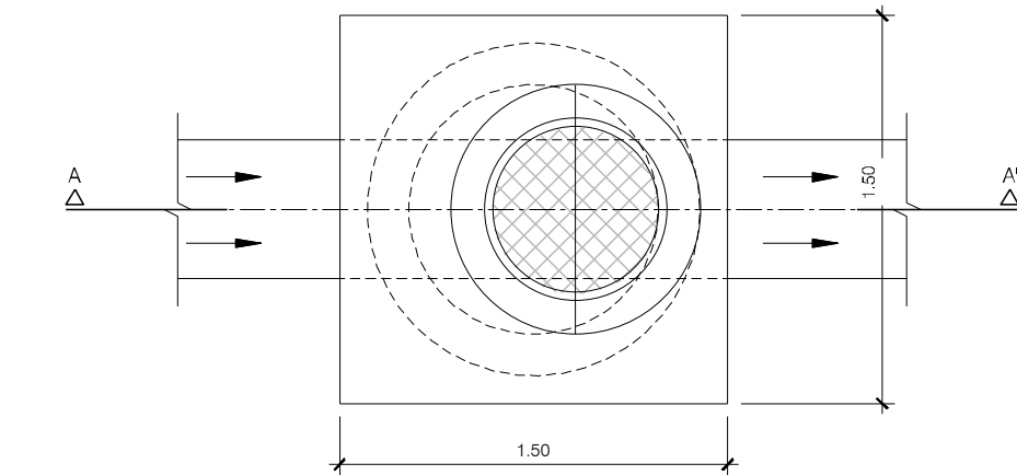
PLANTA POU DE REGISTRE PREFABRICAT SENSE SALTS ESCALA 1/20
