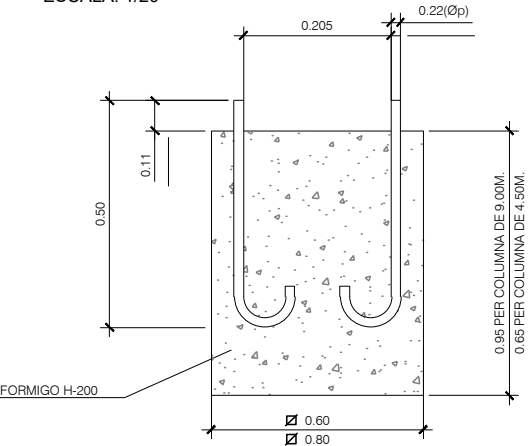
RASA FONAMENTACIÓ PER LLUMENERES EXISTENTS ESCALA: 1/20
