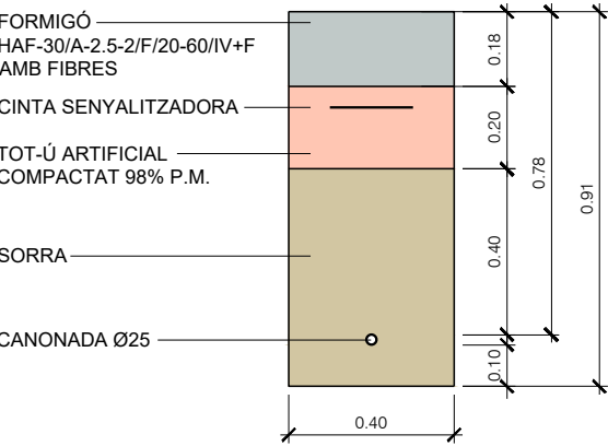
RASA TIPUS PER A CANONADA PE DN25 PN16 ESCALA: 1/20
