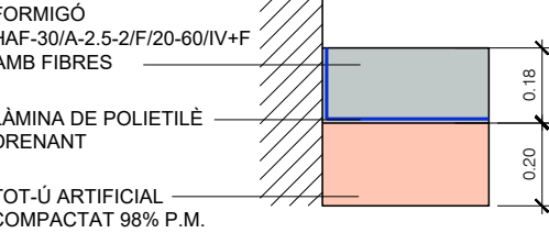
PAVIMENT FORMIGÓ AMB FIBRES I LÀMINA DRENANT ESCALA: 1/20
