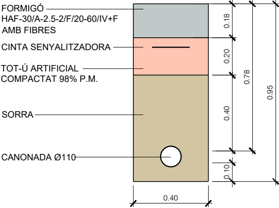
RASA TIPUS PER A CANONADA PE DN110 PN16 ESCALA: 1/20
