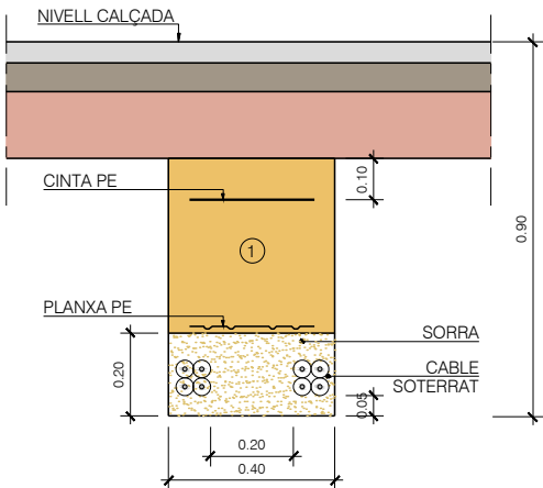
RASA BT AMB 2 CIRCUITS EN CALÇADA ESCALA 1/10
