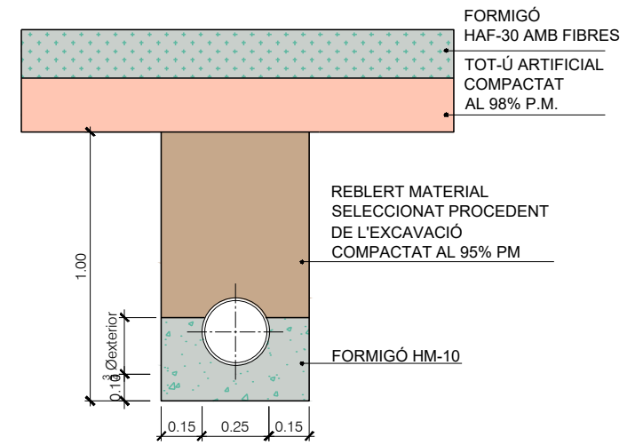
RASA TIPUS PER A COL·LECTOR PE ESTRUCTURAT DOBLE CAPA DN250 ESCALA: 1/25
