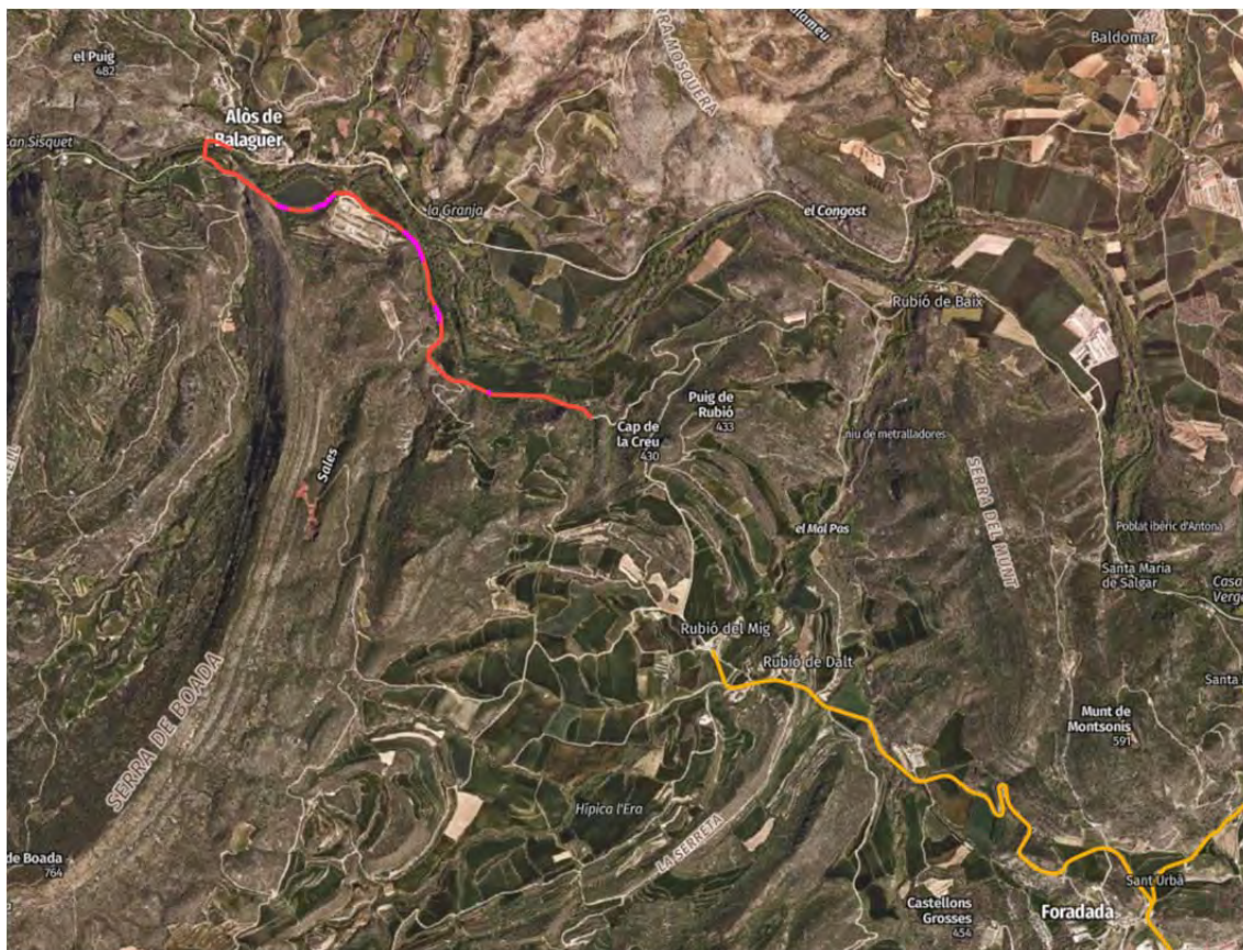
Ortofotomapa situació de la pista de Rubió a Alòs (vermell) en el TM d'Alòs (en groc Ctra Diputació accés a Rubió)
