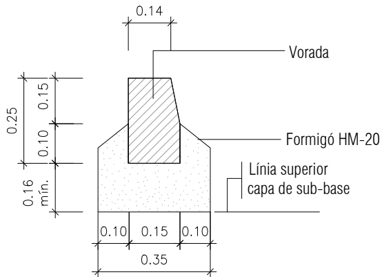
FERM PAVIMENT PANOT E:1/25
