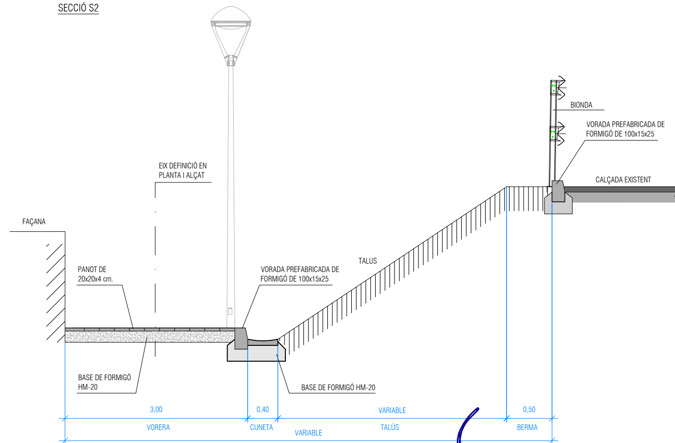
SECCIÓ S2
