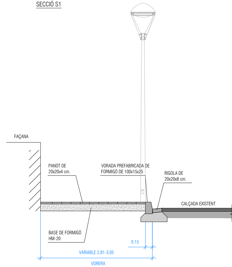
SECCIÓ S1
