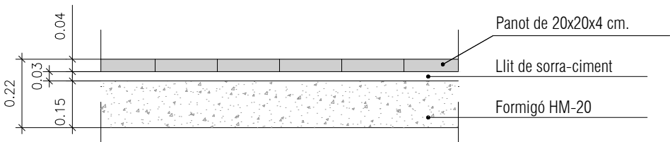
FERM PAVIMENT PANOT E:1/25
