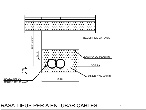
RASA TIPUS PER A ENTUBAR CABLES
