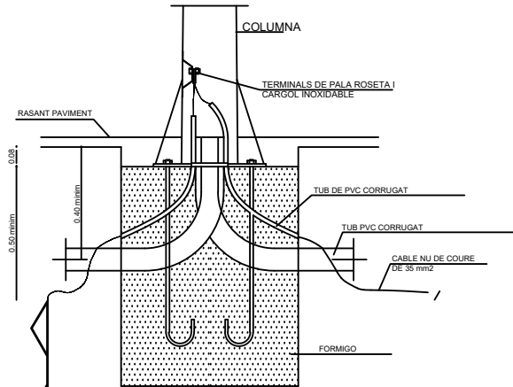
DETALL FONAMENT COLUMNA TIPUS I PRESA DE TERRA
