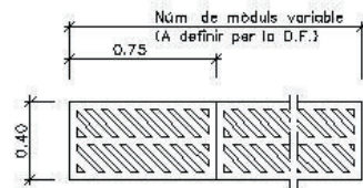
PLANTA REIXA
