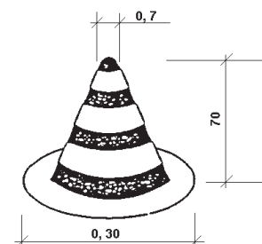
CONO BALIZAMIENTO
