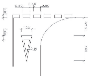
Esquema de marca i ratlla de cedir el pas
