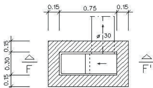
SECCIÓ F-F'
