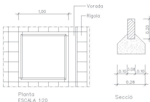
Escocell fiol prefabricat de formigó 100x100x20 (exterior)
