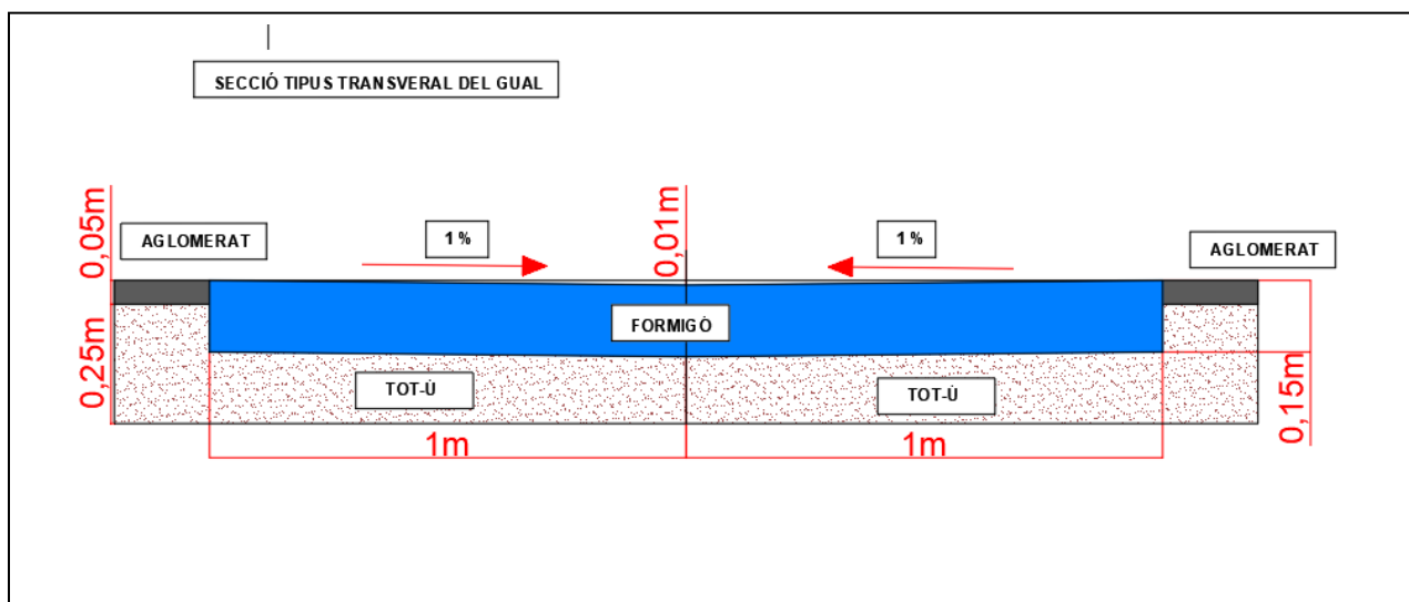
Imatge 19: Secció tipus transversal dels guals
