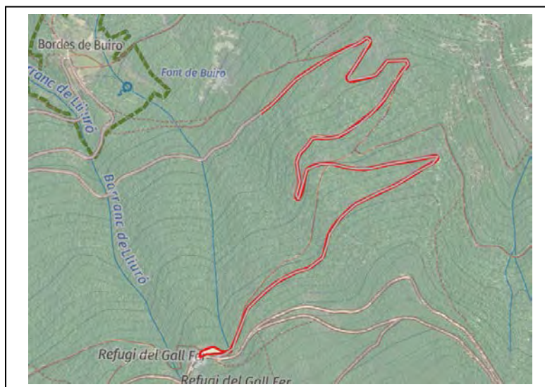
Imatge 8: Barranc zona de l'obra
