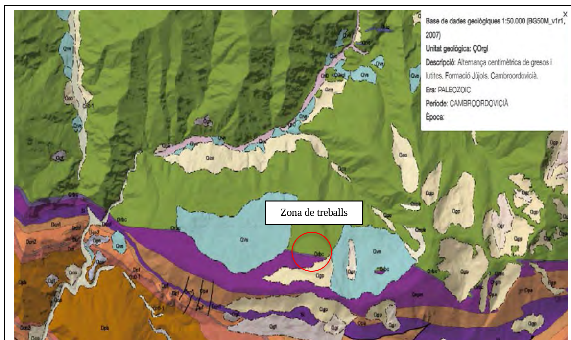
Imatge 5: Geologia de l'àmbit d'estudi i el seu entorn (Font: Institut Cartogràfic i Geològic de Catalunya).
