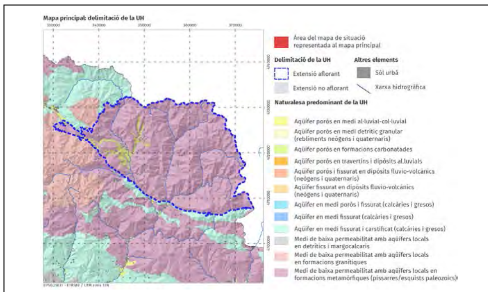
Imatge 7: Hidrologia de la zona de l'obra
