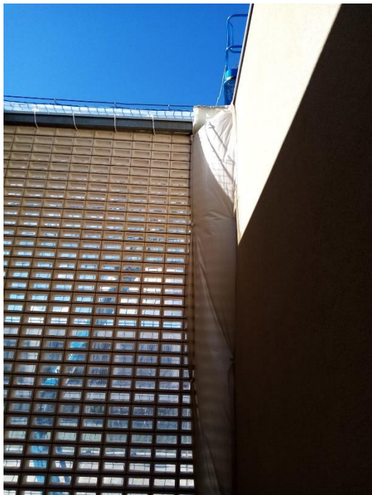
Detall protecció trobada gelosia-façana pati interior Vista junt dilatació i bombament façana
