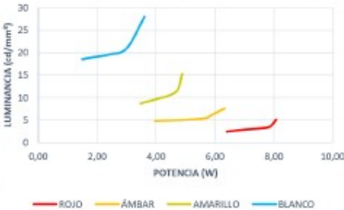
Curvas de percepción (Conductor de vehículo a 30m)
