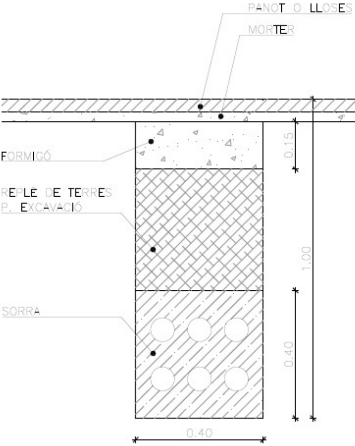
RASA TIPUS 2 E:1/20
