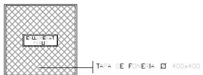
TRONETA REGISTRE D'ENLLUMENAT E:1/20
