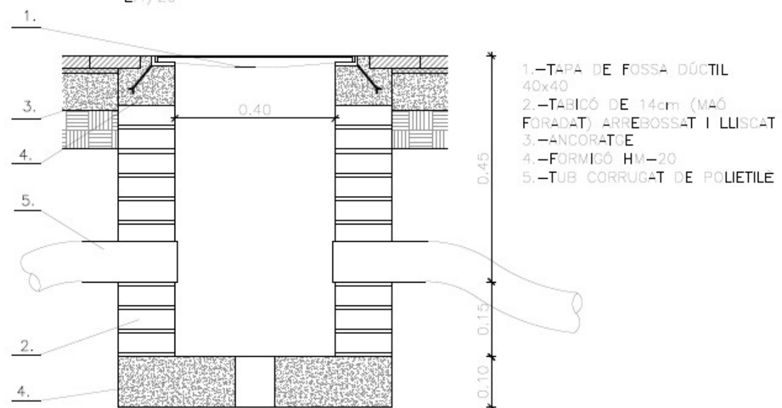
TRONETA REGISTRE D'ENLLUMENAT E:1/20
