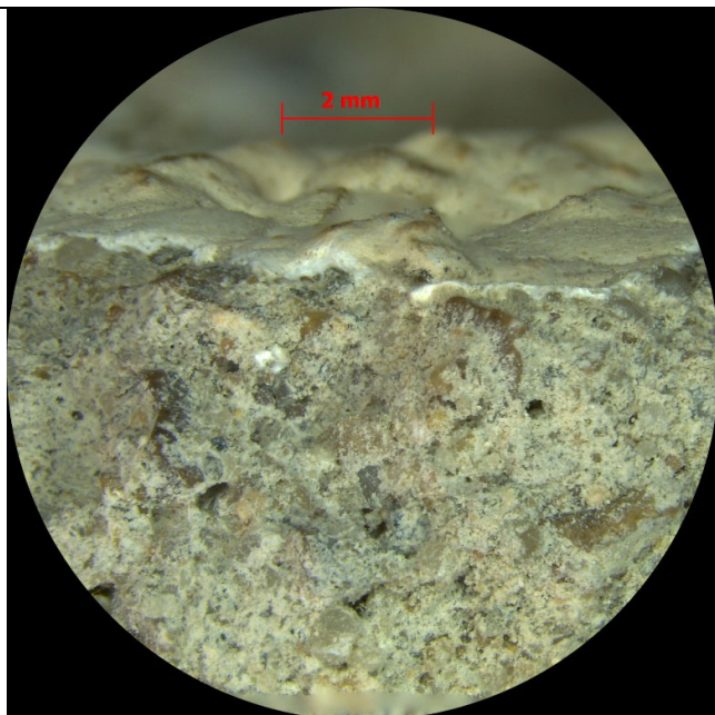
Micrografia 1: Parament reculat façana principal àtic: Morter de ciment amb un acabat repintat i texturat.
