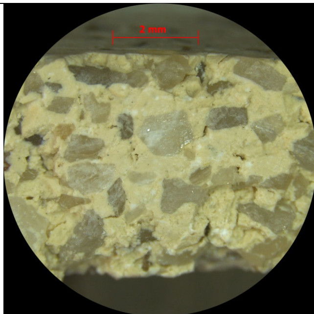
Micrografia 2: Parament general façana principal: Estuc de calç pigmentat en massa del Color A.
