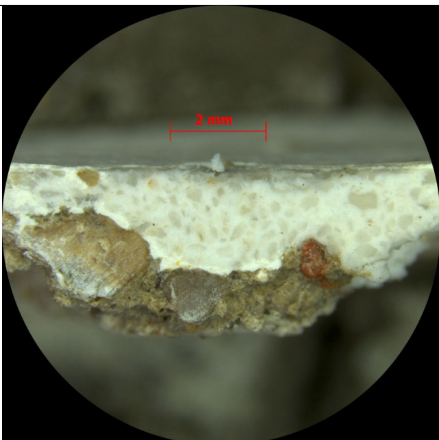
Micrografia 3: Parament façana posterior a àtic: Estuc de calç preconfecionat.
