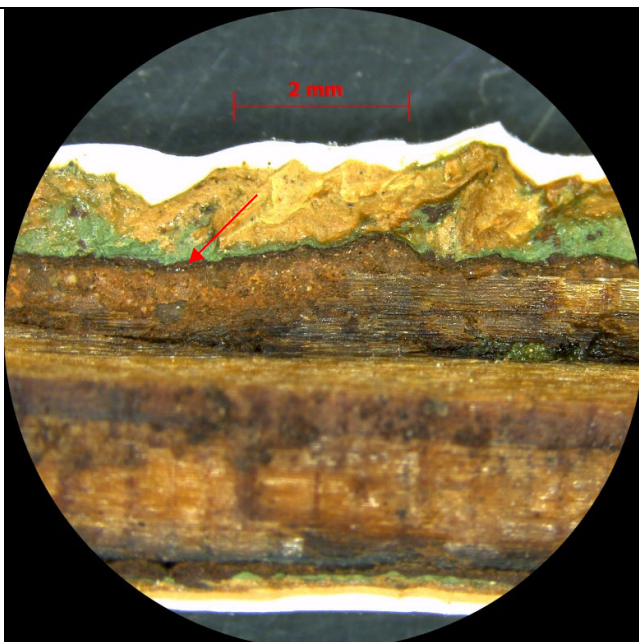
Micrografia 4: Fusteria: Secció d'una de les finestres històriques.
