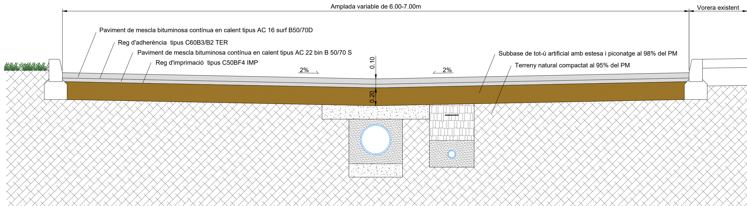
SECCIÓ TRANSVERSAL VIAL (E 1:25)
