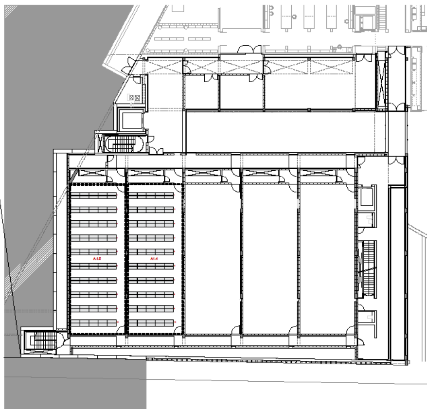
Planta Primera - Dipòsit A.1.4 + A.1.5 E 1/250
