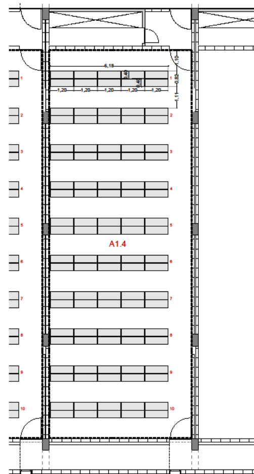
Planta Primera - Detall Prestatgeries E 1/100
