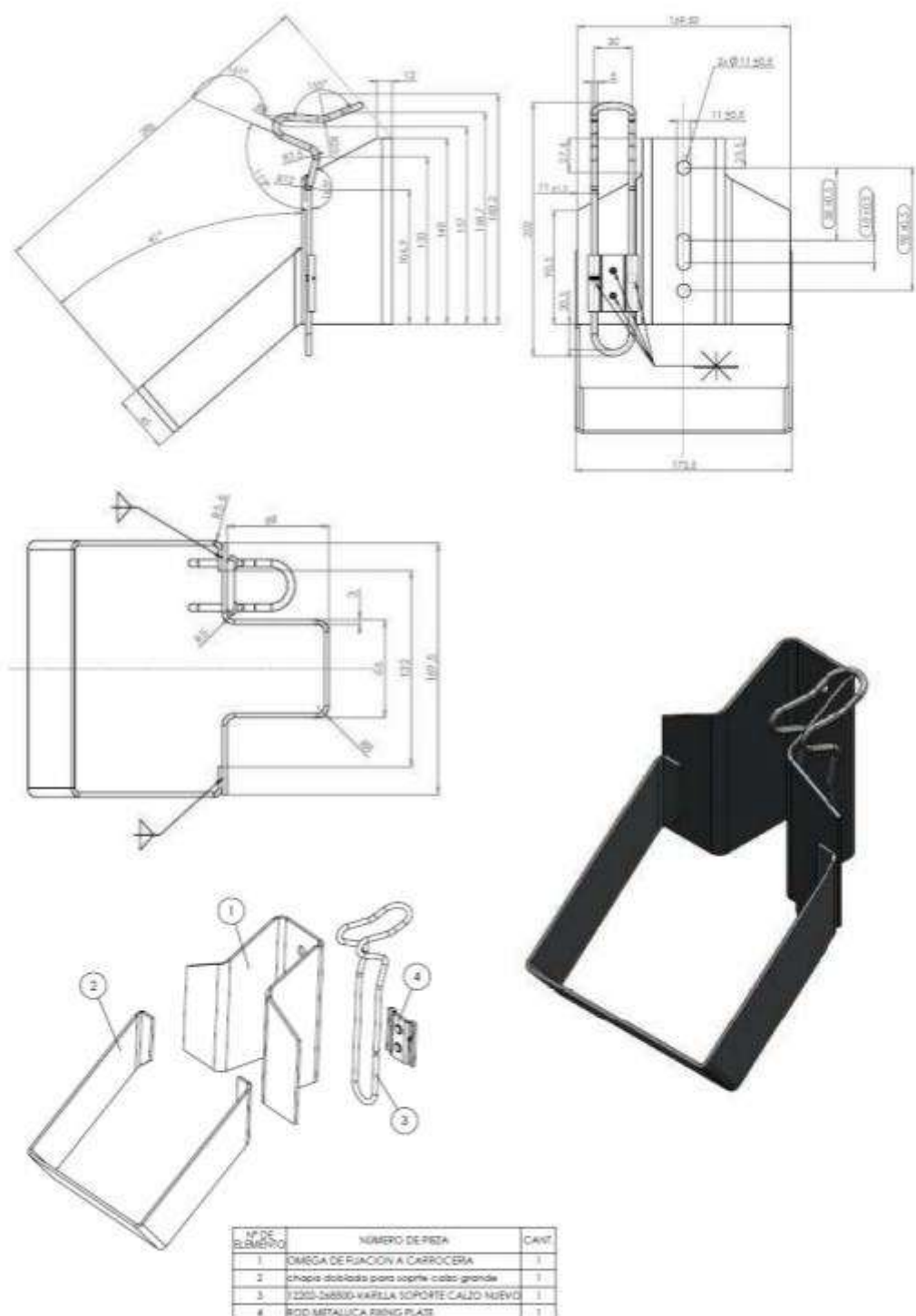
Figura 5. Soporte calzo
