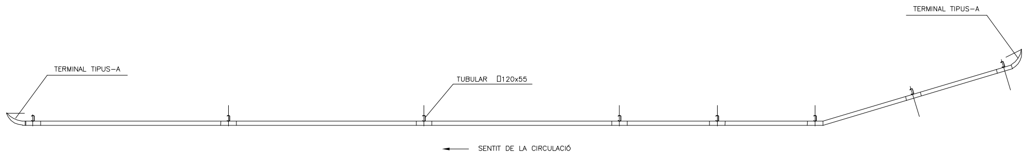
ALÇAT TERMINAL TIPUS-A DETALL D'INSTAL·LACIÓ I ANCORATGE ESCALA: 1/50
