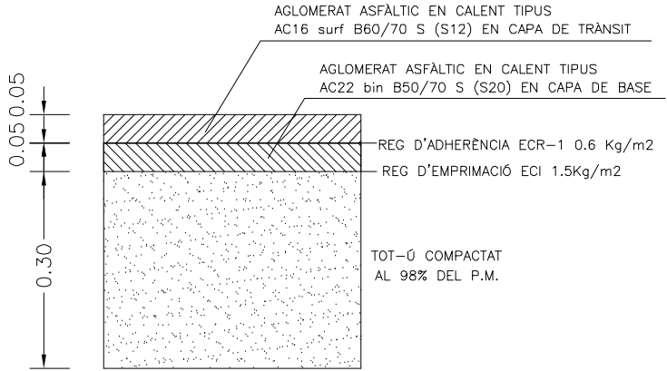
DETALL REPARACIÓ FLONJALLS I ARRELS
