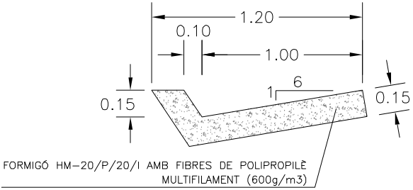
DETALL CUNETA REVESTIDA TTR-10
