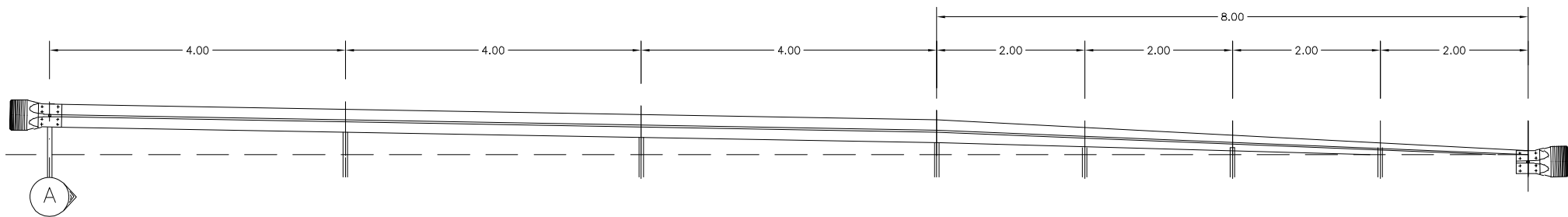
ALÇAT TERMINAL TIPUS-A DETALL D'INSTAL·LACIÓ I ANCORATGE ESCALA: 1/50
