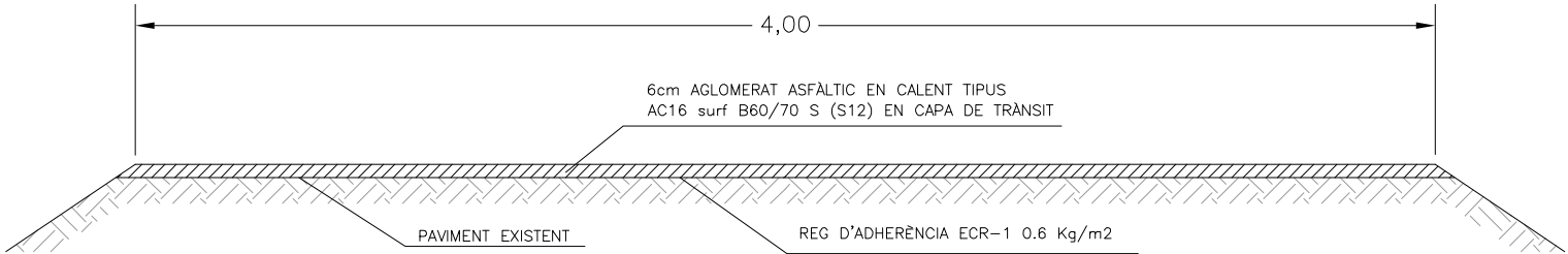
SECCIÓ TIPUS ZONA REFORÇ DEL FERM TRANS DE PAVIMENT ASFÀLTIC
