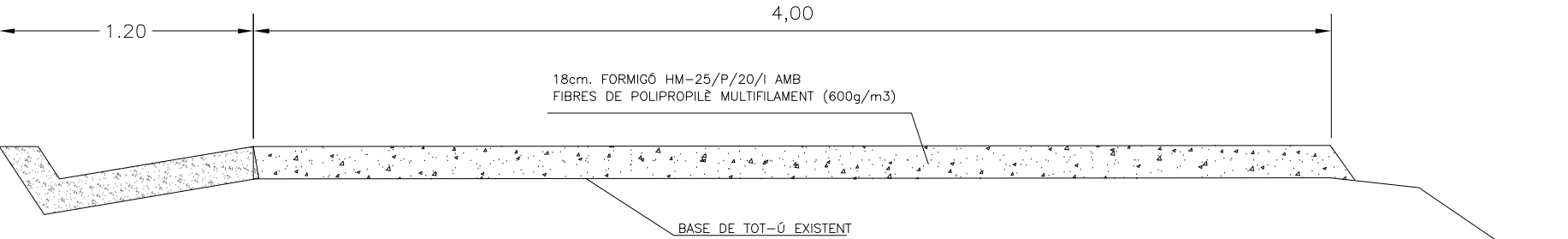
SECCIÓ TIPUS TRANS DE PAVIMENT DE FORMIGÓ
