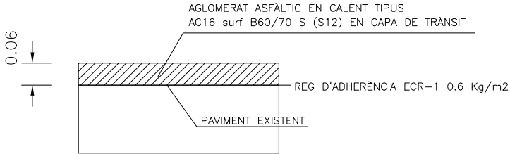
DETALL REFORÇ DEL FERM
