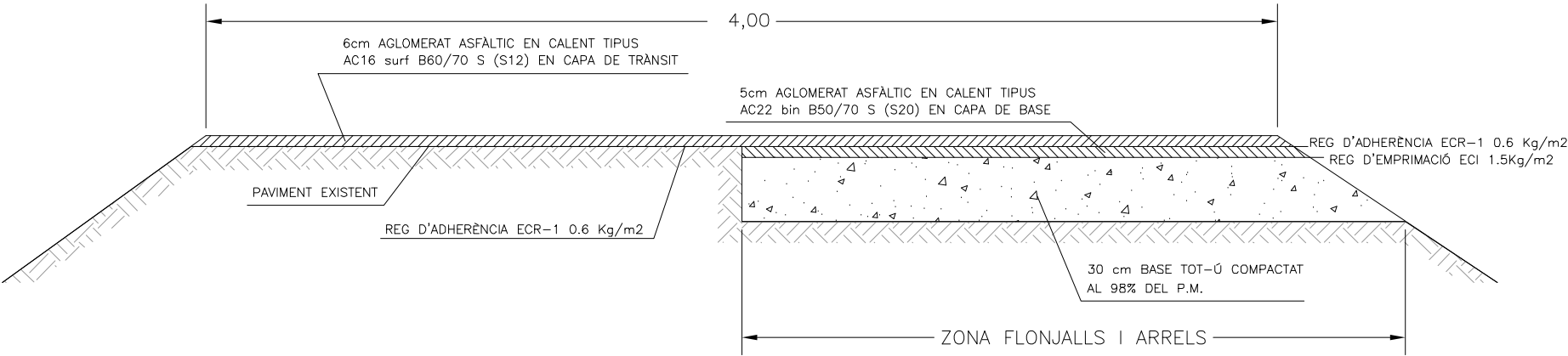
SECCIÓ TIPUS ZONA FLONJALLS I ARRELS
