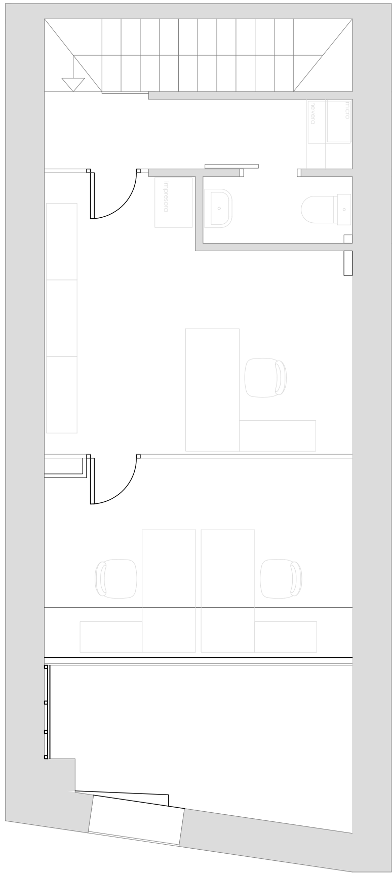
PLANTA ALTELL
