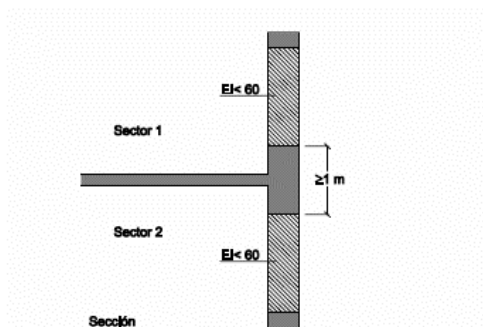
Figura 1.7 Encuentro forjado-fachada
