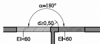
Figura 1.6. Fachadas a 180°
