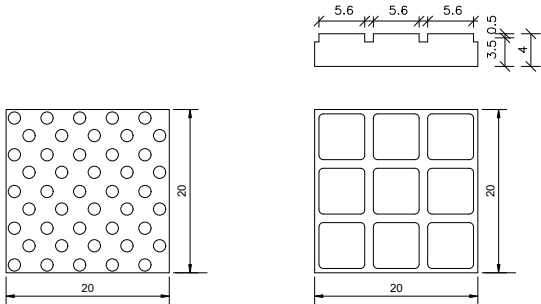
PANOT BOTONERA ANTILLISCANT (TACS COLOR VERMELL)
