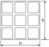
PANOT TIPUS 9 PASTILLES (20 x 20 x 4)
