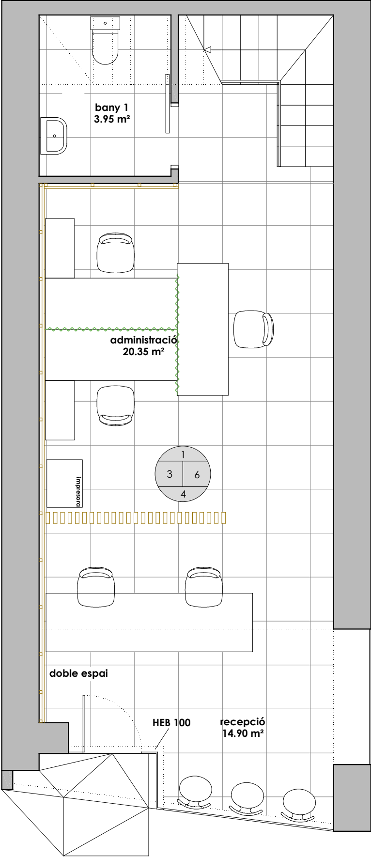
PLANTA BAIXA
