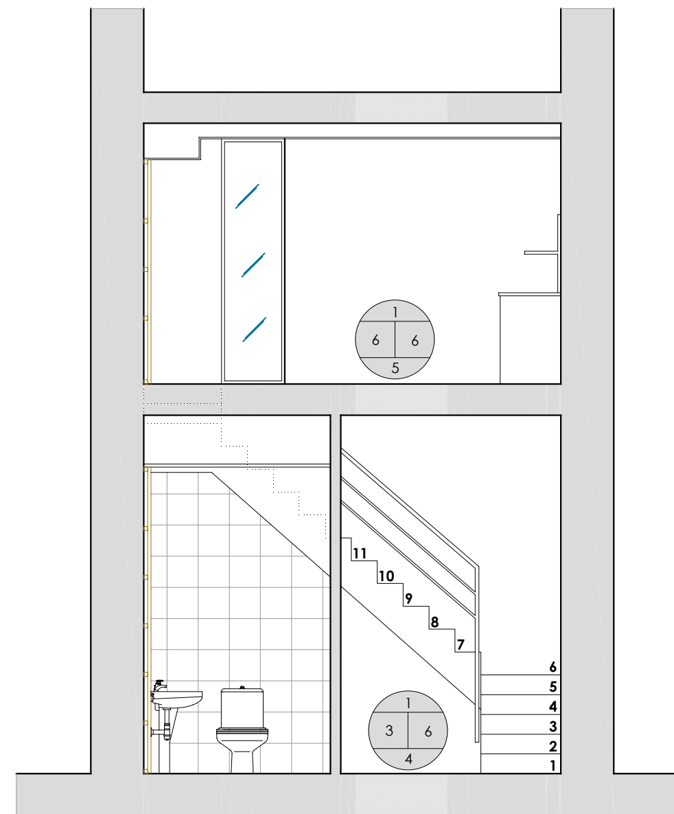
SECCIÓ TRANSVERSAL
