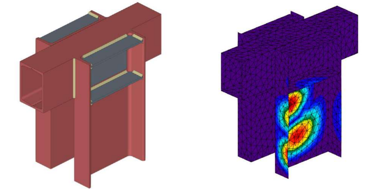
Figura 1.5.4.2. Geometria i tensions de Von Mises en un dels models d'unió analitzats amb CYPE CONNECT
