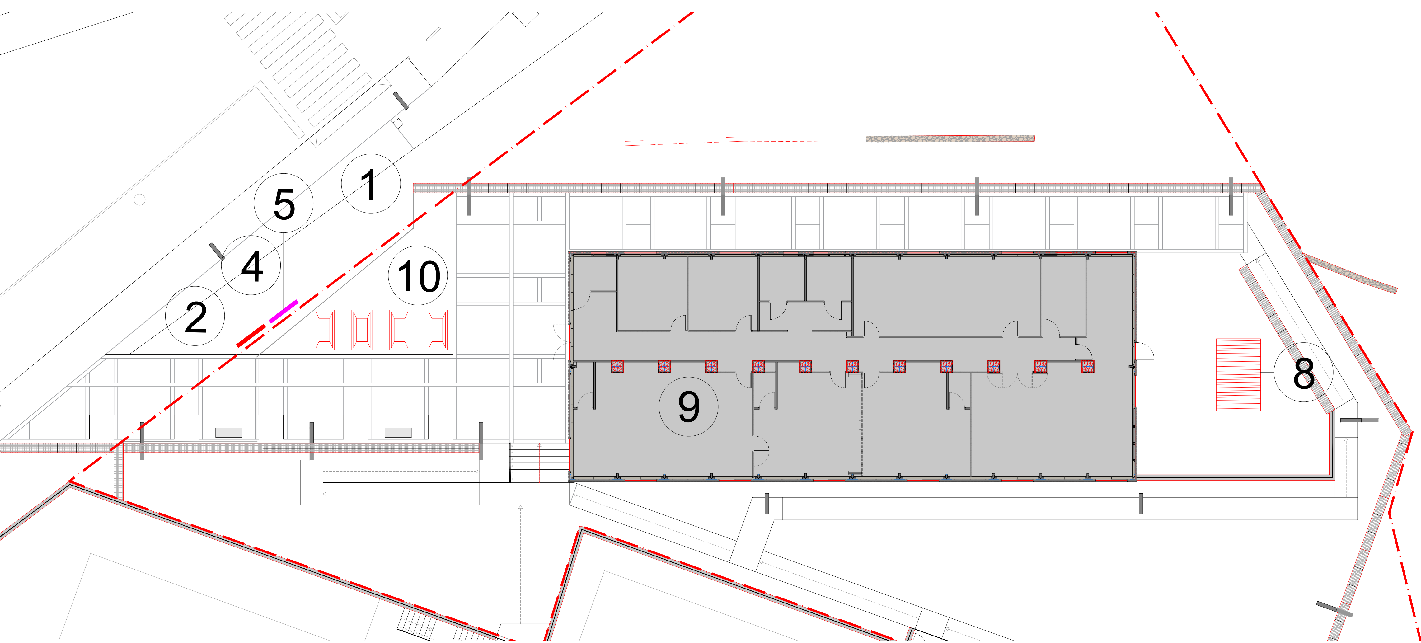
PLANTA BAIXA
