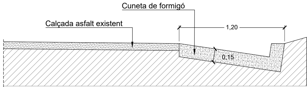
Secció tipus cuneta remountable V
