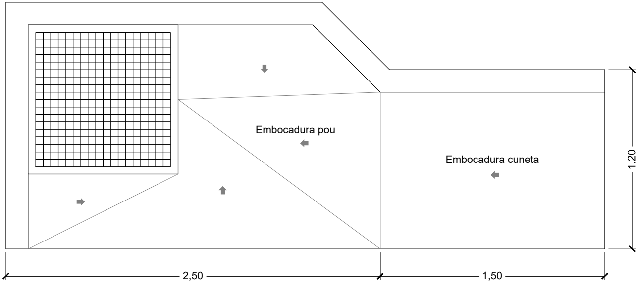
Planta tipus - embocadura de pou
