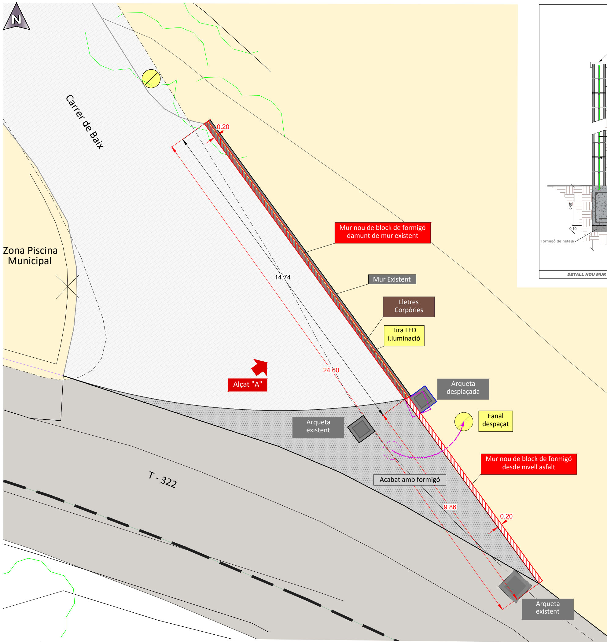
Planta e.1/100
