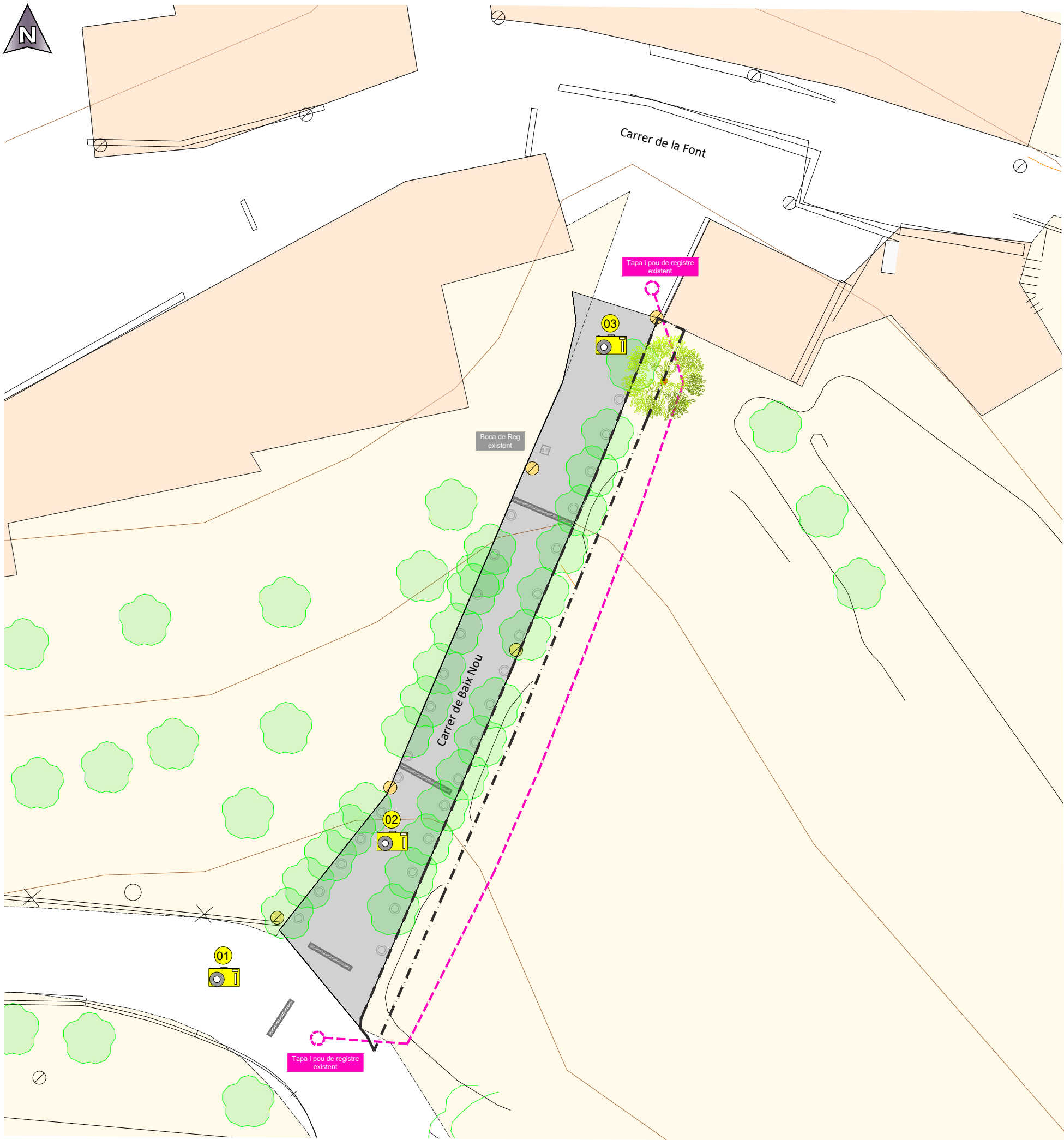
Planta e.1/100
