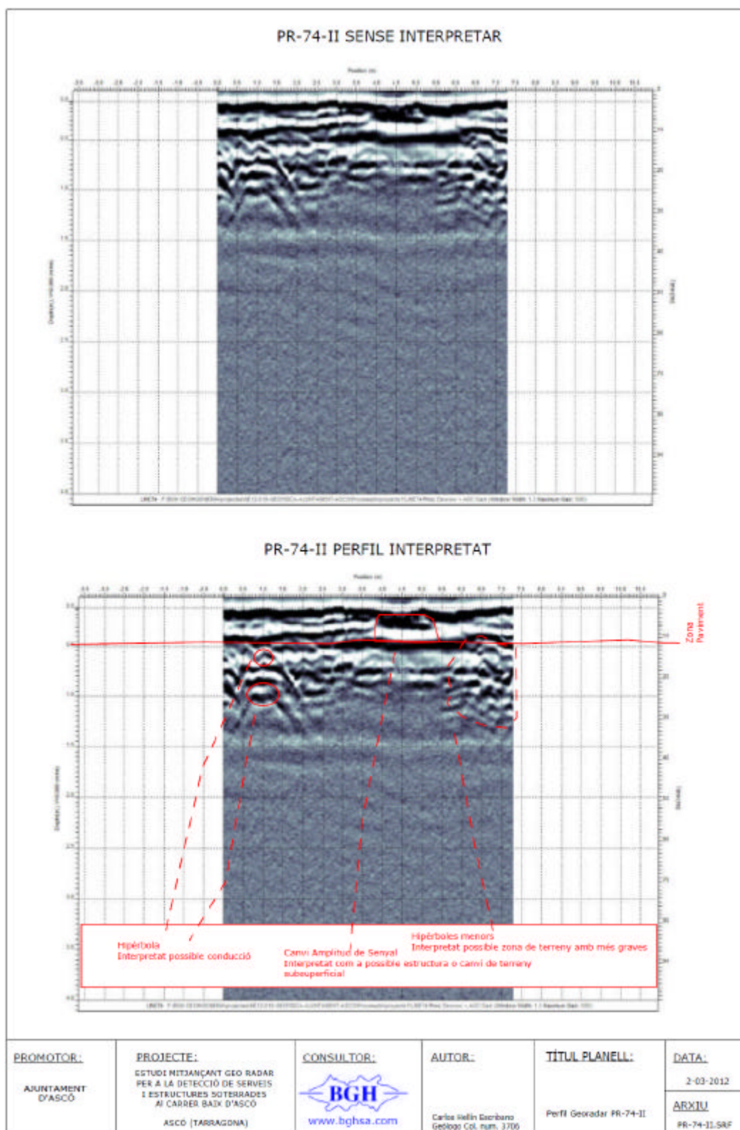
Figura 60. PR-74-II PERFIL GEORADAR. Transversal a Carrer de Baix.
