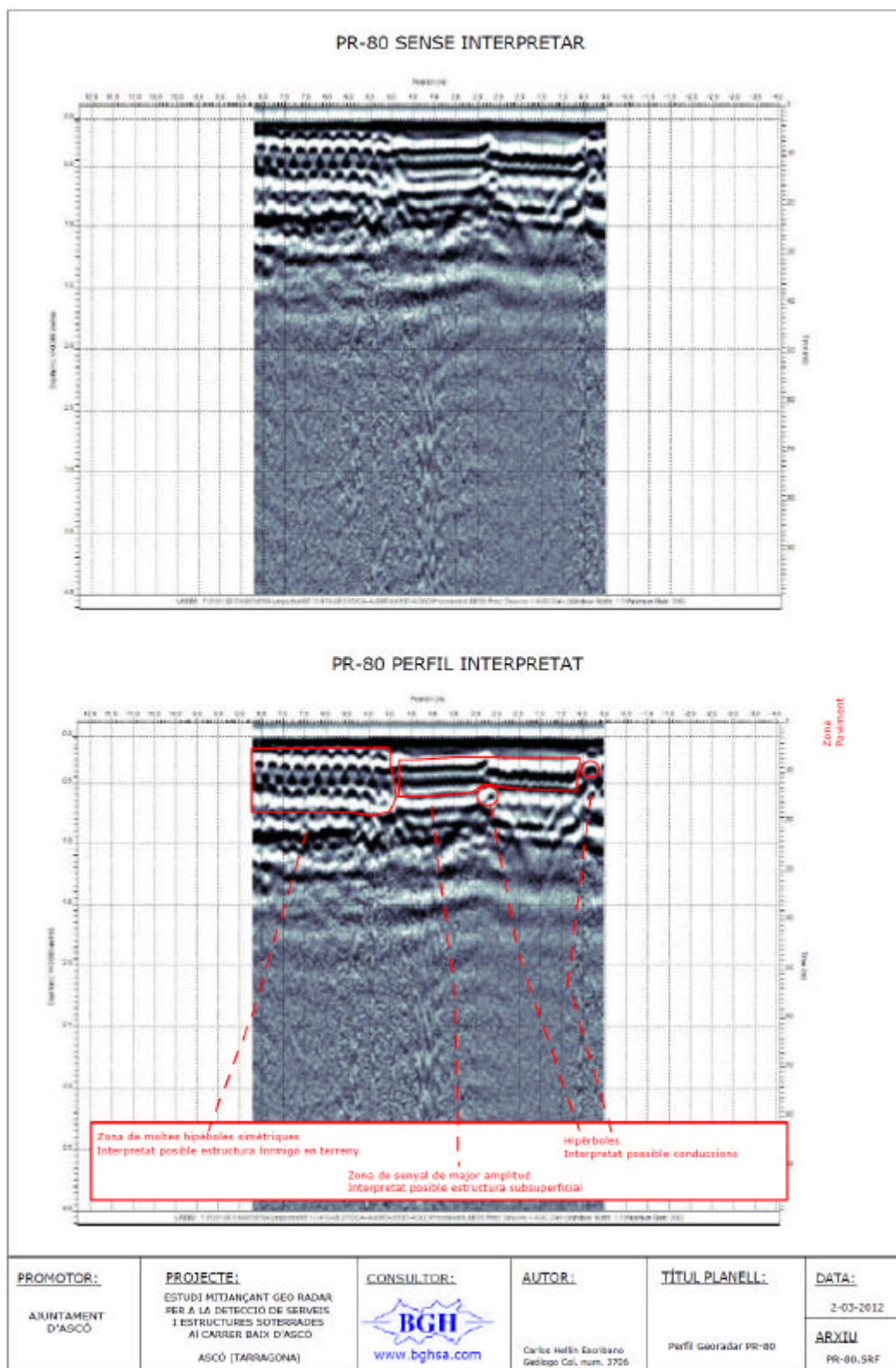
Figura 51. PR-80 PERFIL GEORADAR. Carrer de Baix, parteix sud. Costat est.
