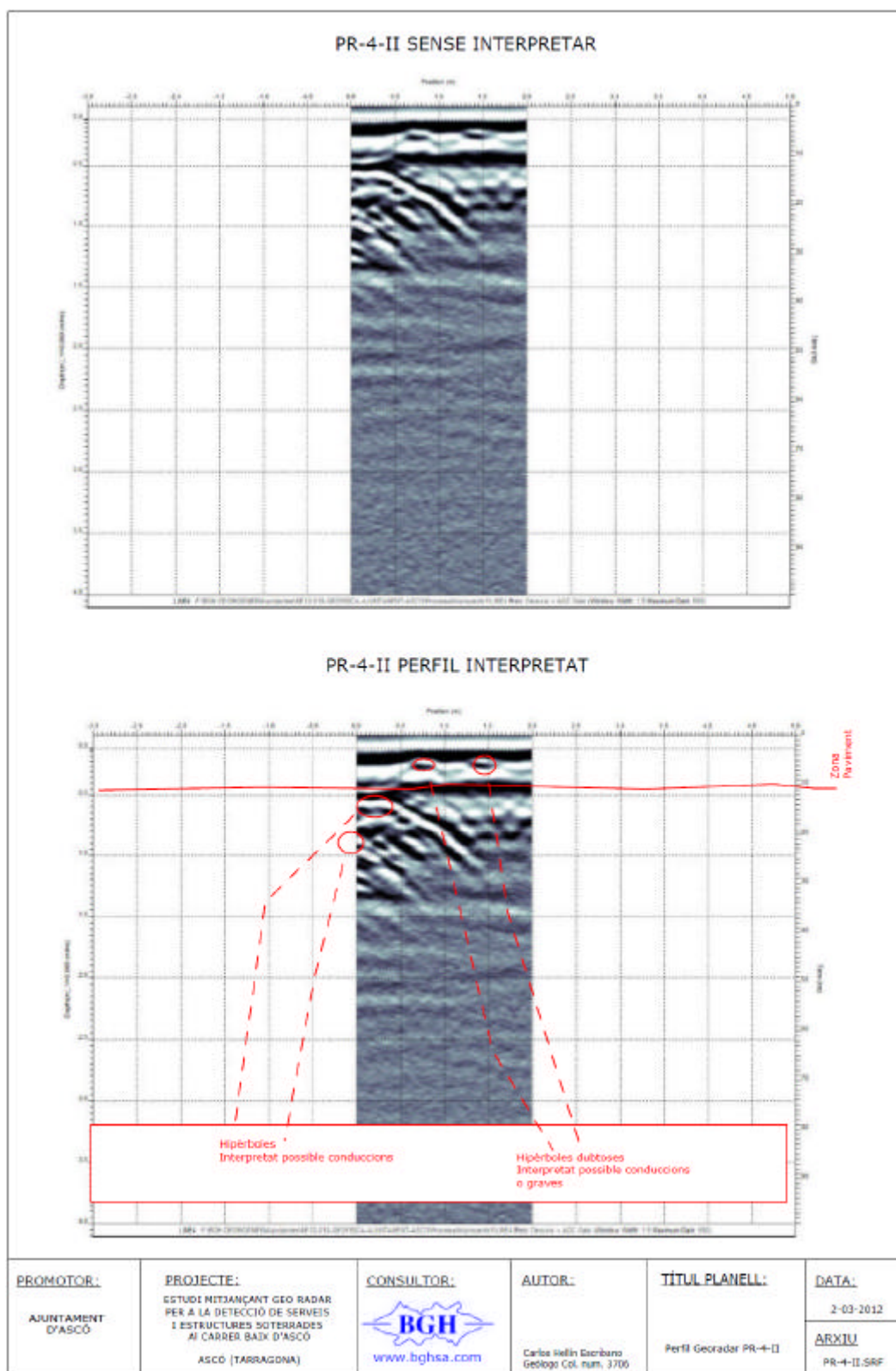
Figura 54. PR-4-II PERFIL GEORADAR. Transversal a Carrer de Baix.
