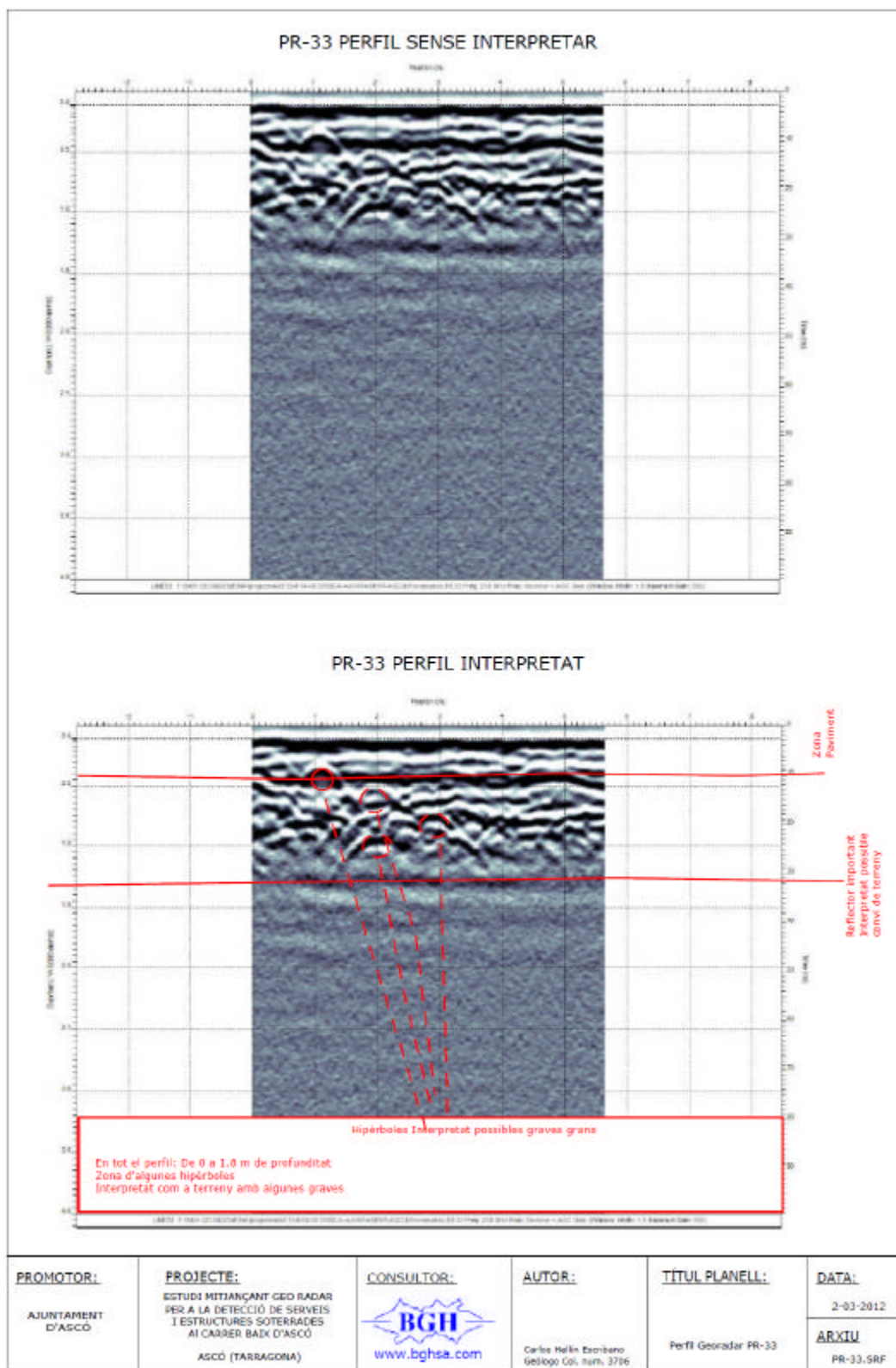
Figura 25. PR-33 PERFIL GEORADAR. Carrer al nord-centro de Carrer de Baix, costat nord.
