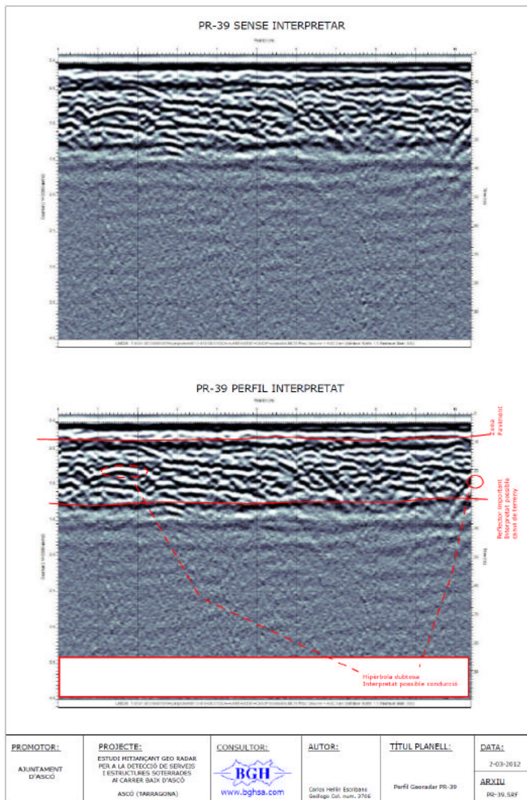
Figura 28. PR-39 PERFIL GEORADAR. Carrer situat al nord de la Plaça Major. Costat nord.
