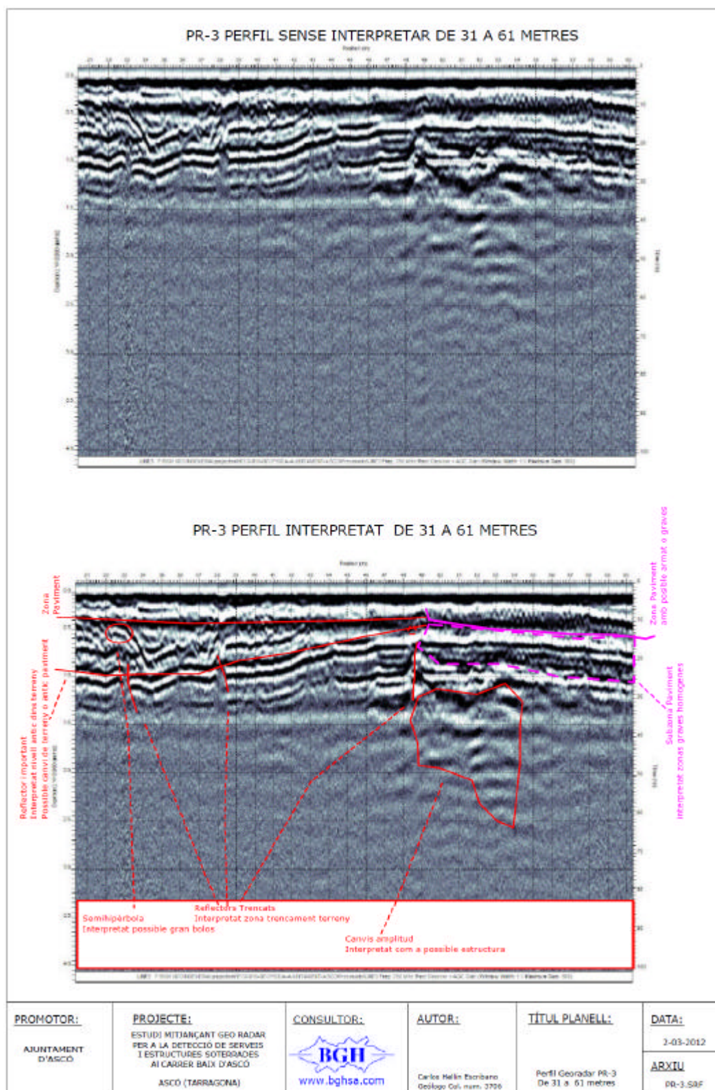
Figura 6. PR-3 PERFIL GEORADAR. Carrer de Baix. Costat oest. De 31 a 61 metres.
