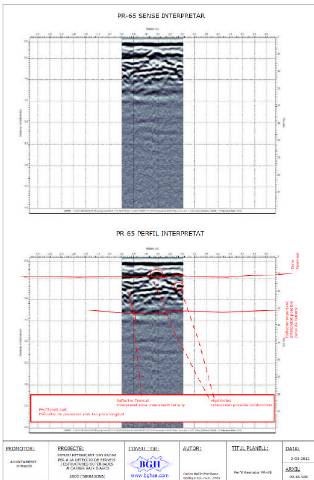
Figura 40. PR-65 PERFIL GEORADAR. Transversal en el Carrer al nord-centro de Carrer de Baix.
