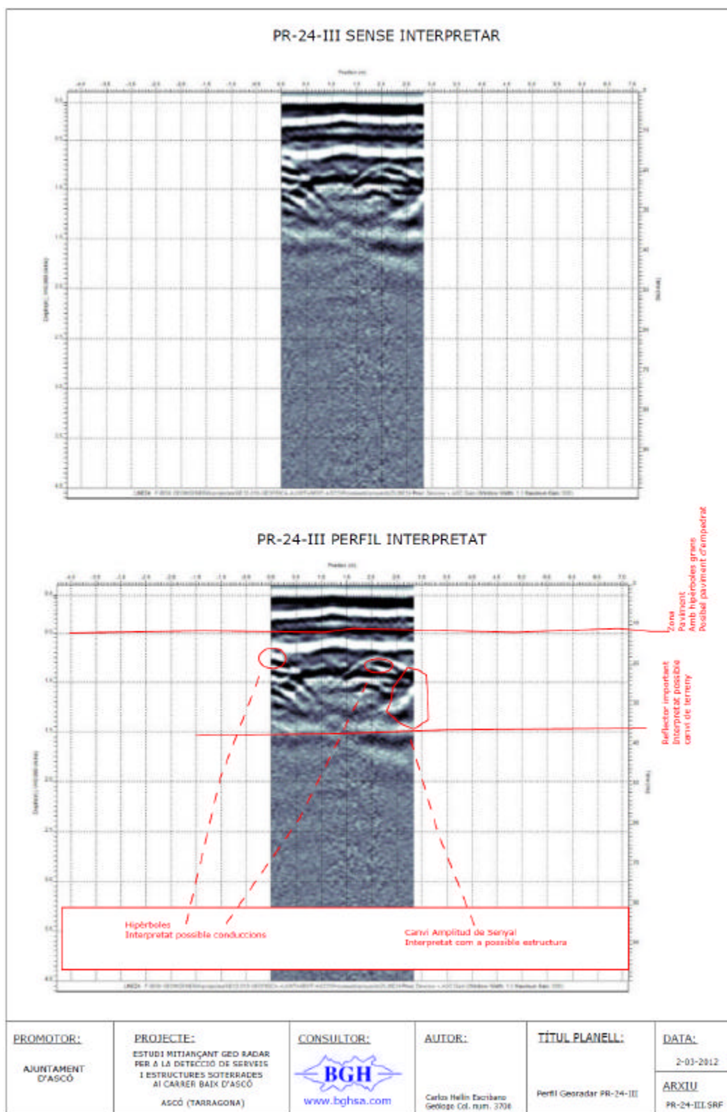
Figura 63. PR-24-III PERFIL GEORADAR. Transversal a Carrer de Baix.
