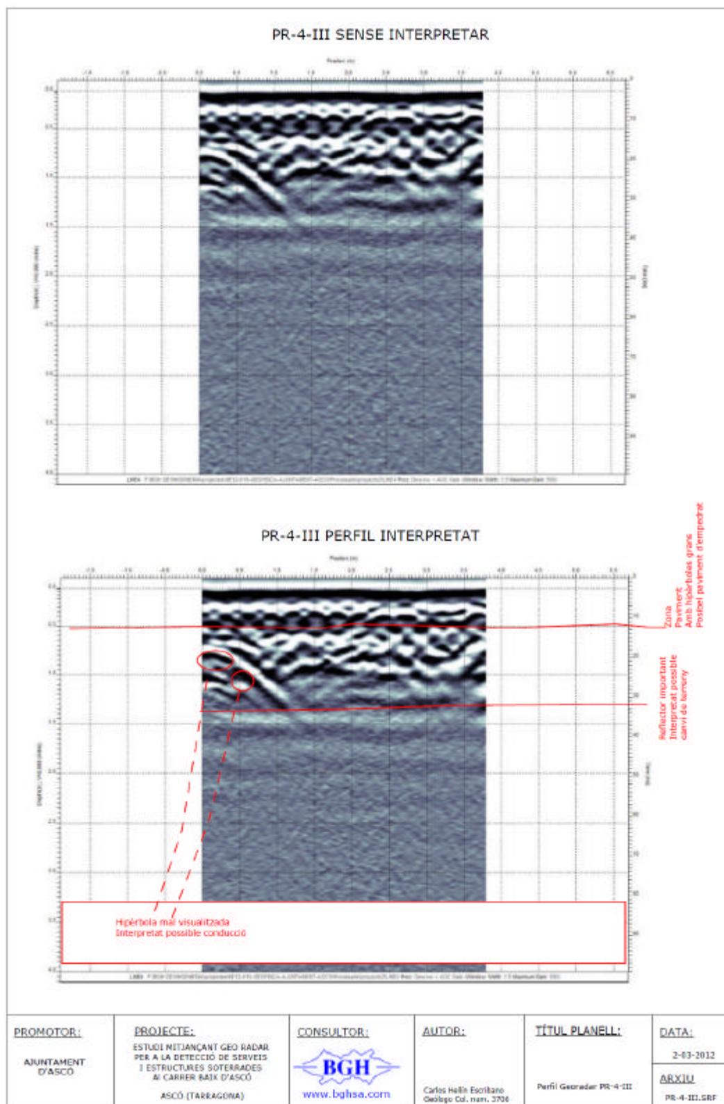
Figura 62. PR-4-III PERFIL GEORADAR. Transversal a Carrer de Baix.
