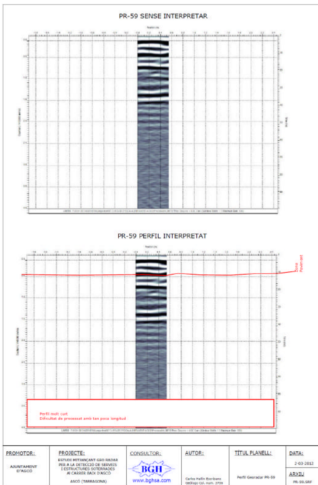
Figura 37. PR-59 PERFIL GEORADAR. Transversal en el Segon carrer perpendicular al Carrer de Baix al nord.
