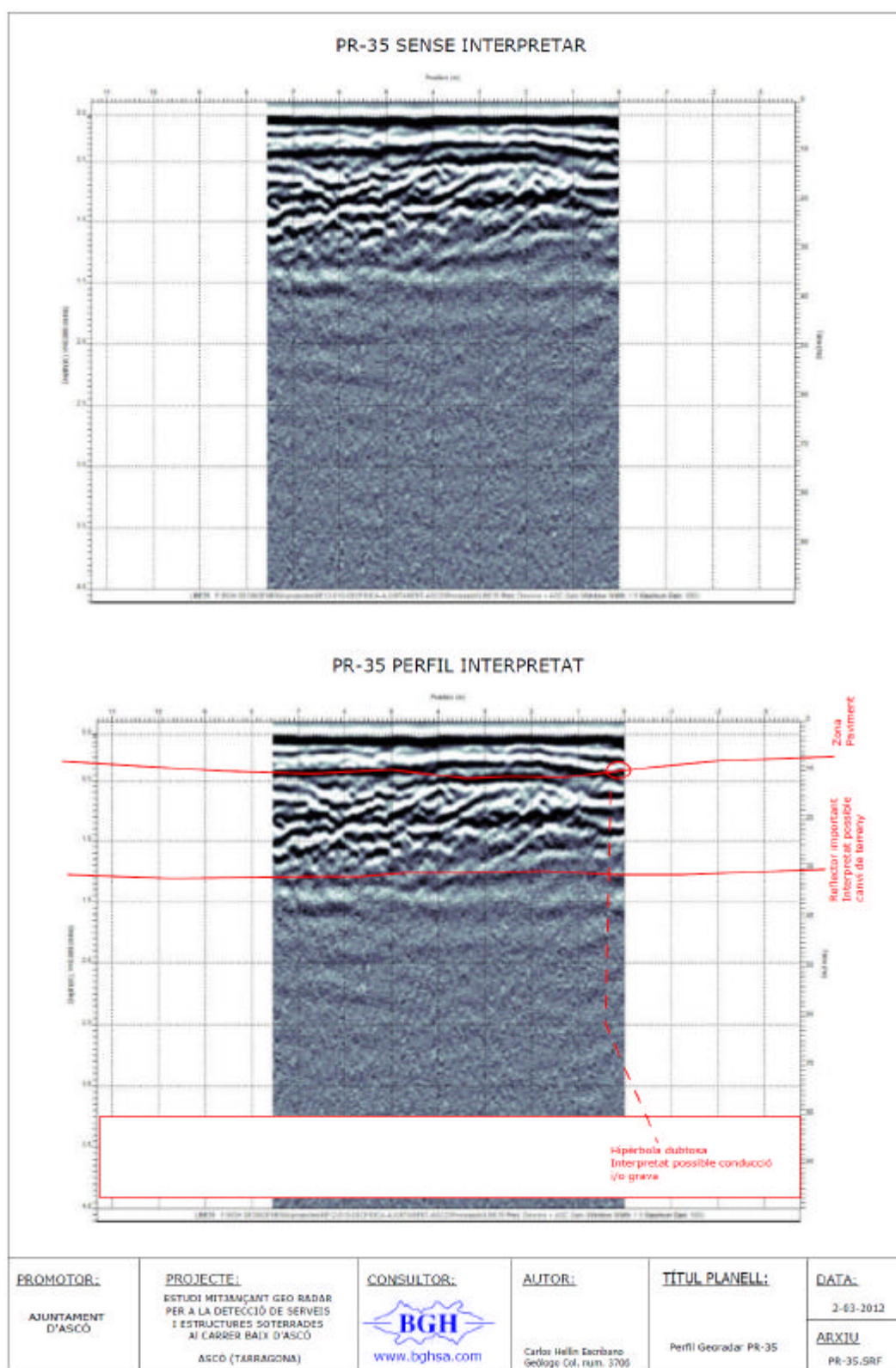
Figura 26. PR-35 PERFIL GEORADAR. Segon carrer perpendicular al Carrer de Baix al sud. Costat nord.
