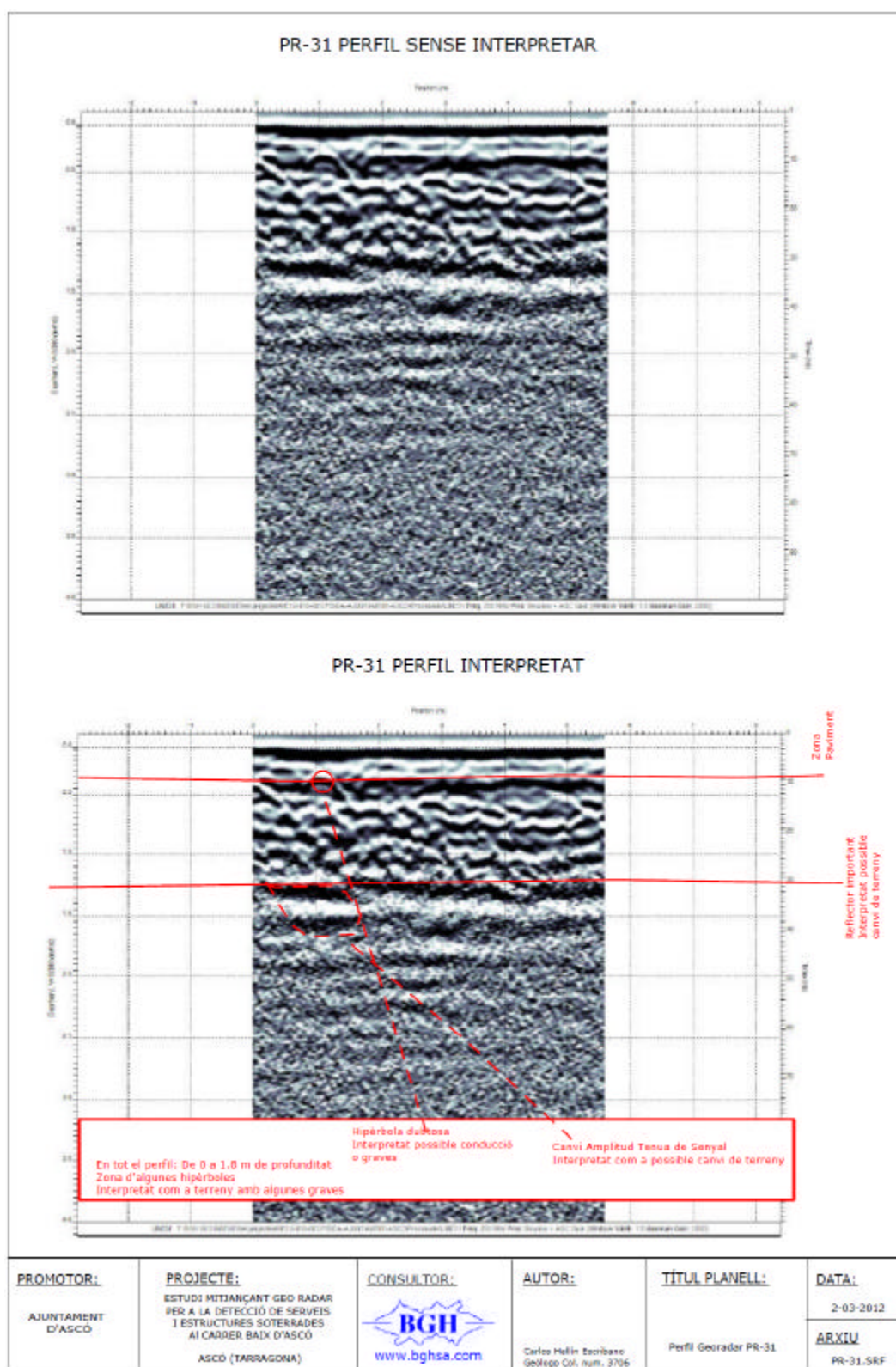
Figura 24. PR-31 PERFIL GEORADAR. Carrer al nord-centro de Carrer de Baix, zona centro.
