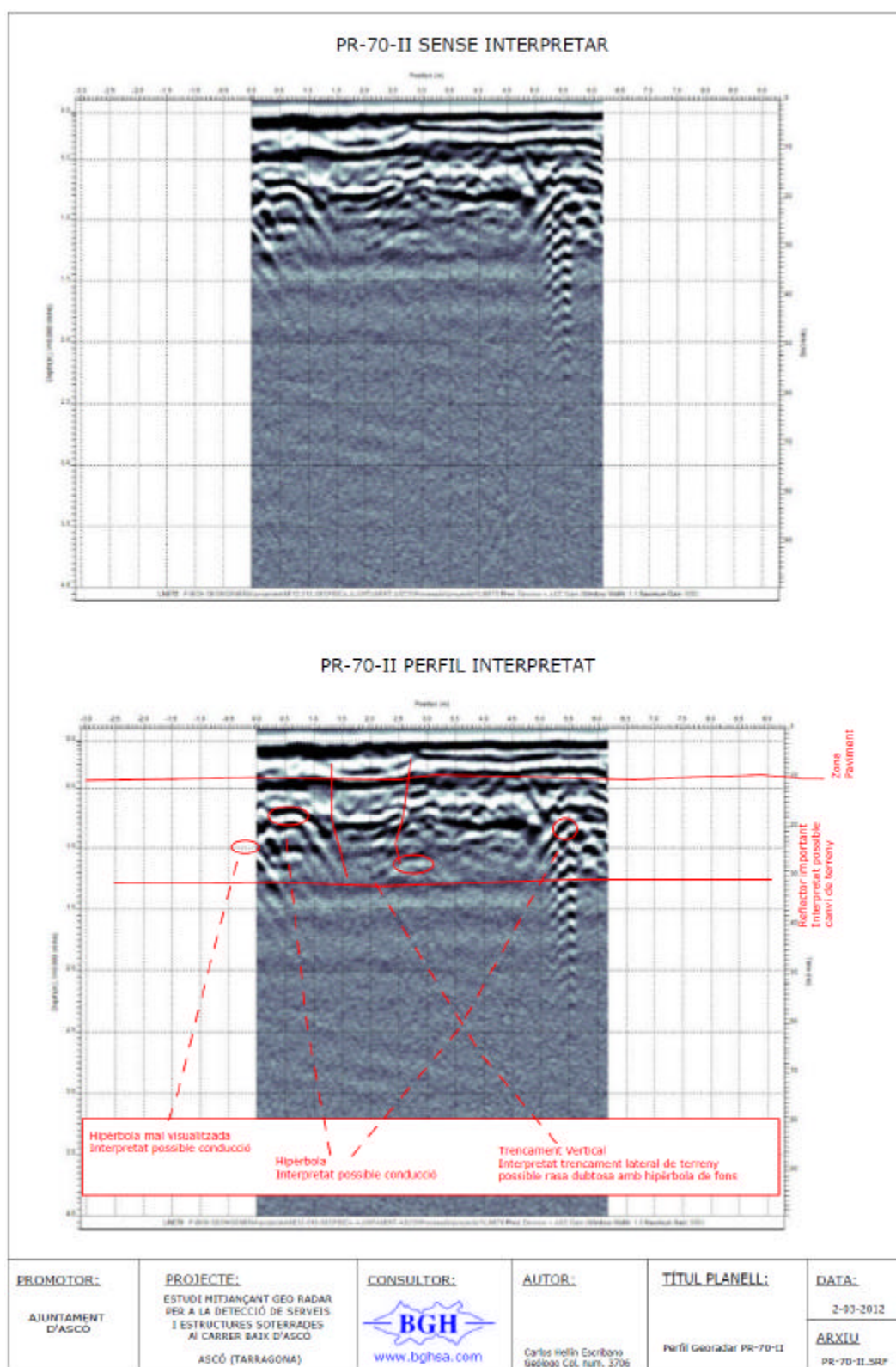
Figura 59. PR-70-II PERFIL GEORADAR. Transversal a Carrer de Baix.
