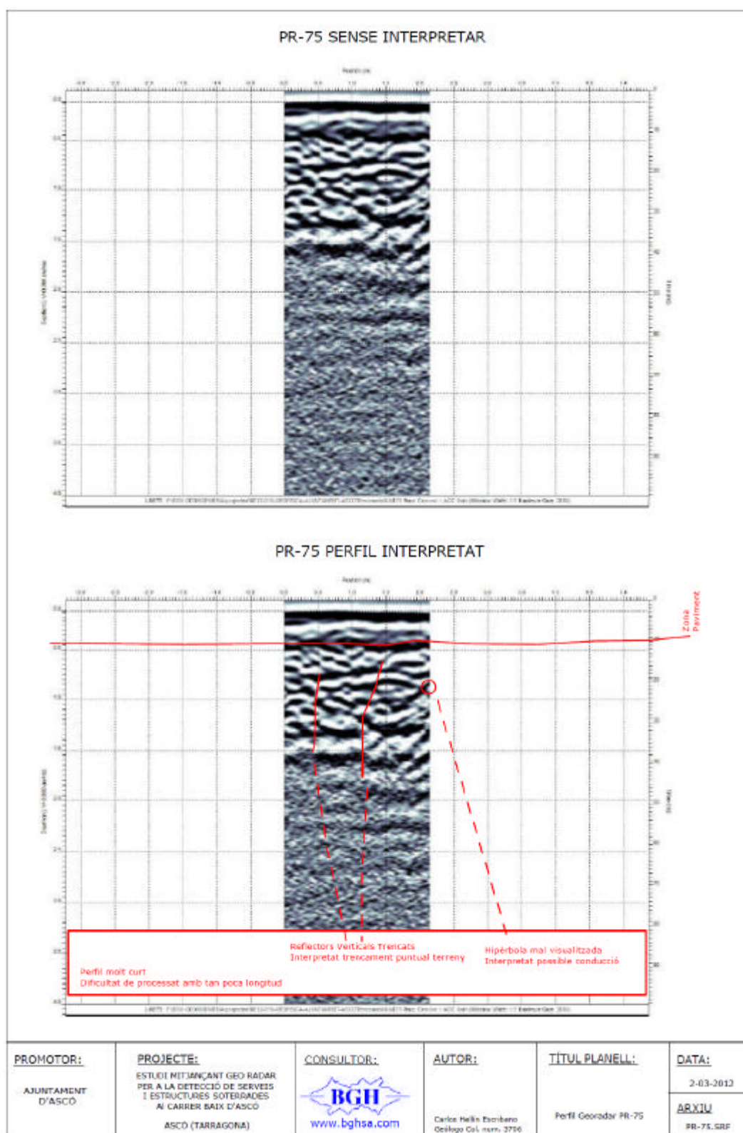
Figura 45. PR-75 PERFIL GEORADAR. Transversal en el carrer situat al nord de la Plaça Major.
