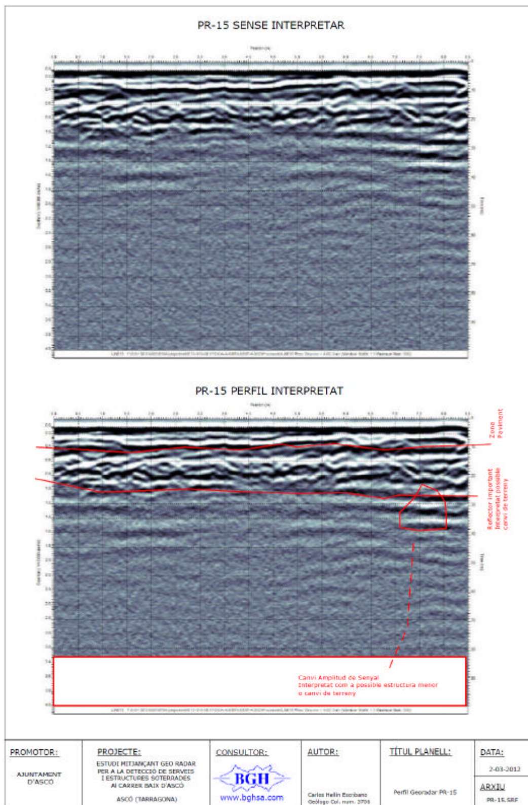
Figura 16. PR-15 PERFIL GEORADAR. Carrer Baixada Cavaller. Costat sud.
