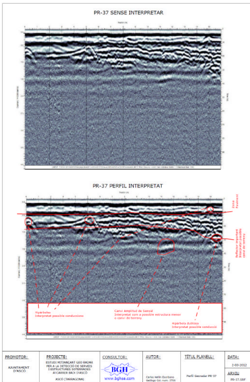
Figura 27. PR-37 PERFIL GEORADAR. Segon carrer perpendicular al Carrer de Baix al sud. Costat sud.
