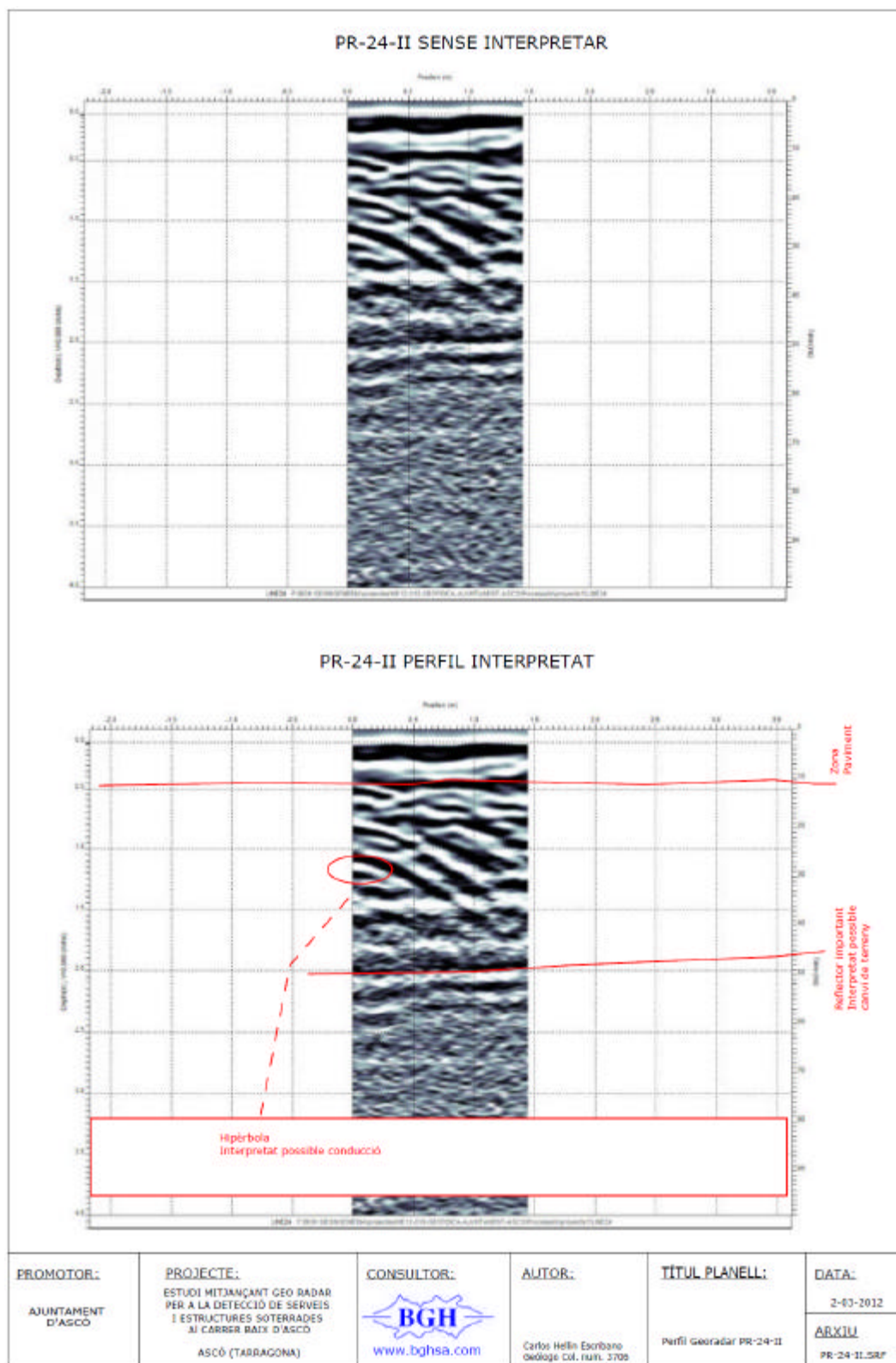
Figura 55. PR-24-II PERFIL GEORADAR. Transversal a Carrer de Baix.
