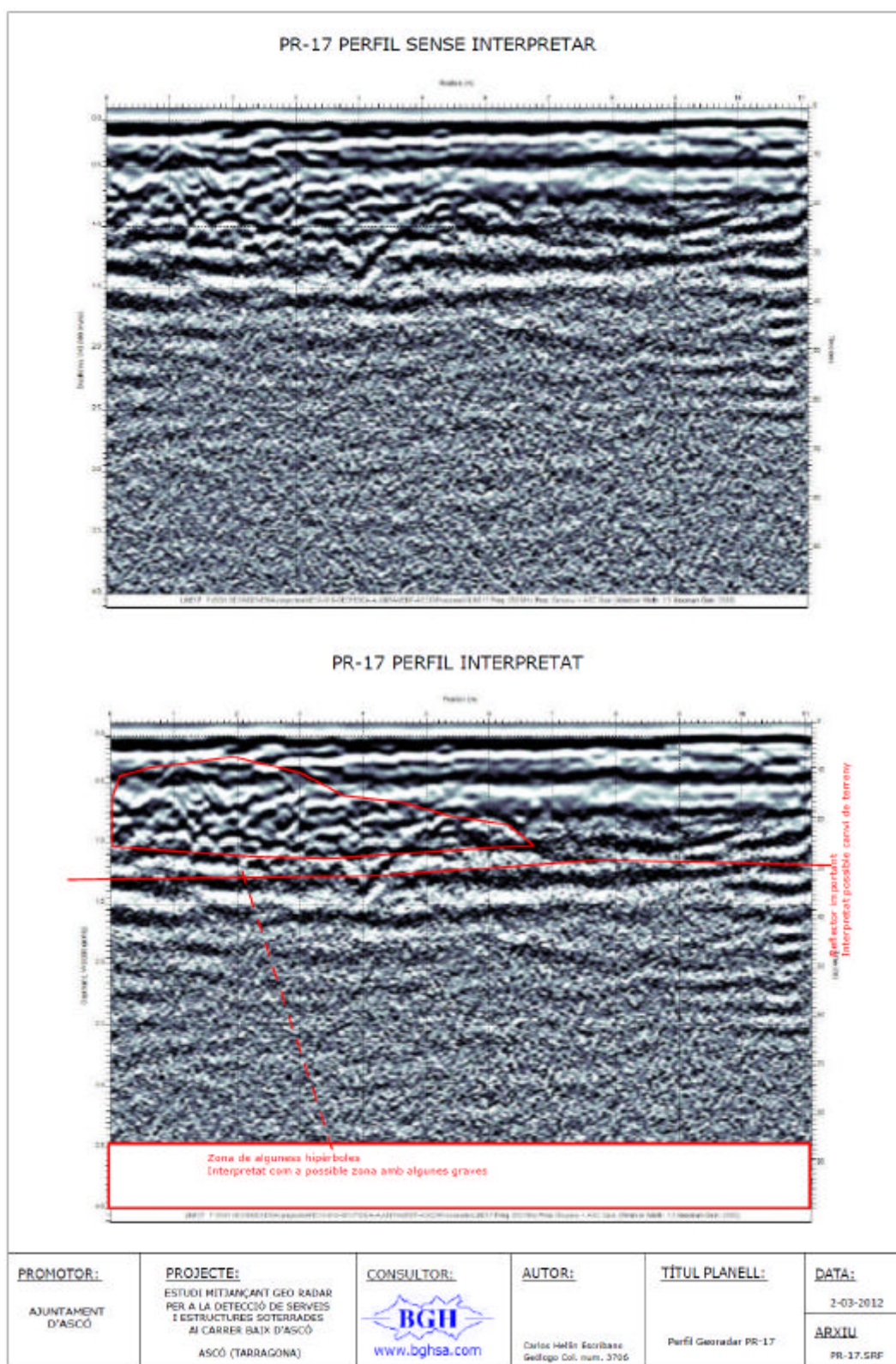
Figura 17. PR-17 PERFIL GEORADAR. Carrer Baixada Cavaller. Costat sud.
