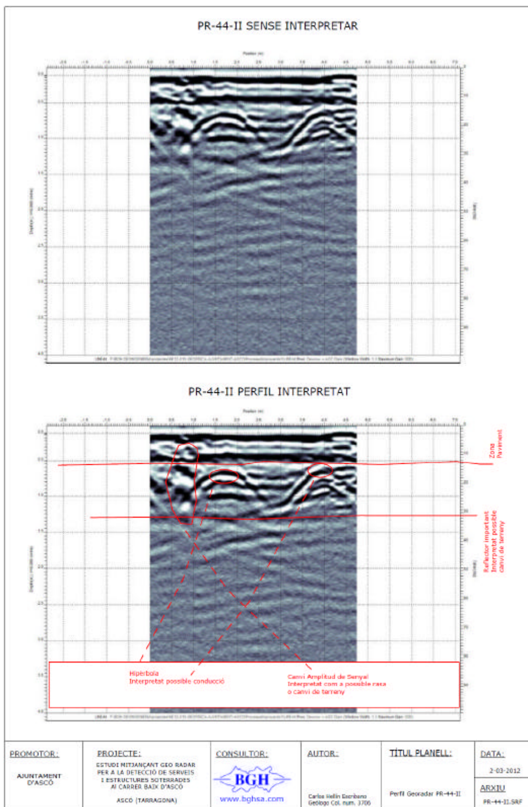
Figura 57. PR-44-II PERFIL GEORADAR. Transversal a Carrer de Baix.
