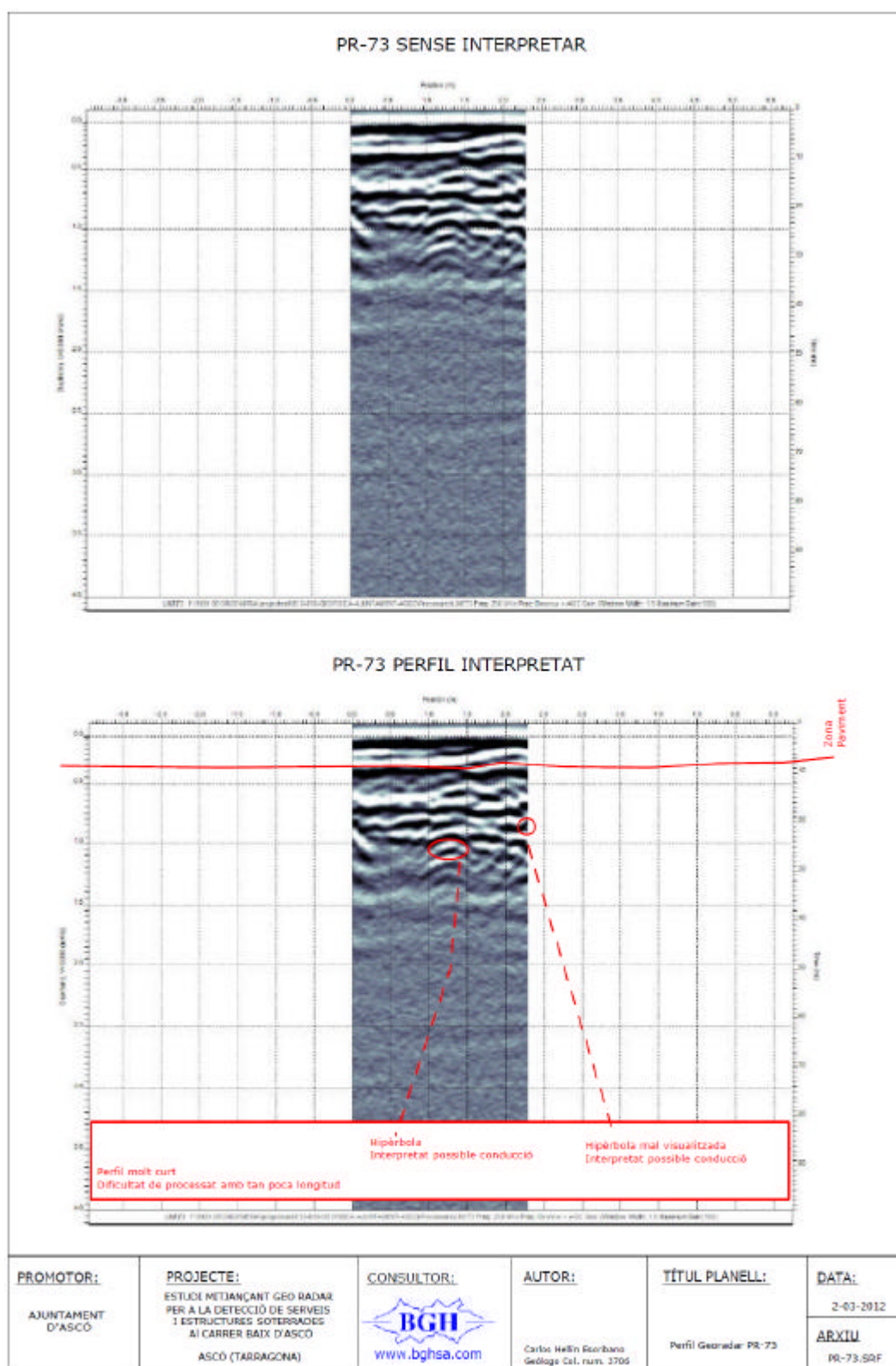
Figura 44. PR-73 PERFIL GEORADAR. Transversal en el carrer situat al nord de la Plaça Major.
