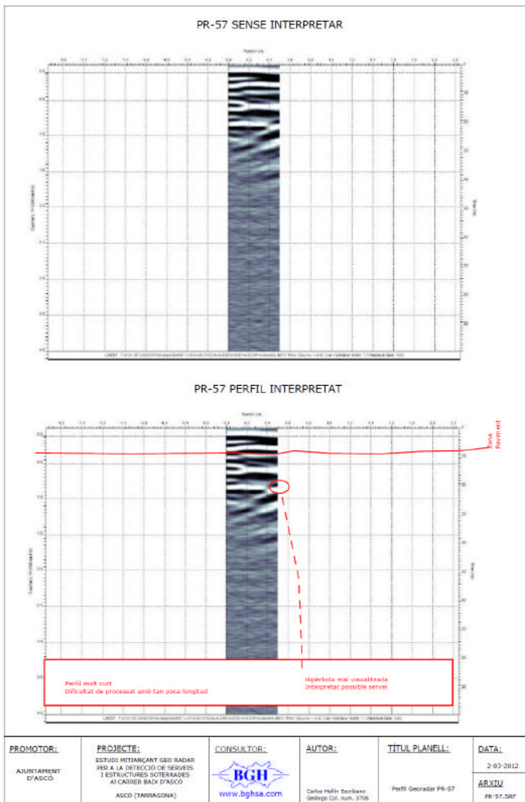
Figura 36. PR-57 PERFIL GEORADAR. Transversal a la baixada del Carrer de Baix.
