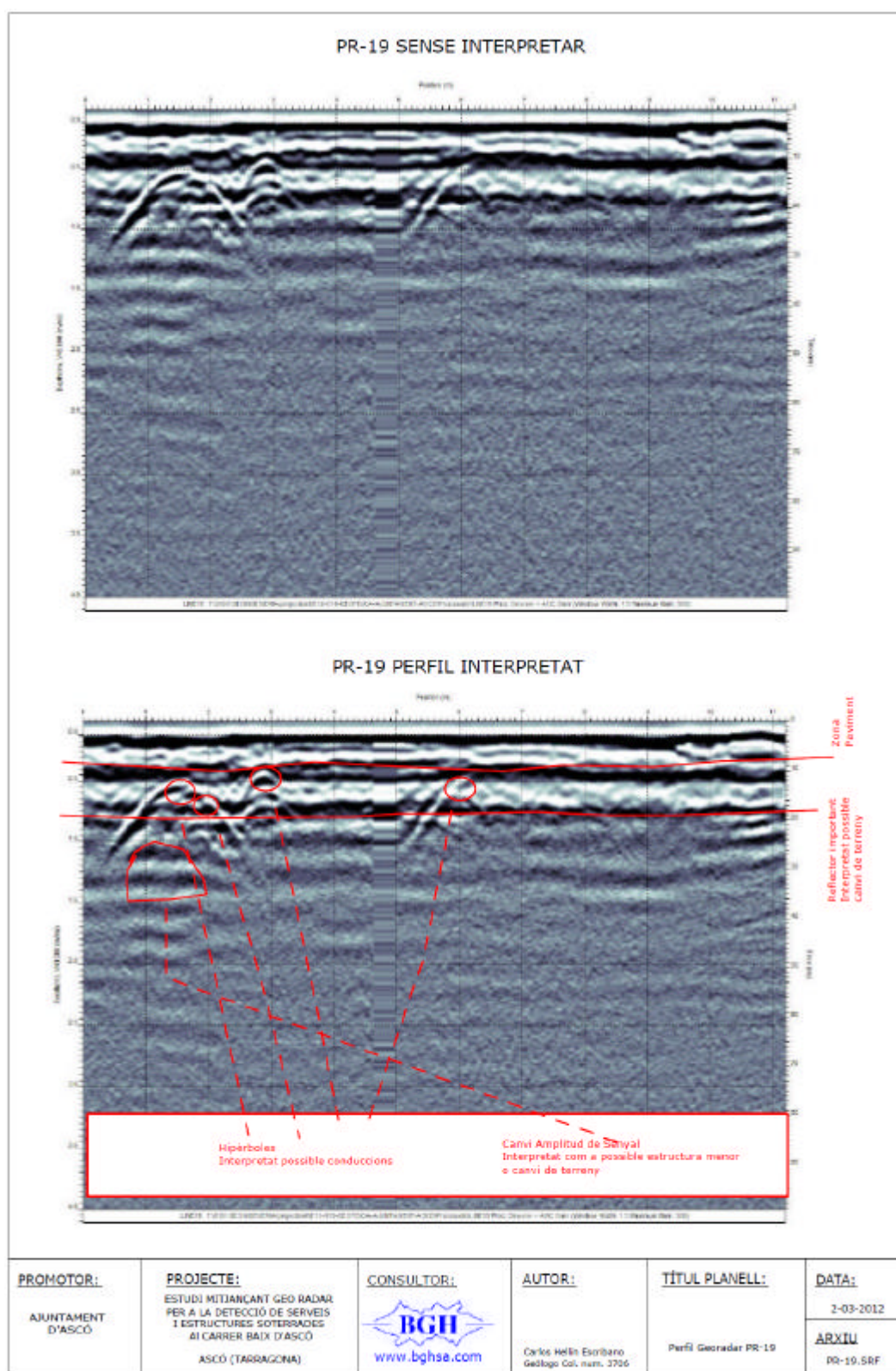
Figura 18. PR-19 PERFIL GEORADAR. Baixada des de Carrer de Baix, sud.
