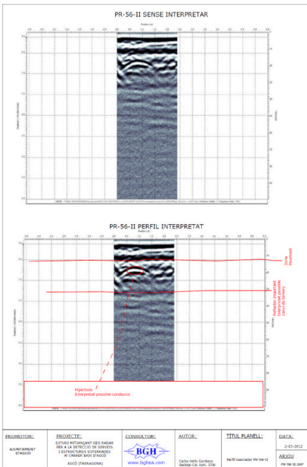
Figura 58. PR-56-II PERFIL GEORADAR. Transversal a Carrer de Baix.
