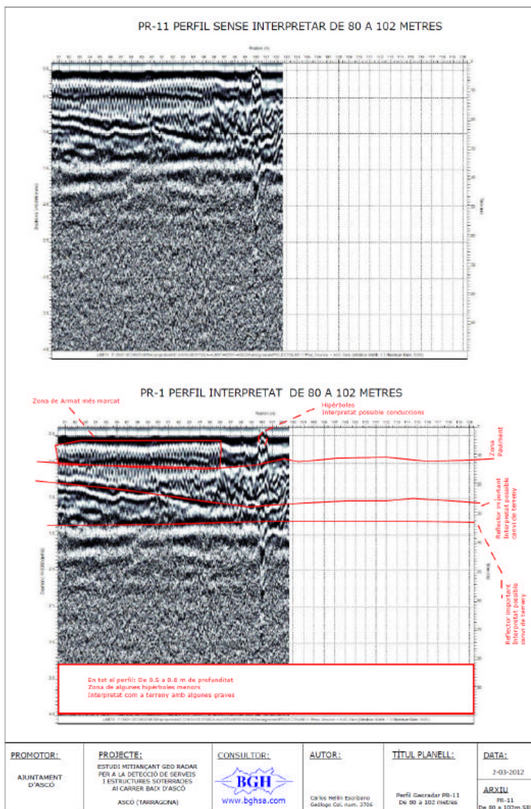
Figura 14. PR-11 PERFIL GEORADAR. Carrer de Baix. Costat est. De 80 a 102 metres.
