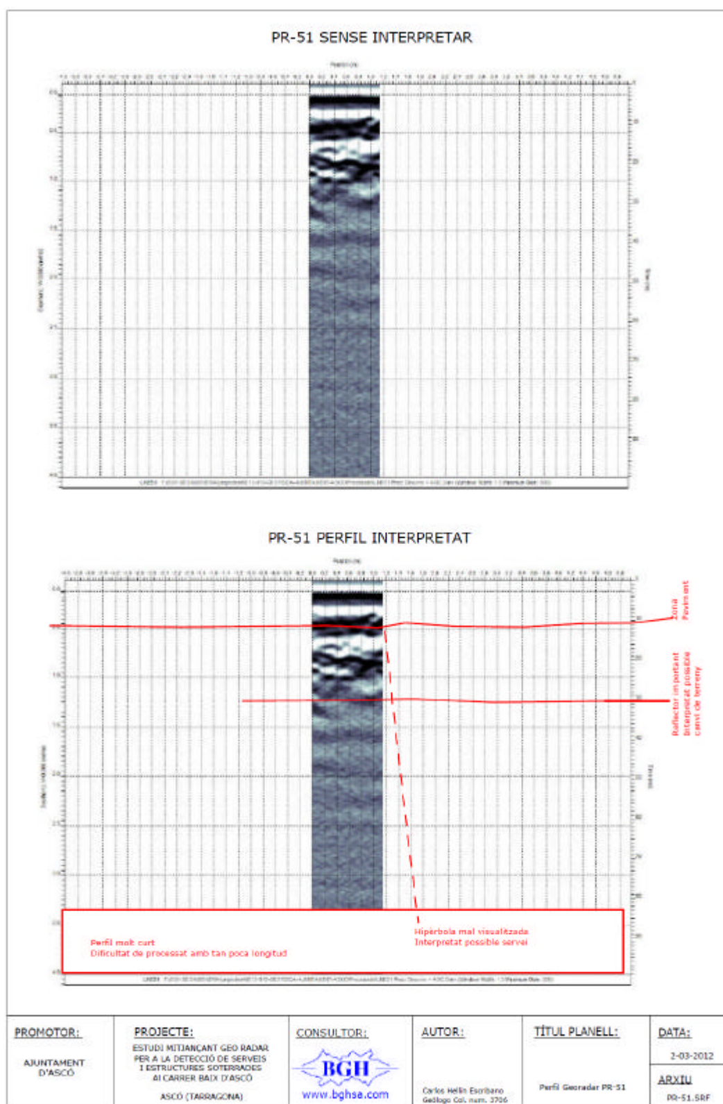
Figura 33. PR-51 PERFIL GEORADAR. Transversal, en el quart replà de les escales que van al Carrer Bajunja.
