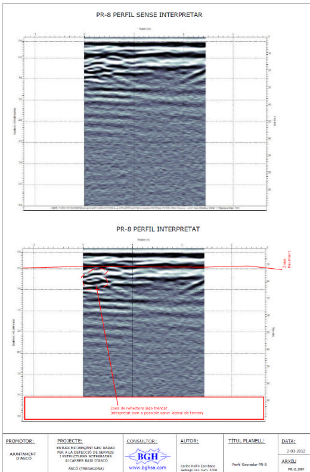
Figura 11. PR-8 PERFIL GEORADAR. Carrer de Baix. Costat est.
