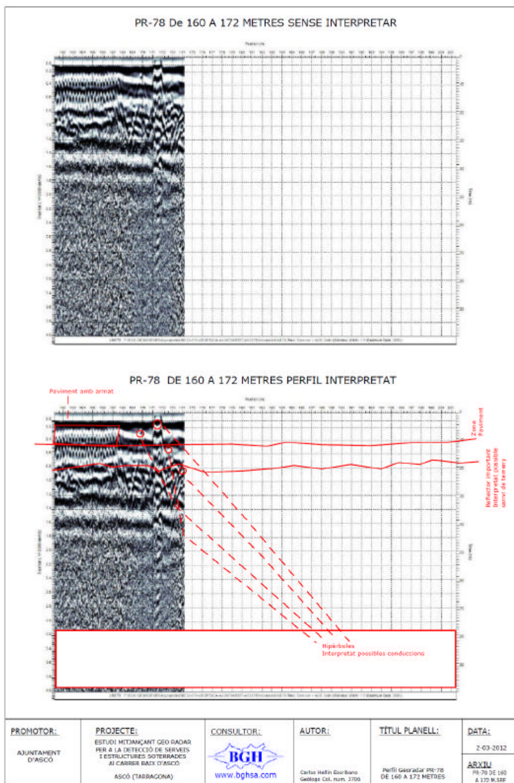
Figura 50. PR-78 PERFIL GEORADAR. Carrer de Baix. Centre. De 0 a 40 metres
