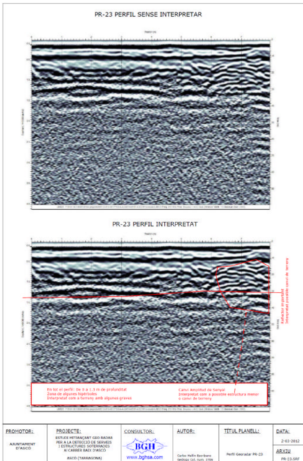
Figura 20. PR-23 PERFIL GEORADAR. Segon carrer perpendicular al Carrer de Baix al nord. Costat sud.
