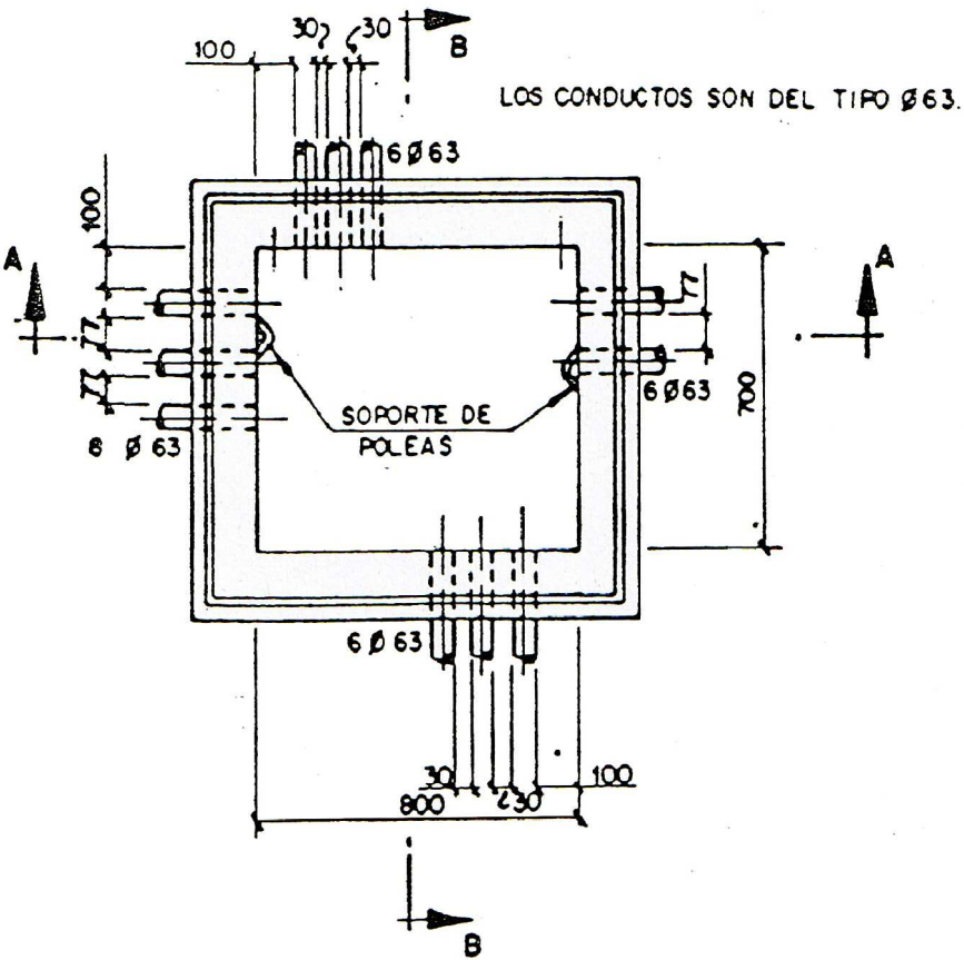
COTAS EN mm DIMENSIONAT I ENTRADES D' ARQUETA TIPUS H
