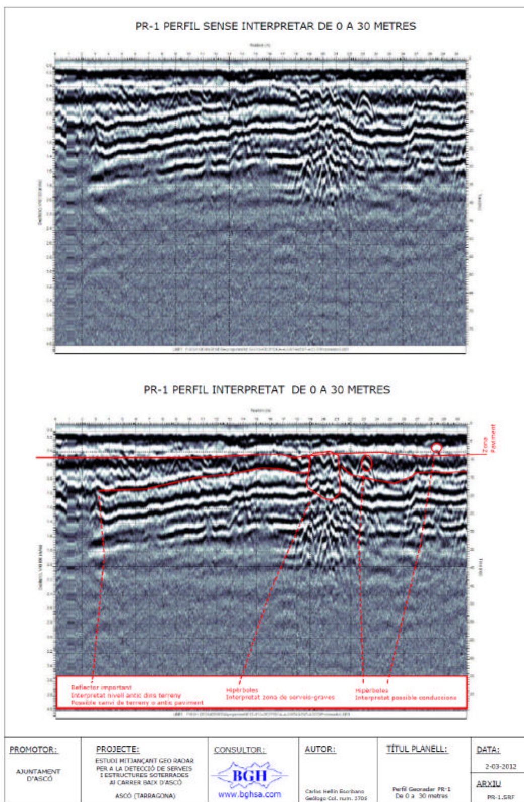
Figura 3. PR-1 PERFIL GEORADAR. Carrer de Baix. Costat oest. De 0 a 30 metres.
