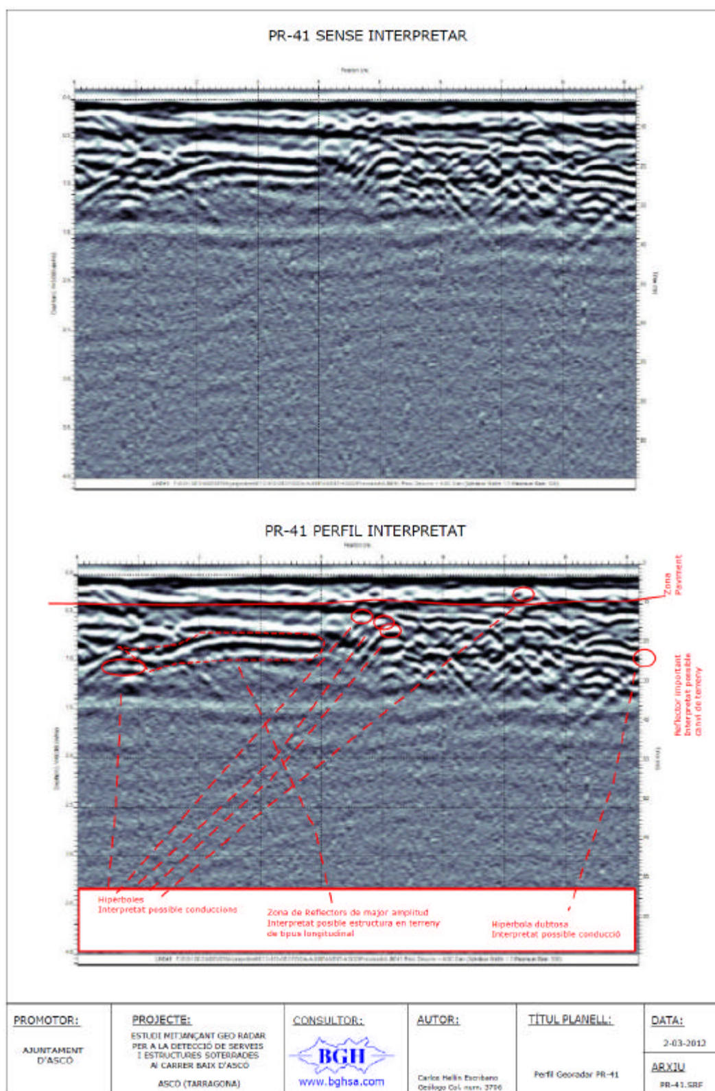
Figura 29. PR-41 PERFIL GEORADAR. Carrer situat al nord de la Plaça Major. Costat sud.
