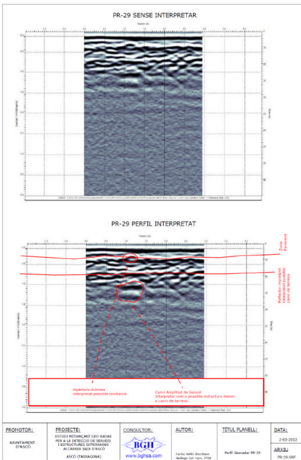
Figura 23. PR-29 PERFIL GEORADAR. Carrer al nord-centro de Carrer de Baix, costat sud.
