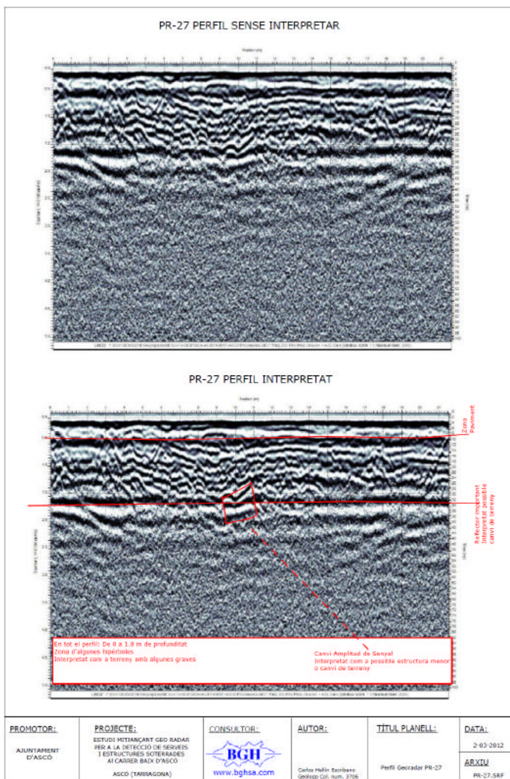
Figura 22. PR-27 PERFIL GEORADAR. Carrer paral·lel al Carrer de Baix, al nord. Costat sud.
