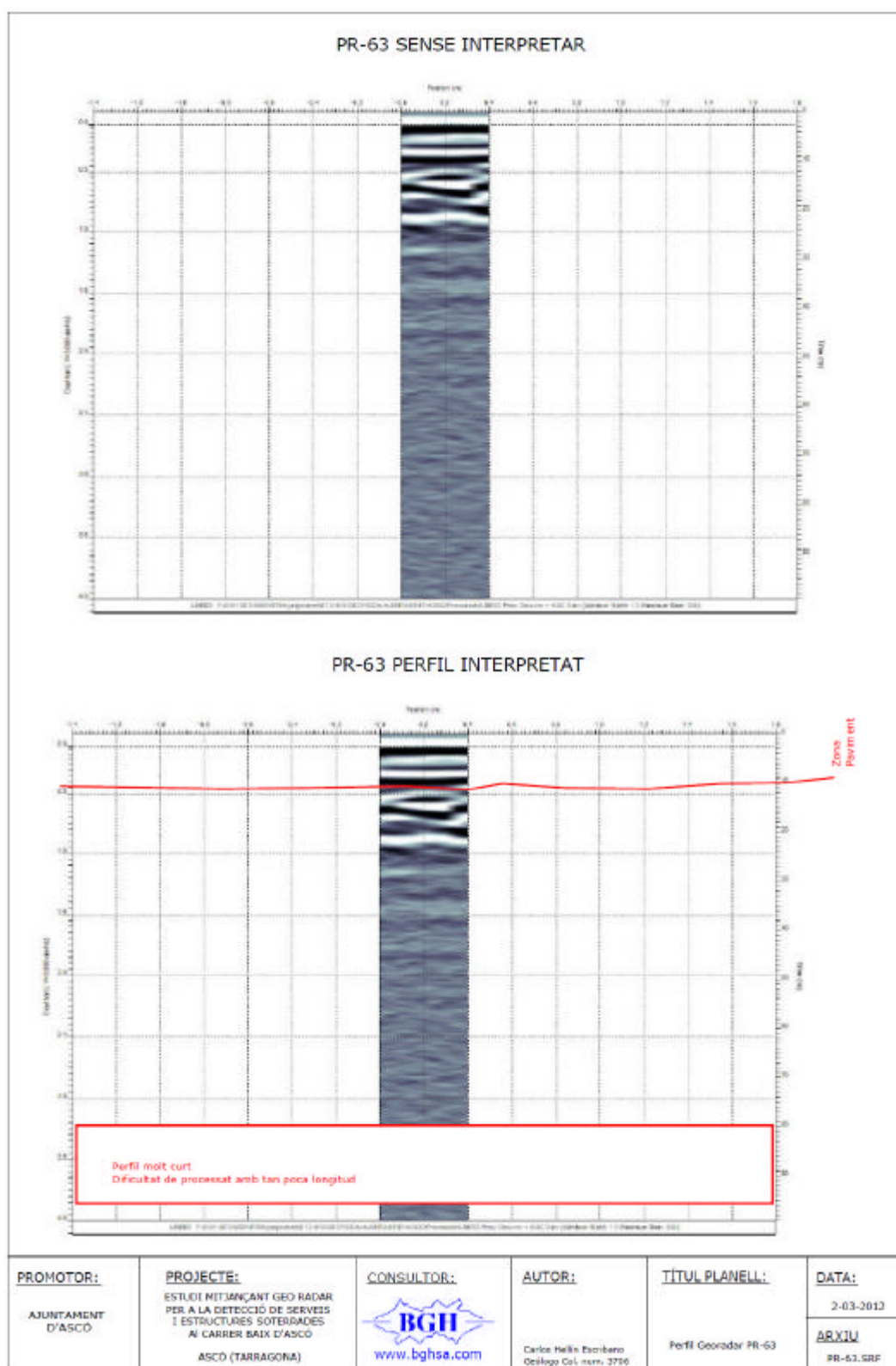
Figura 39. PR-63 PERFIL GEORADAR. Transversal en el Carrer paral·lel al Carrer de Baix, al nord.
