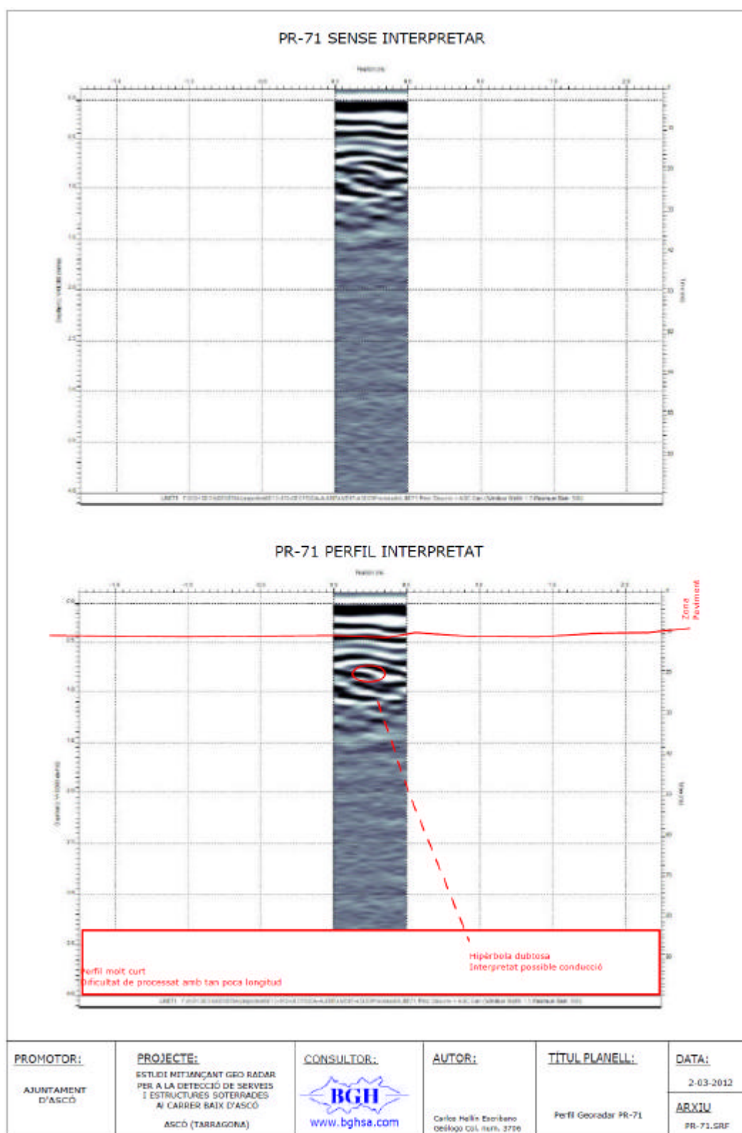
Figura 43. PR-71 PERFIL GEORADAR. Transversal en el segon carrer perpendicular al Carrer de Baix al sud.
