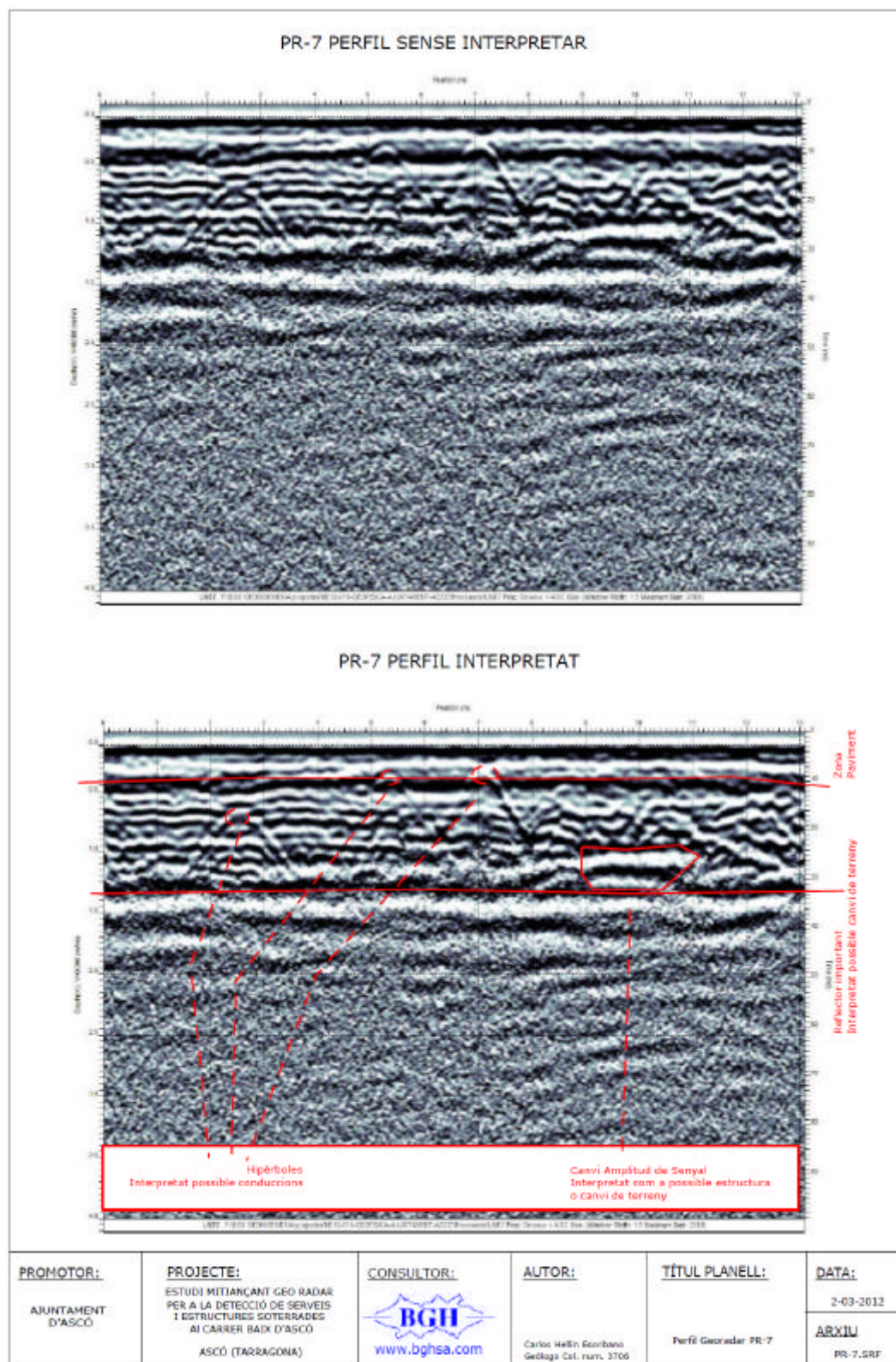
Figura 10. PR-7 PERFIL GEORADAR. Carrer de Baix. Costat est.
