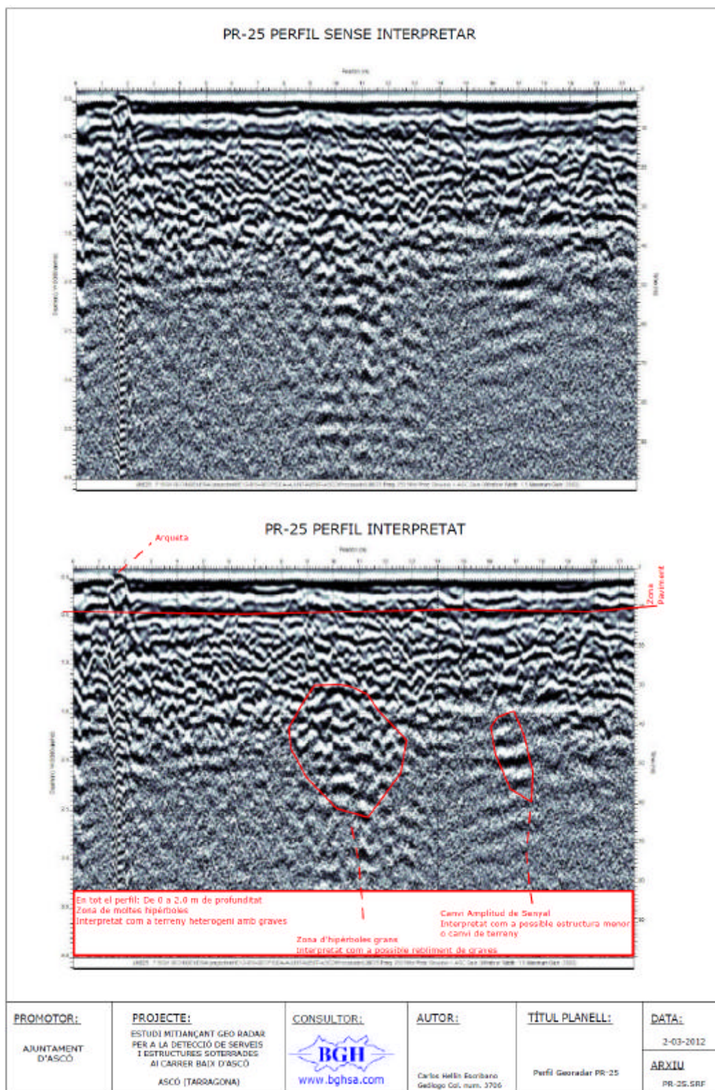
Figura 21. PR-25 PERFIL GEORADAR. Carrer paral·lel al Carrer de Baix, al nord. Costat nord.
