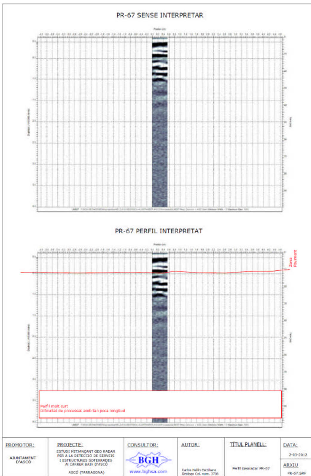
Figura 41. PR-67 PERFIL GEORADAR. Transversal en el segon carrer perpendicular al Carrer de Baix al sud.
