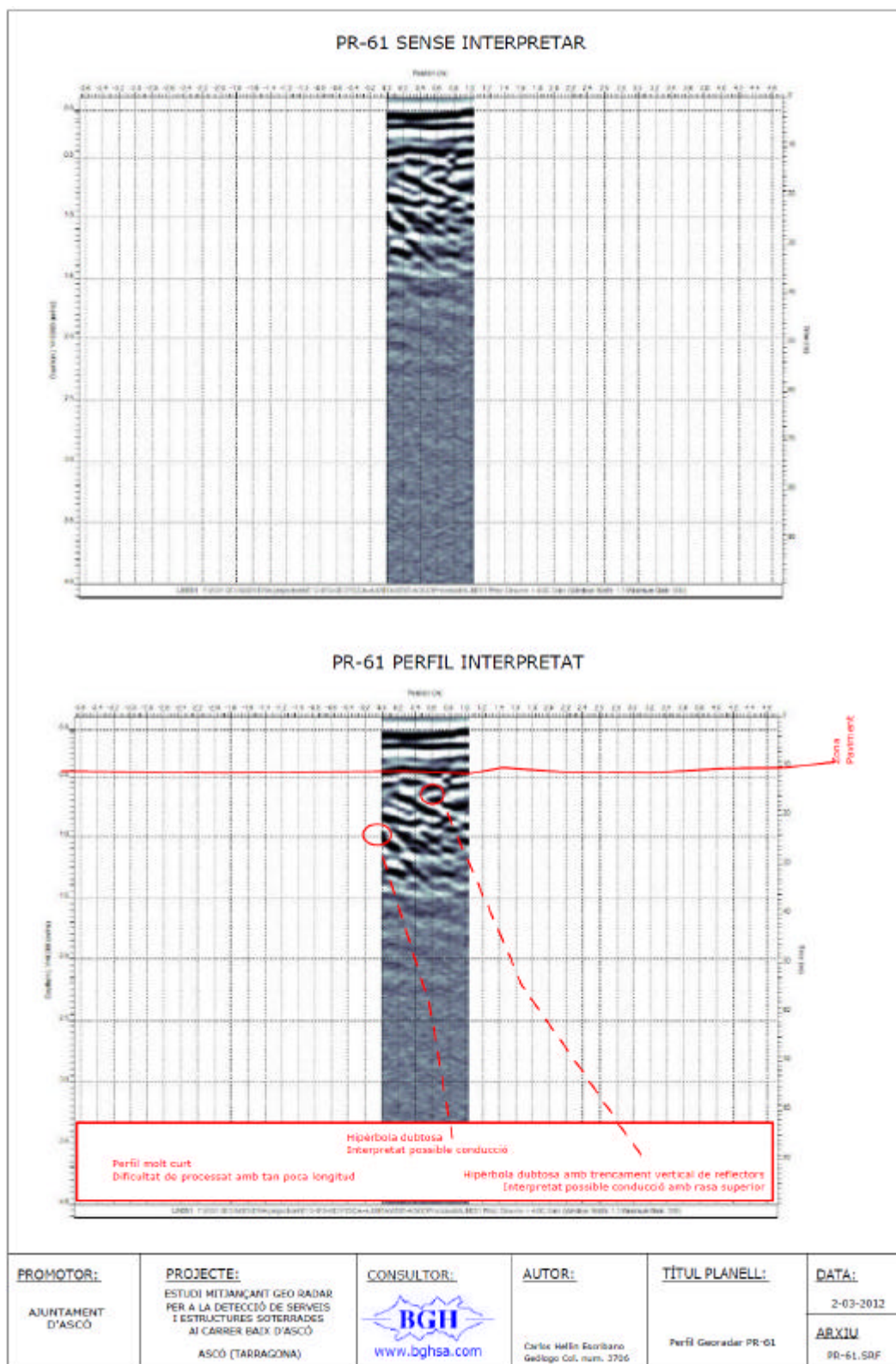
Figura 38. PR-61 PERFIL GEORADAR. Transversal en el Carrer paral·lel al Carrer de Baix, al nord.
