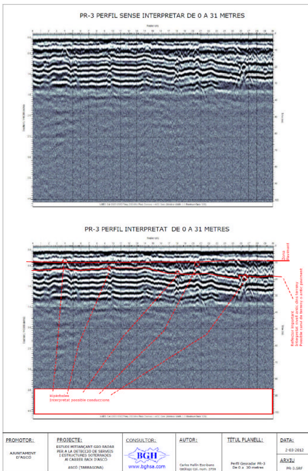
Figura 5. PR-3 PERFIL GEORADAR. Carrer de Baix. Costat oest. De 0 a 31 metres.
