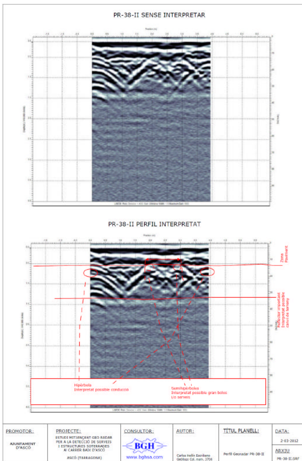
Figura 56. PR-38-II PERFIL GEORADAR. Transversal a Carrer de Baix.
