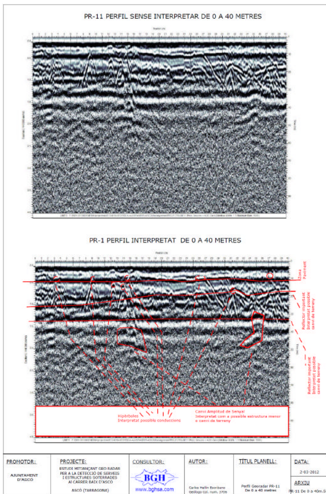
Figura 12. PR-11 PERFIL GEORADAR. Carrer de Baix. Costat est. De 0 a 40 metres.
