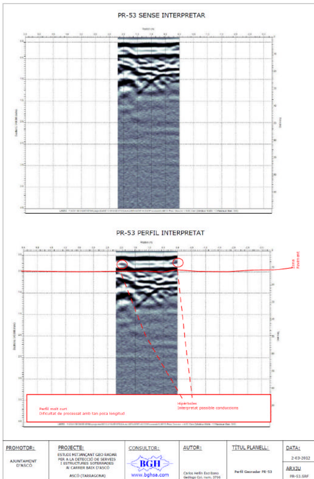
Figura 34. PR-53 PERFIL GEORADAR. Longitudinal, en el cinquè replà de les escales que van al Carrer Baijunca.
