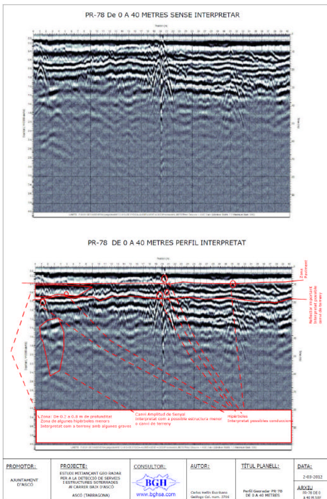
Figura 46. PR-78 PERFIL GEORADAR. Carrer de Baix. Centre. De 0 a 40 metres
