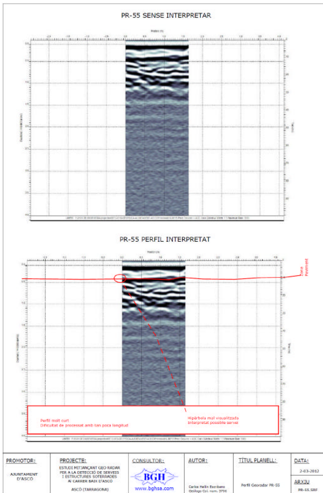
Figura 35. PR-55 PERFIL GEORADAR. Transversal, en el cinquè replà de les escales que van al Carrer Baijunca.
