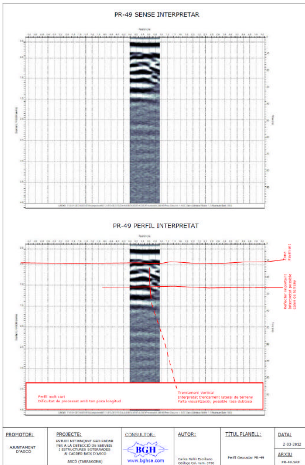
Figura 32. PR-49 PERFIL GEORADAR. Transversal, en el tercer replà de les escales que van al Carrer Baijunca.
