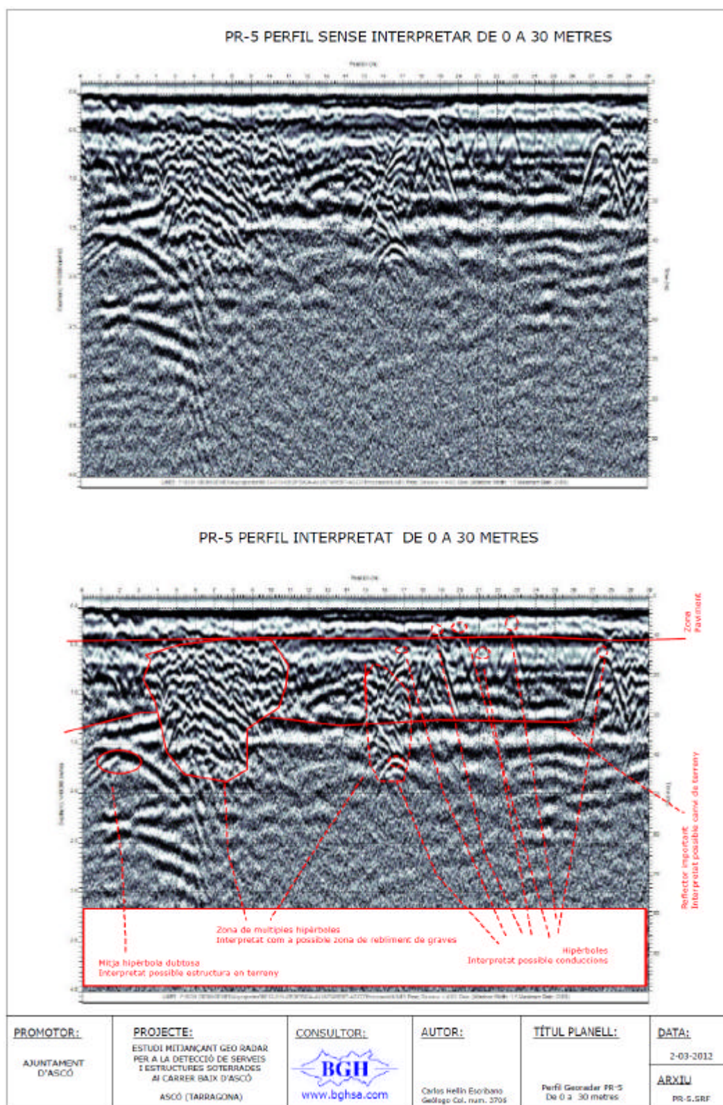
Figura 8. PR-5 PERFIL GEORADAR. Carrer de Baix. Costat est. De 0 a 30 metres.
