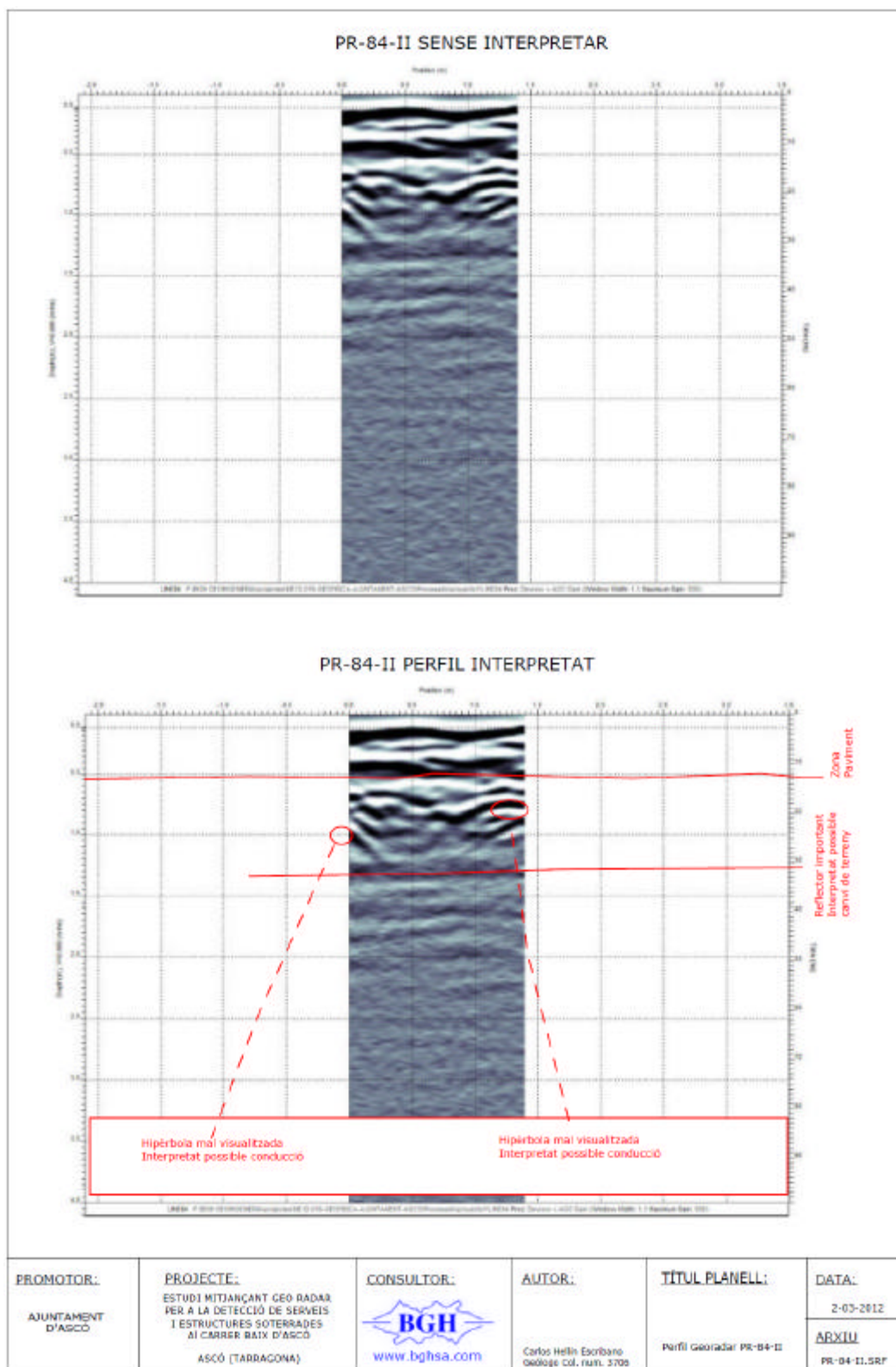
Figura 61. PR-84-II PERFIL GEORADAR. Transversal a Carrer de Baix.
