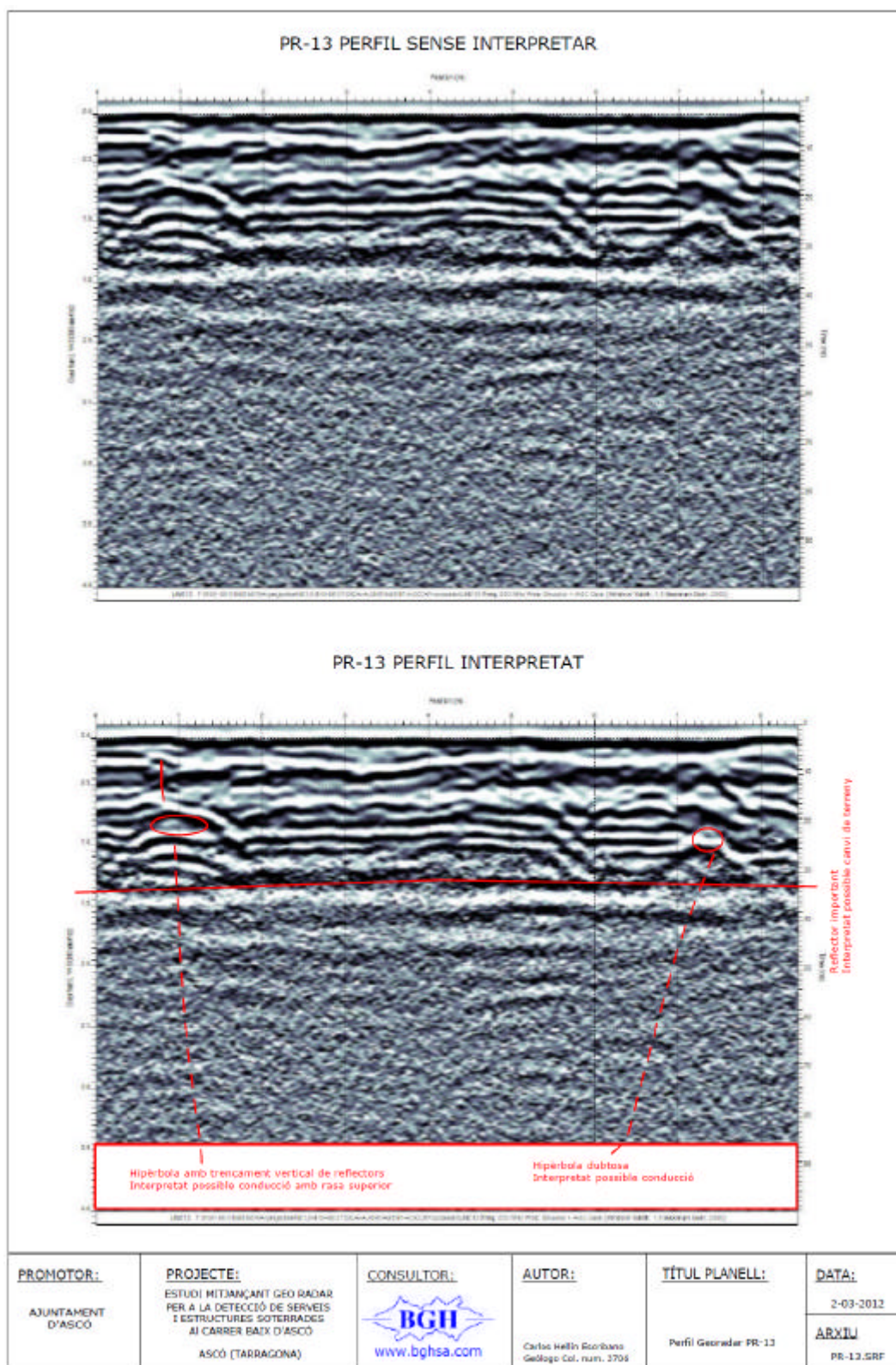
Figura 15. PR-13 PERFIL GEORADAR. Carrer Baixada Cavaller. Costat nord.
