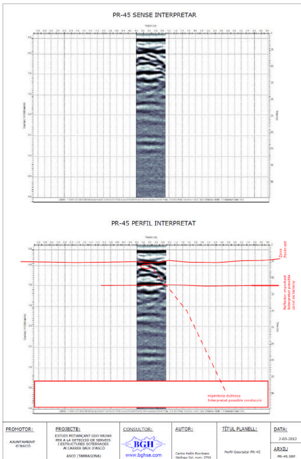
Figura 30. PR-45 PERFIL GEORADAR. Transversal, en el primer replà de les escales que van al Carrer Baijuna.
