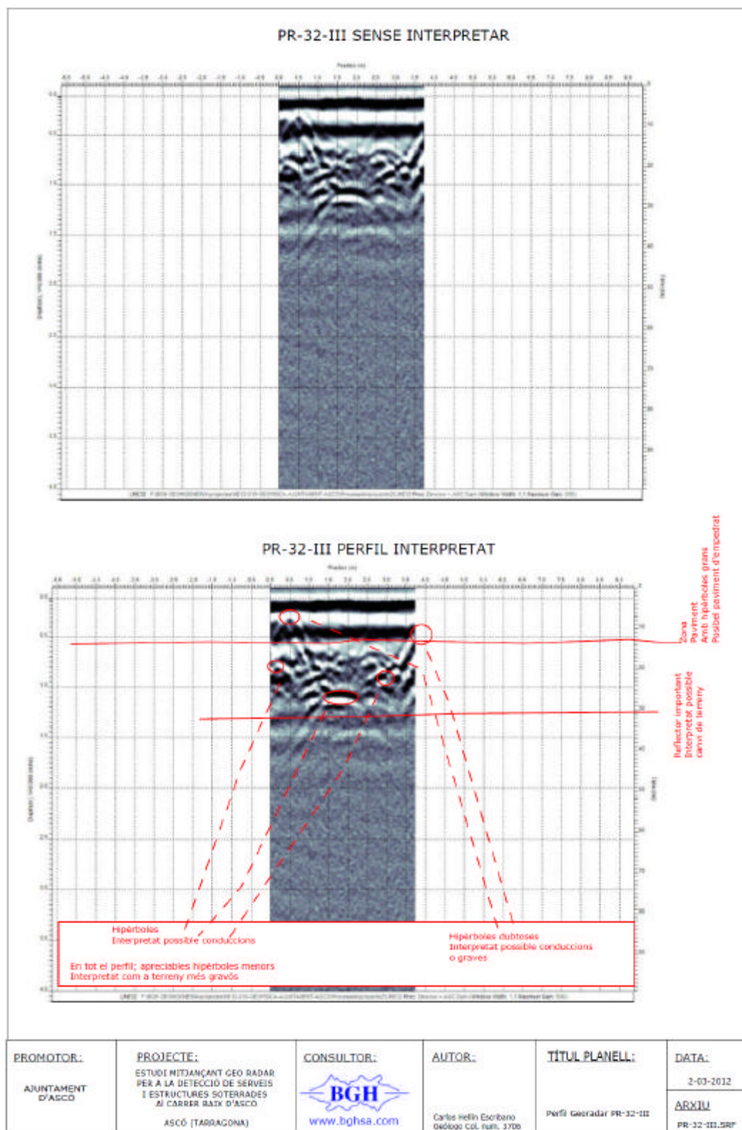
Figura 64. PR-32-III PERFIL GEORADAR. Transversal a Carrer de Baix.
