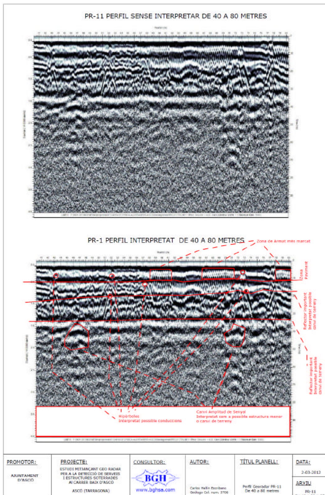
Figura 13. PR-11 PERFIL GEORADAR. Carrer de Baix. Costat est. De 40 a 80 metres.
