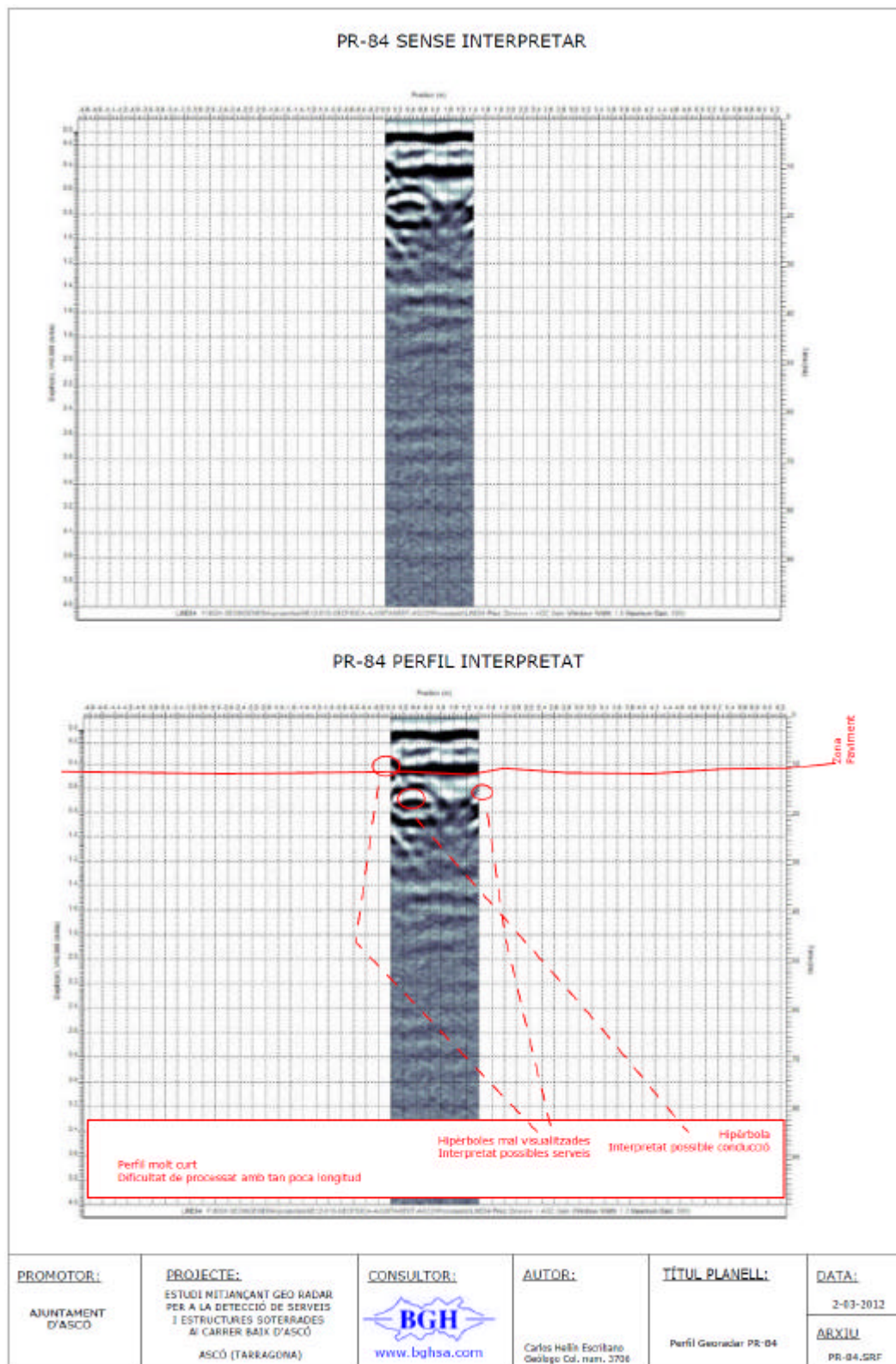
Figura 53. PR-84 PERFIL GEORADAR. Transversal a Carrer de Baix. Inici Carrer
