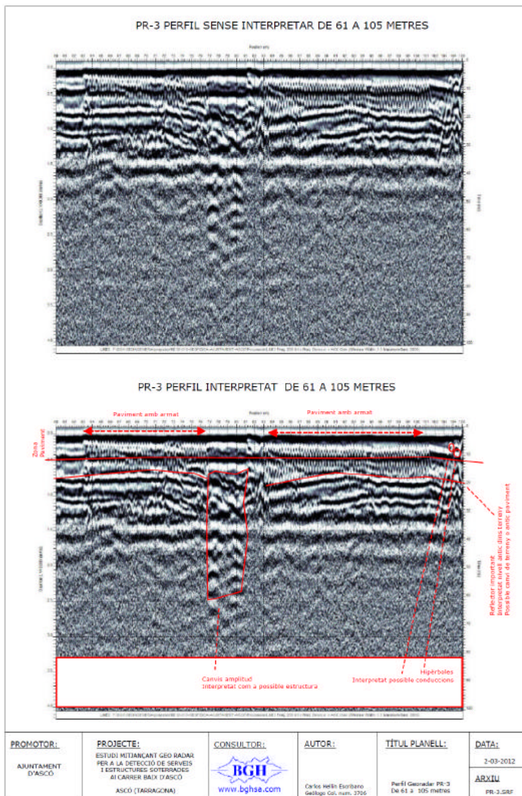
Figura 7. PR-3 PERFIL GEORADAR. Carrer de Baix. Costat oest. De 61 a 105 metres.
