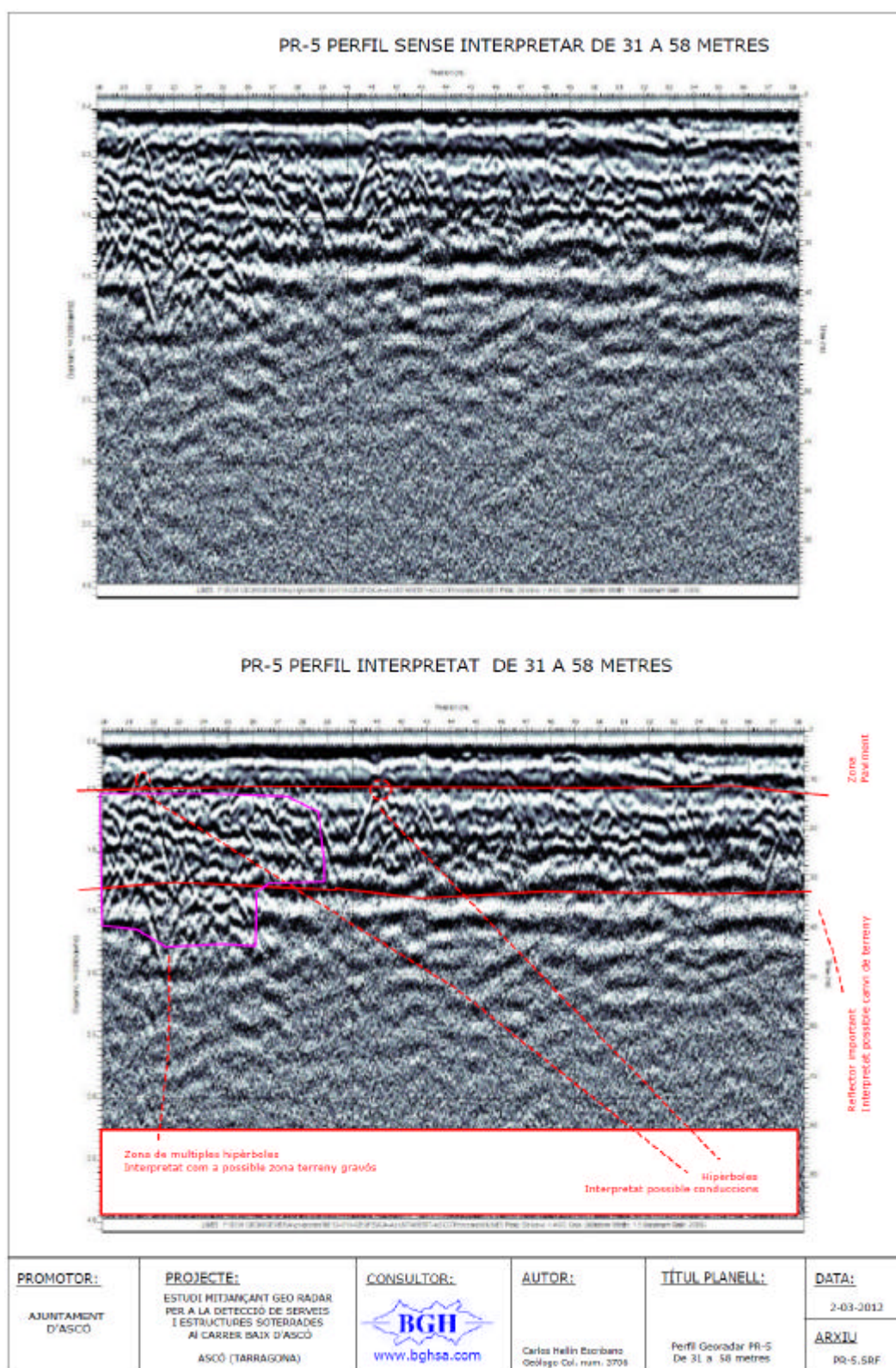
Figura 9. PR-5 PERFIL GEORADAR. Carrer de Baix. Costat est. De 31 a 58 metres.
