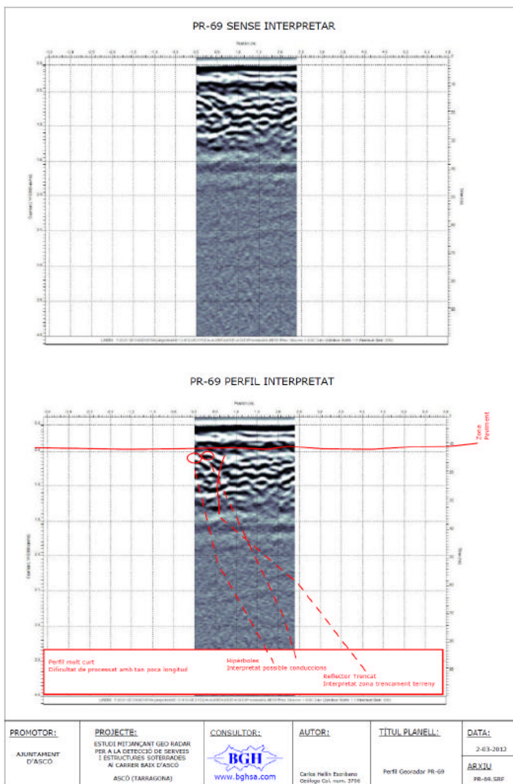
Figura 42. PR-69 PERFIL GEORADAR. Transversal en el segon carrer perpendicular al Carrer de Baix al sud.
