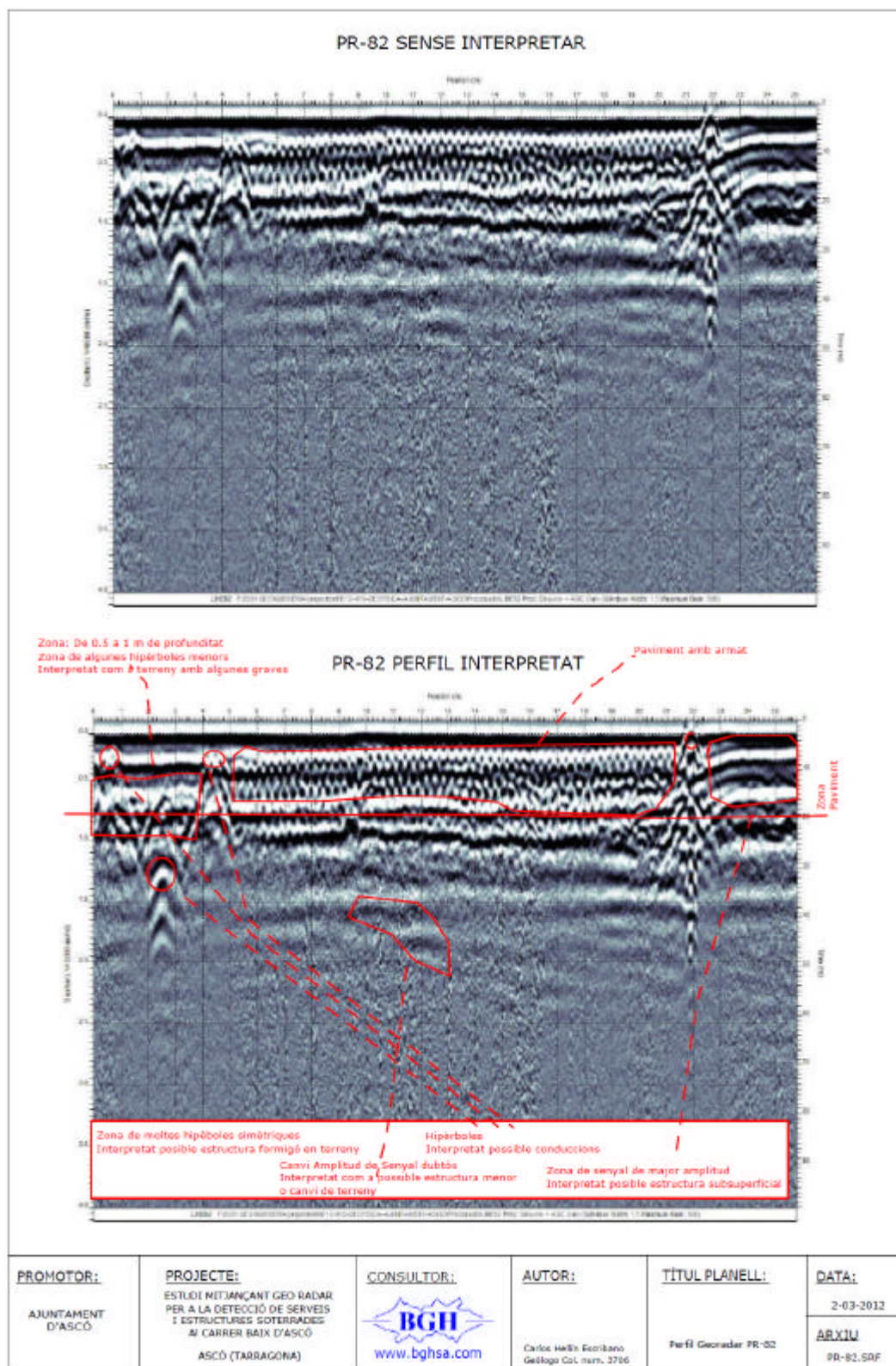
Figura 52. PR-82 PERFIL GEORADAR. Carrer de Baix, parteix sud. Costat est.
