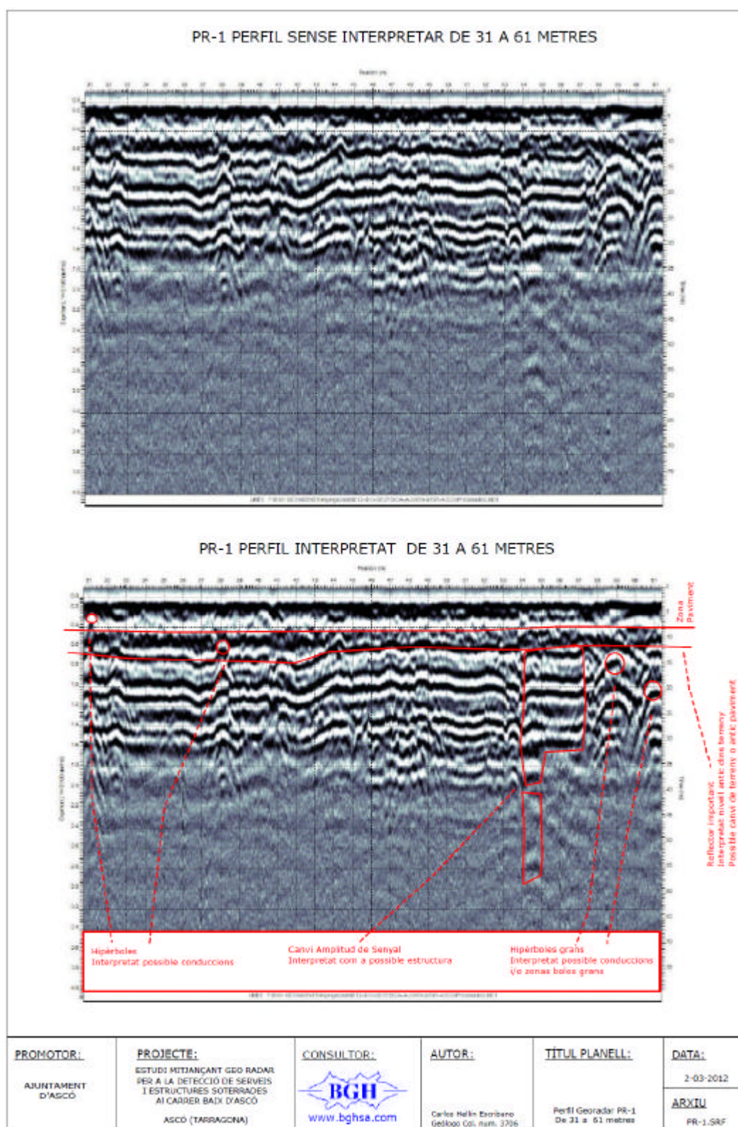
Figura 4. PR-1 PERFIL GEORADAR. Carrer de Baix. Costat oest. De 31 a 61 metres.
