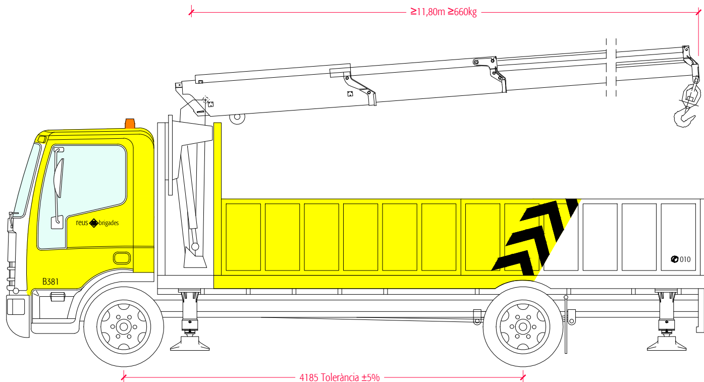
LOT 1: CAMIÓ 16 TONES. CAIXA BASCULANT HIDRÀULICA + GRUA ESCALA 1/40
