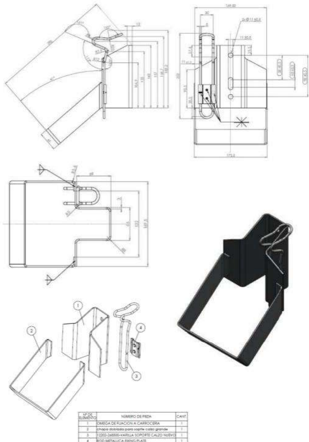
Figura 5. Soporte calzo
