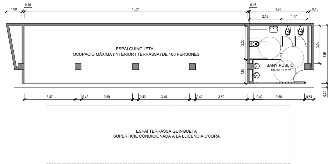
DETALL ESPAI GUINGUETA I TERRASSA e.1/150
