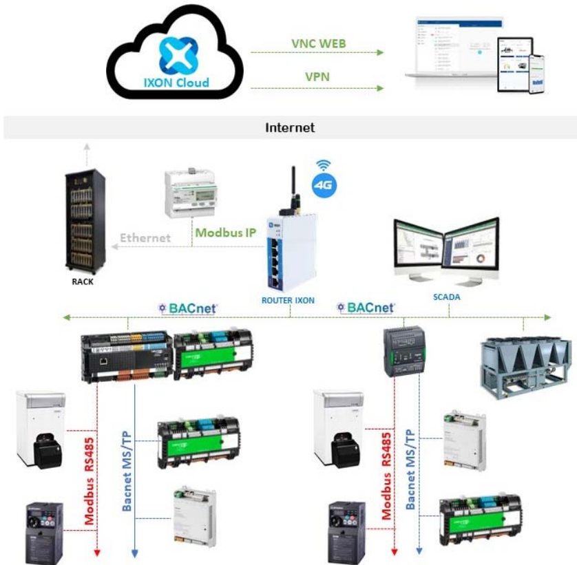
Imatge 8. Estructura Telecomandament Tipus SCADA
