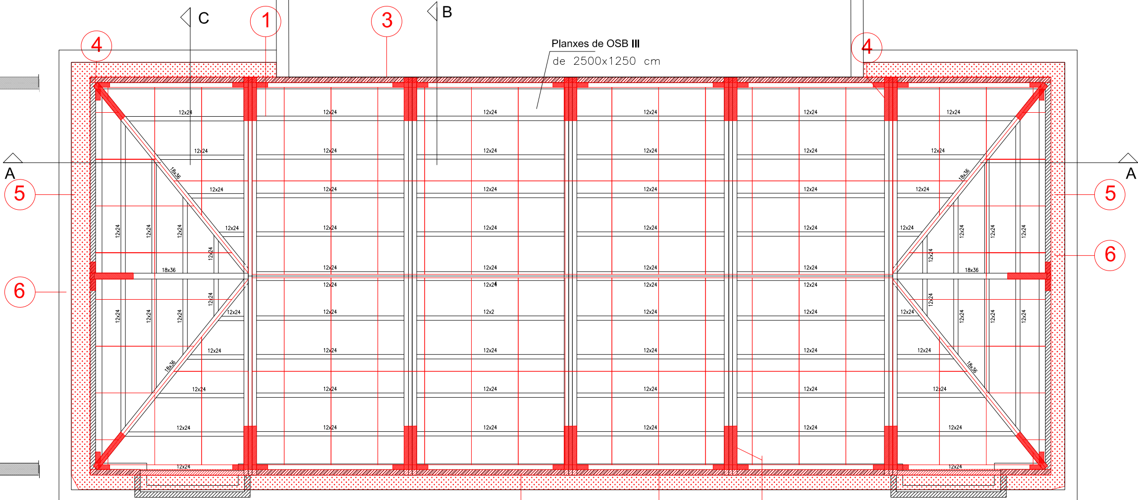
PLANTA COBERTA EDIFICI EXISTENT
