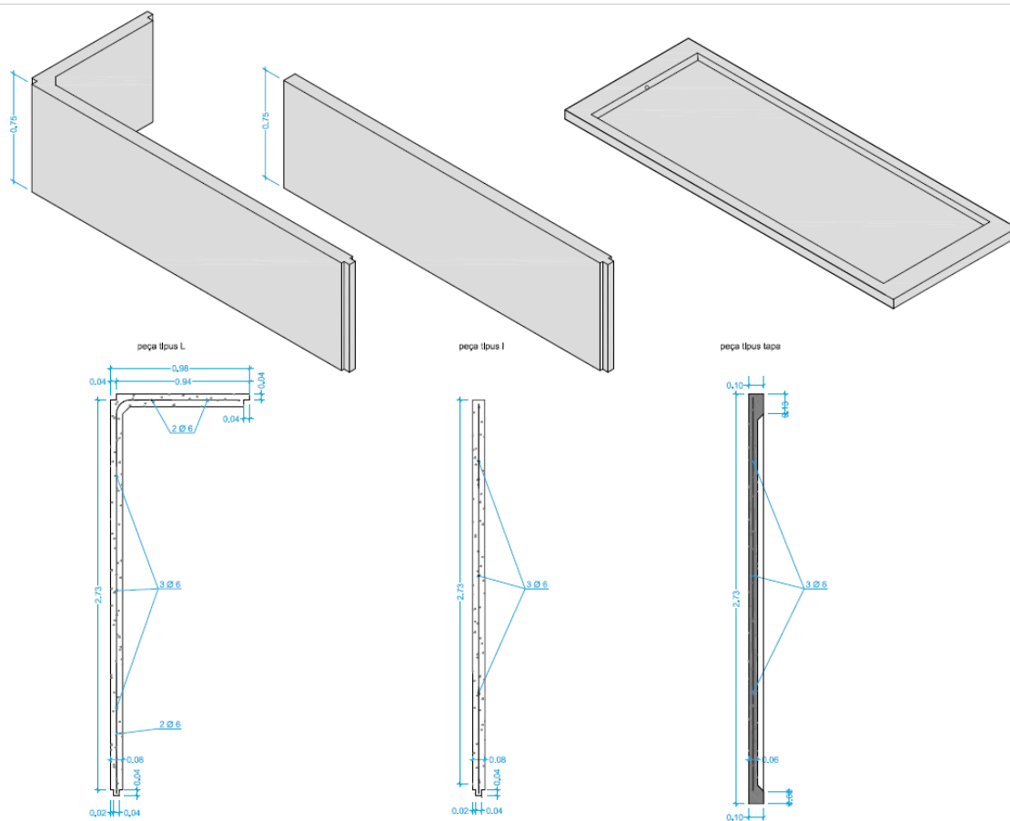
Detall peces prefabricades per a construcció de nínxols
