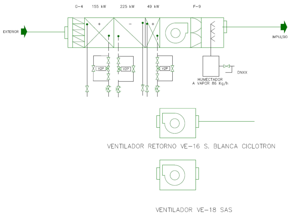
Fig. 7. Extracte esquema CL7 segons document "Esquemes aire climatitzadors ciclótró"
