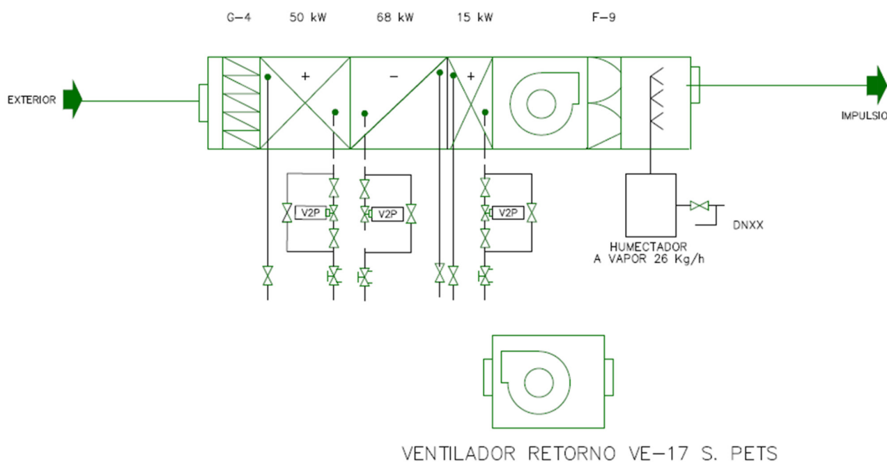
Fig. 9. Extracte esquema CL9 segons document "Esquemes aire climatitzadors ciclotró"
