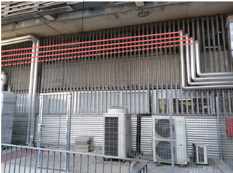
Canonades existents per attell tècnic darrera de relliga
