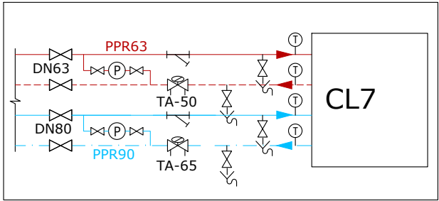
DETALL A: VALVULERIA UTAs
