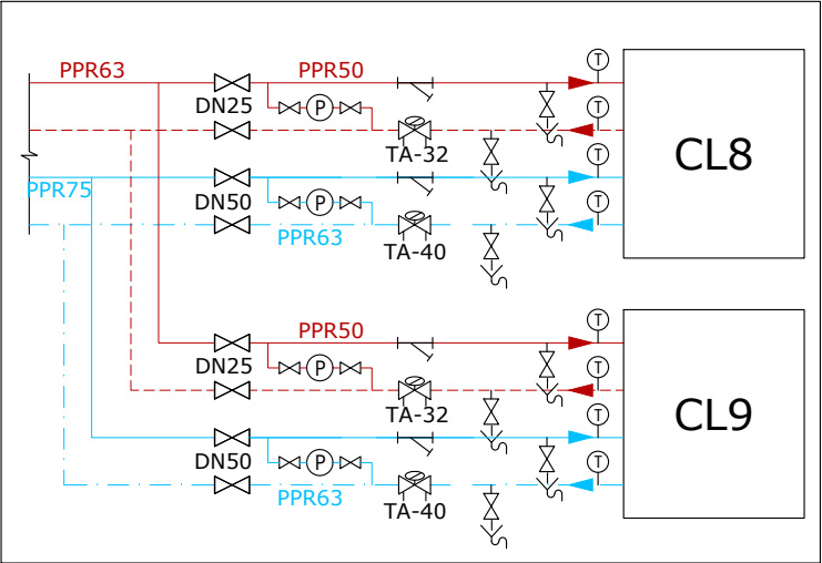
DETALL B: VALVULERIA UTAs
