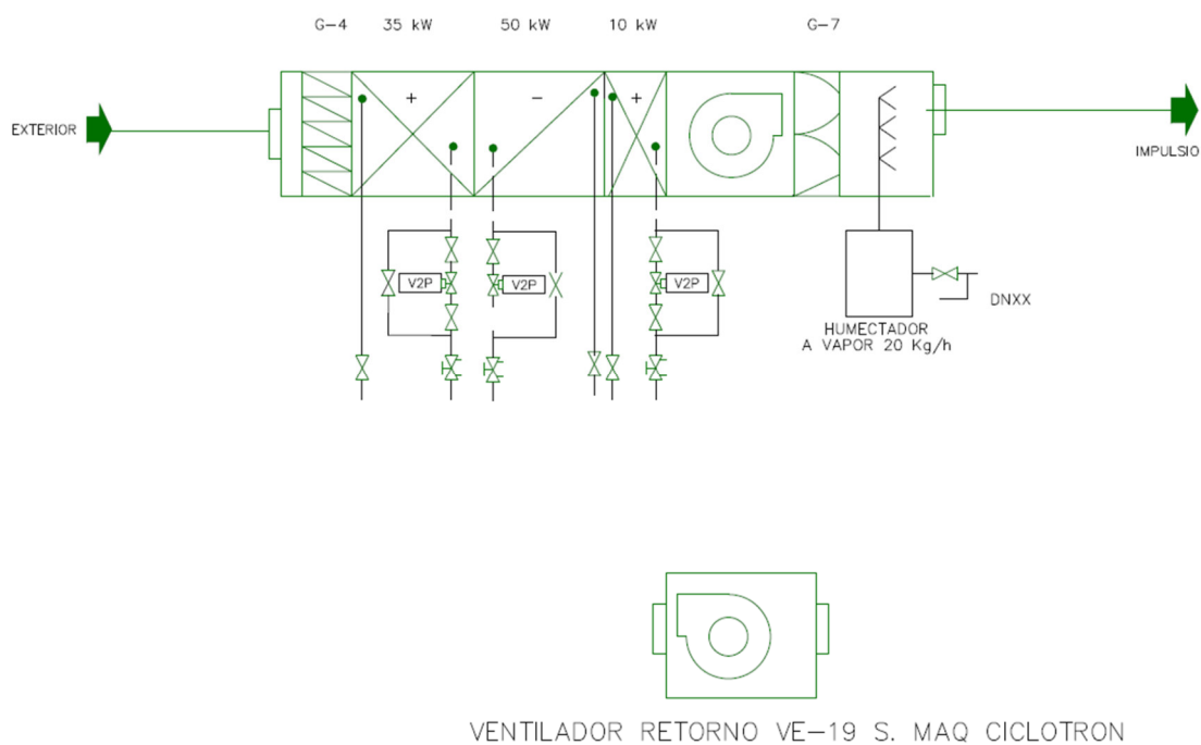
Fig. 8. Extracte esquema CL8 segons document "Esquemes aire climatitzadors ciclótró"
