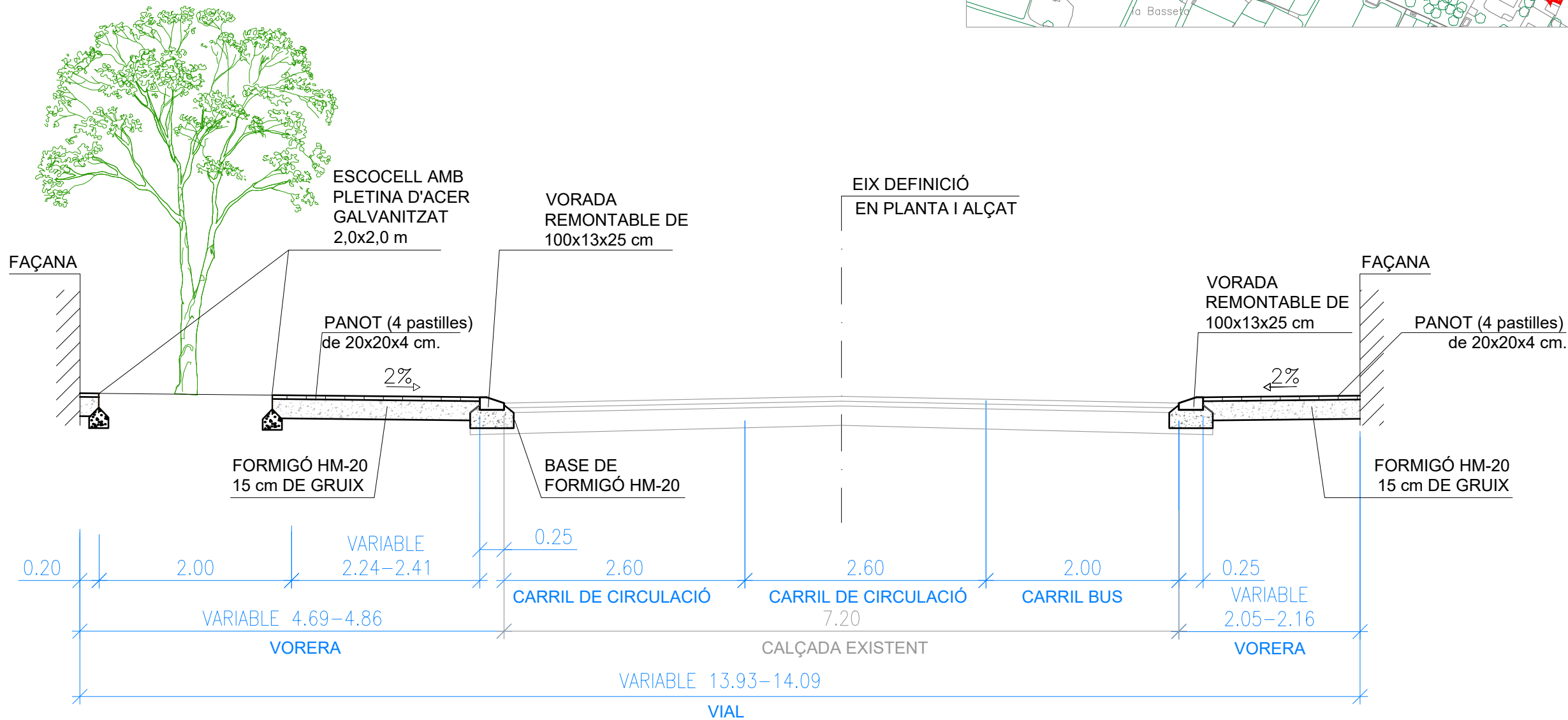
SECCIÓ S3 E:1/50
