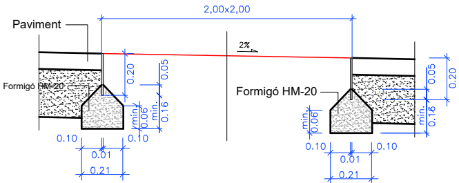
Secció A-A'
