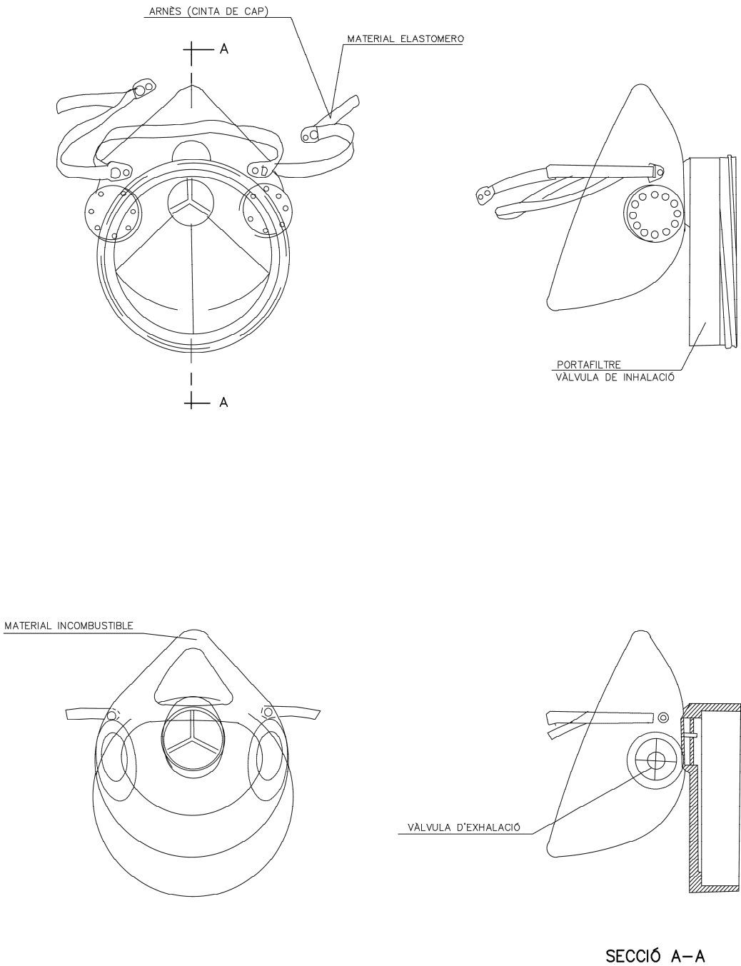
SECCIÓ A-A
