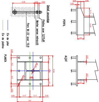
DETALL PLANTA S-5, S-10, S-11, S-16 I S-18
