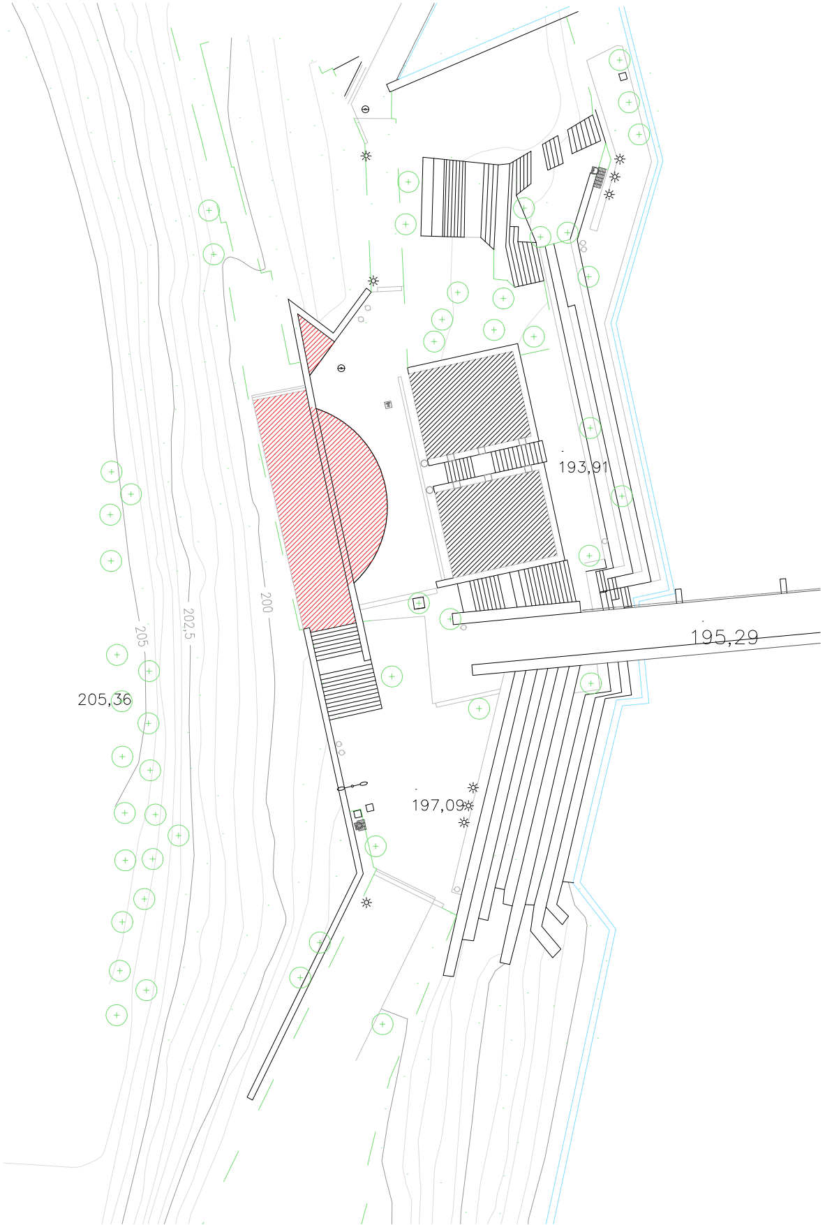
EMPLAÇAMENT e: 1/500
