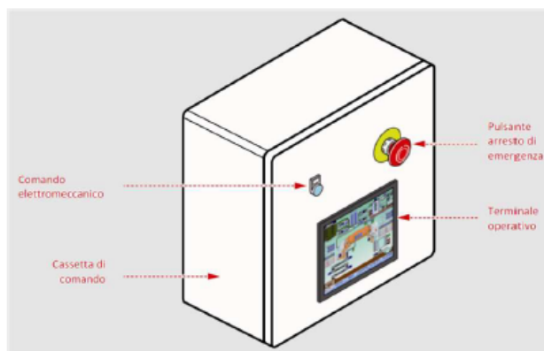
Quadre elèctric centrífuga
