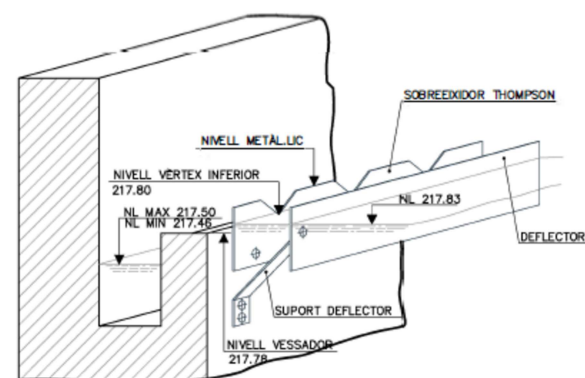
DETALL "X" S/E
