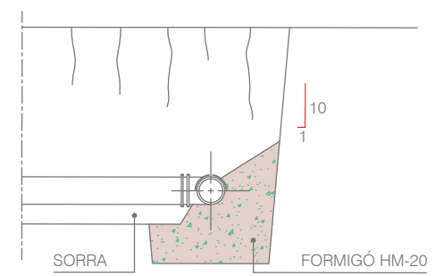
SECCIÓ B-B'
