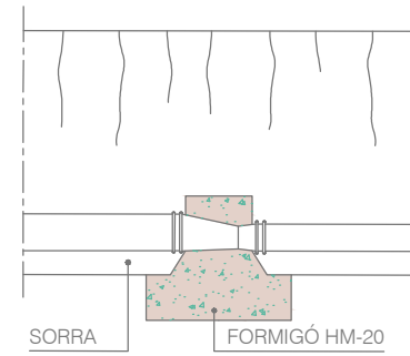
SECCIÓ C-C'
