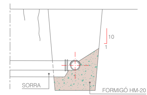
SECCIÓ A-A'
