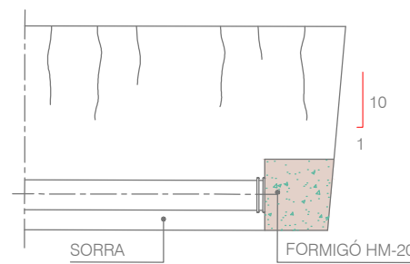
SECCIÓ D-D'
