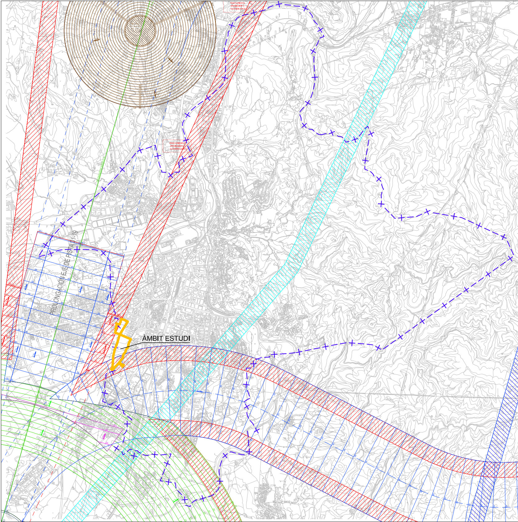
DETALL ÀMBIT TERME MUNICIPAL DE GIRONA SERVITUDS D'INSTAL·LACIONS RADIOELÈCTRIQUES
