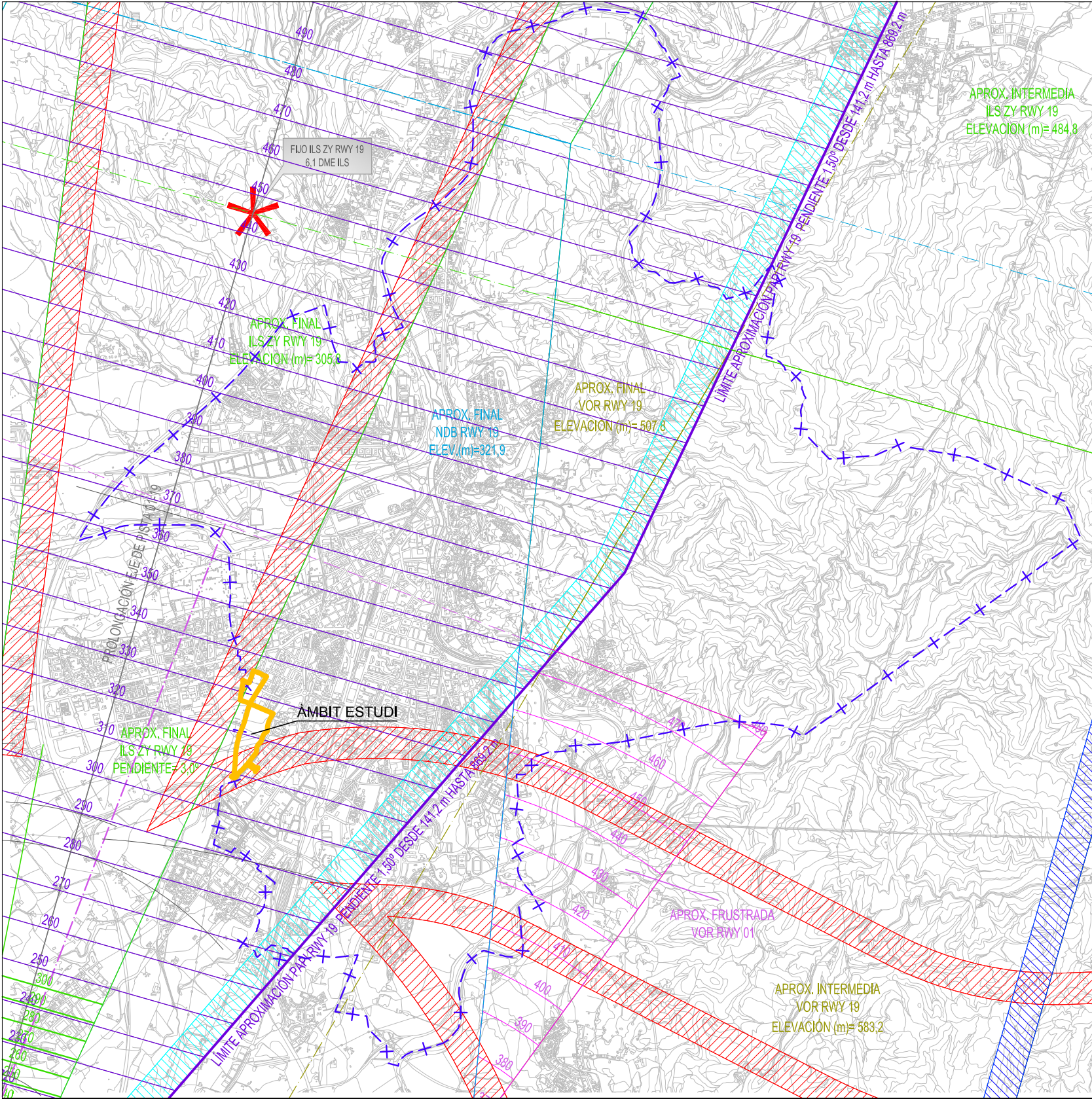
DETALL ÀMBIT TERME MUNICIPAL DE GIRONA SERVITUDS OPERACIÓ AERONAUS
