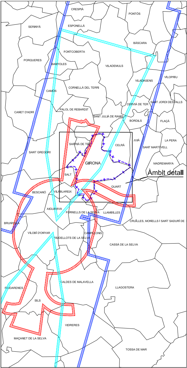
AFFECTACIÓ SERVITUDS AERONÀUTIQUES AEROPORT DE GIRONA-COSTA BRAVA
