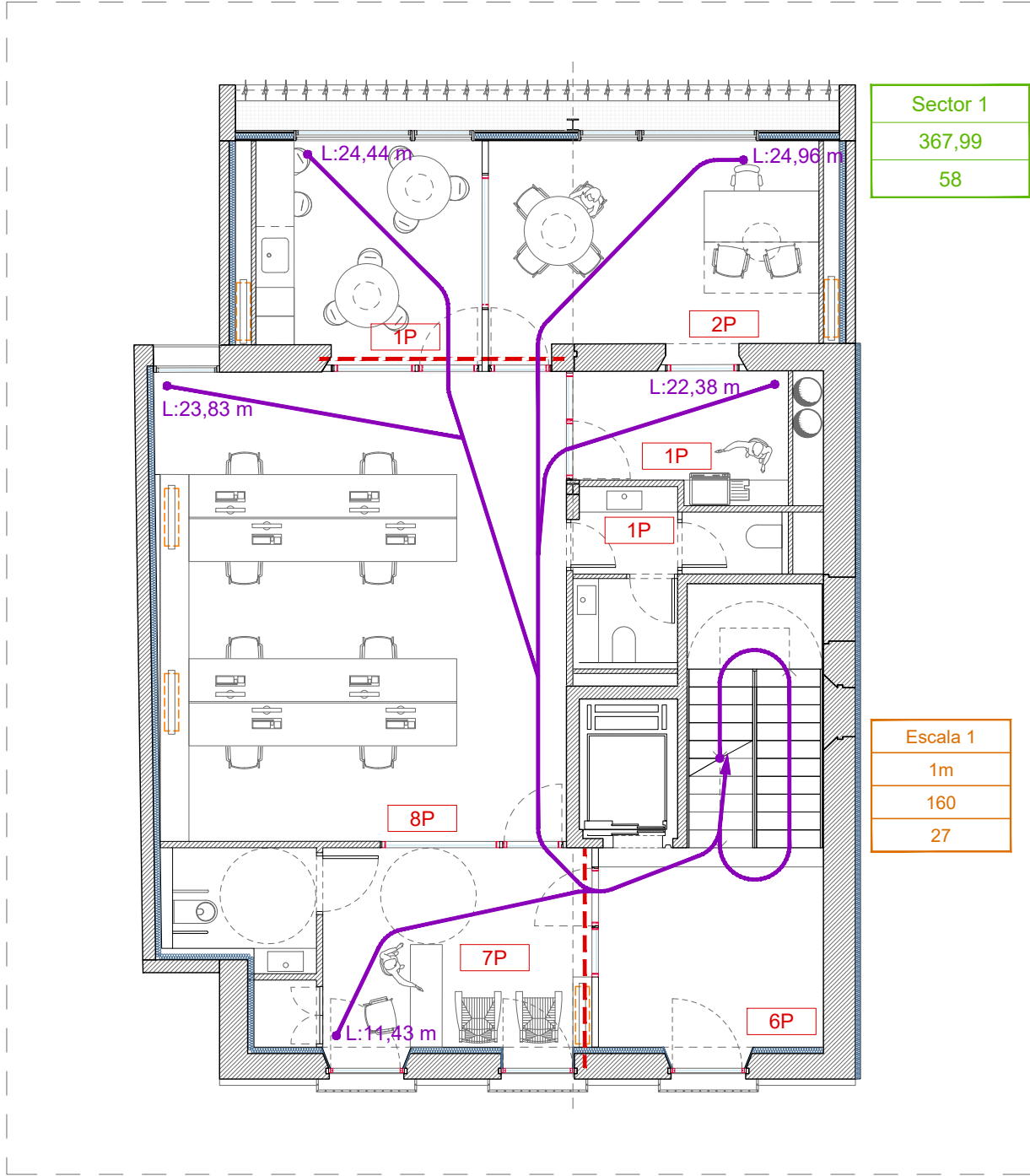
PLANTA PRIMERA
