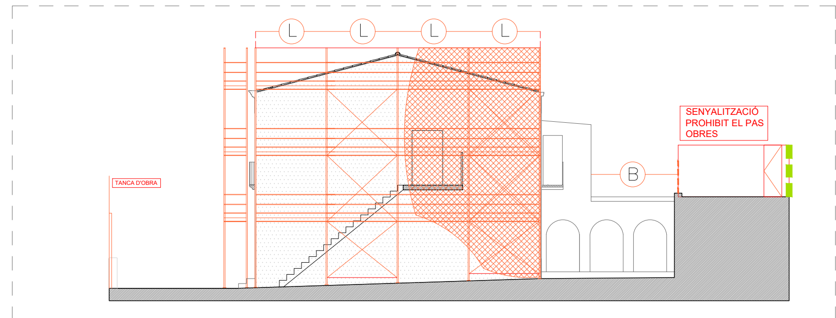
SECCIÓ S2-S2' E: 1/150
