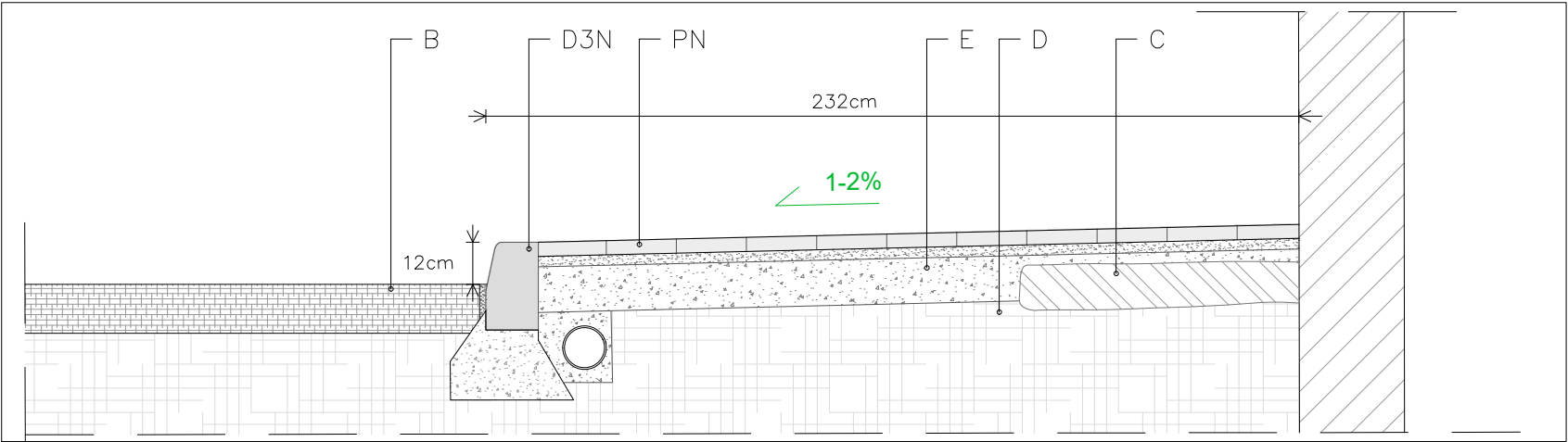
SECCIÓ TIPUS VORERA AMPLIADA DETALL ESQUEMA (I-20)
