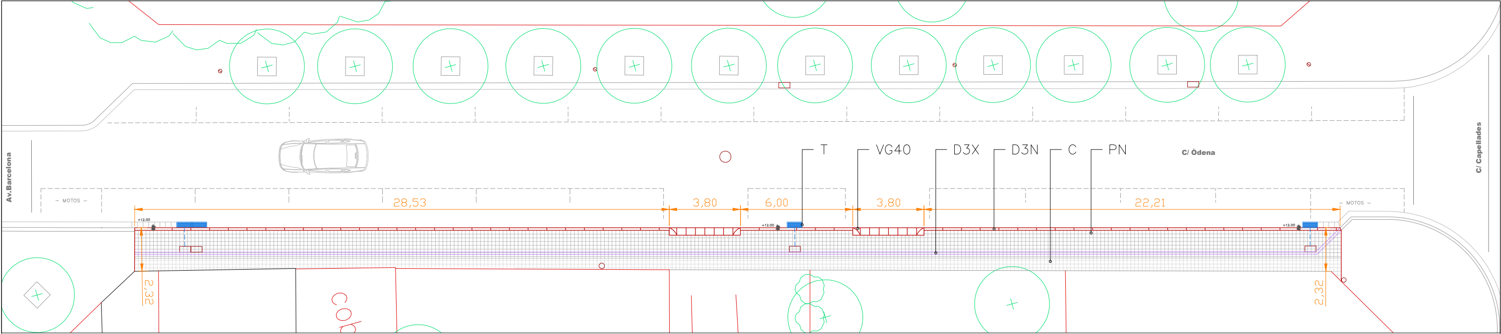
VORERA EST ÒDNA TRAM NORD (I-200)
