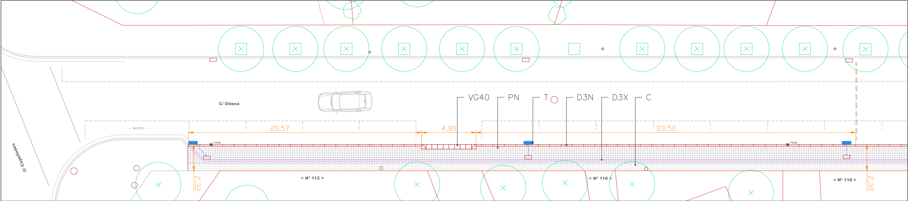
VORERA EST ÒDENA PART SUD (I-200)
