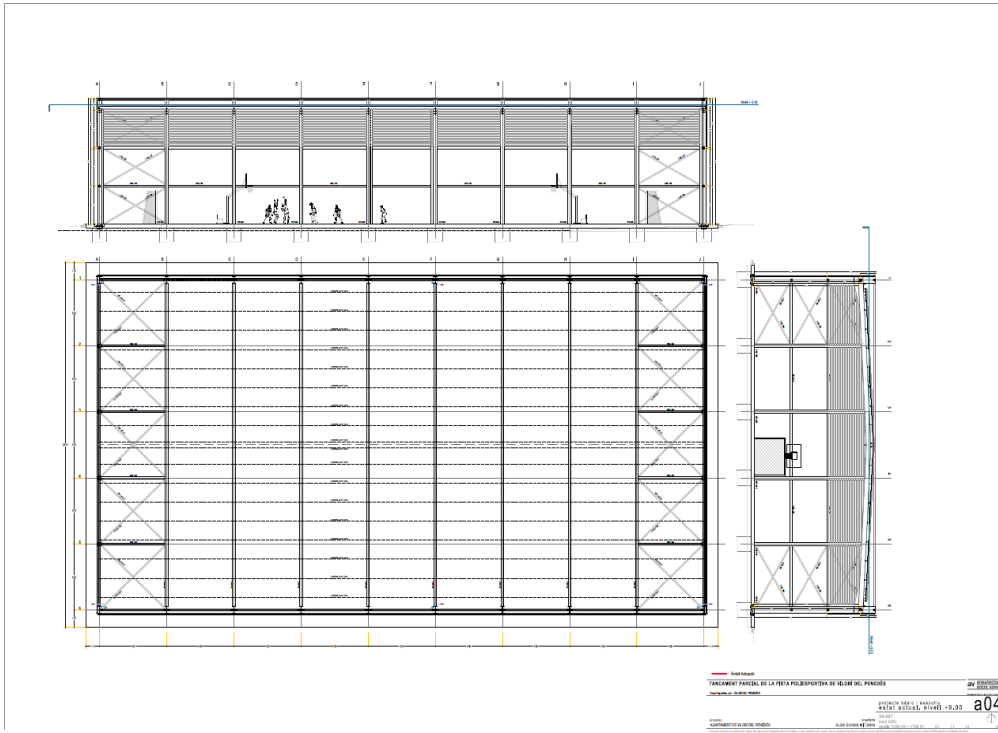
Planta encavallades edifici El Centre
