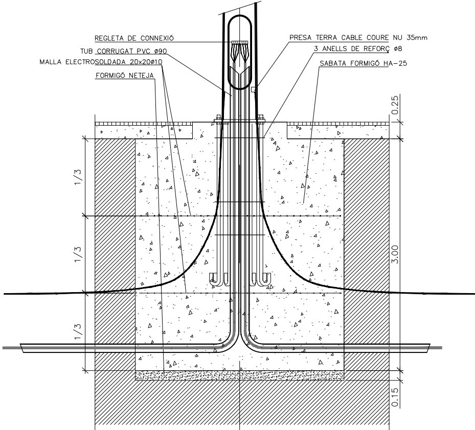
SECCIÓ
