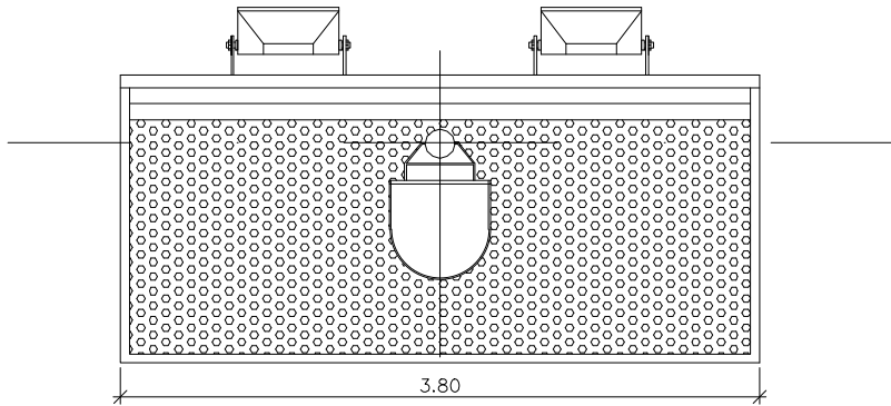
GALERIA SUPERIOR
