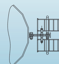
DESCANSILLO ABATIBLE
