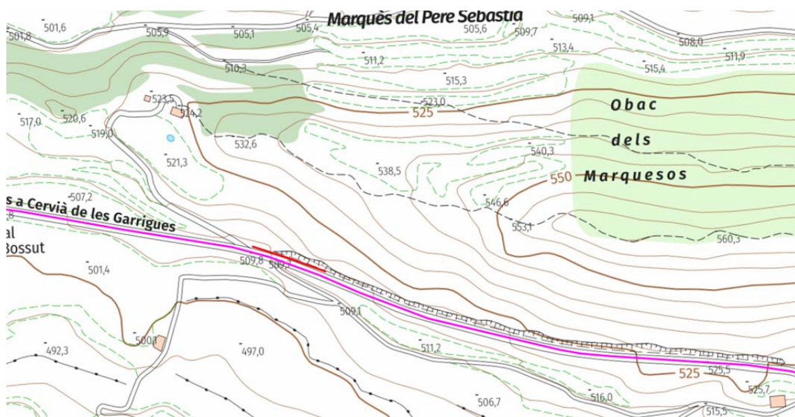
Situació tram de talús pk 2+875 en la pista a Castellans (TM Cervià de les Garrigues)
