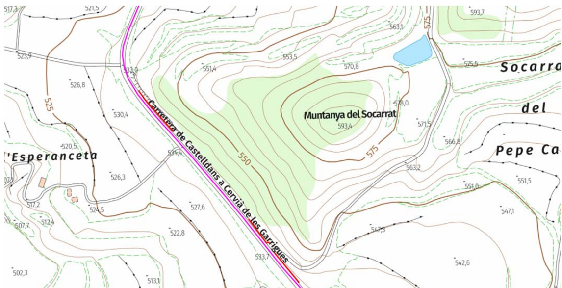
Situació de l'indret d'estabilització de talussos en la pista a Castellans (TM Cervià de les Garrigues)
