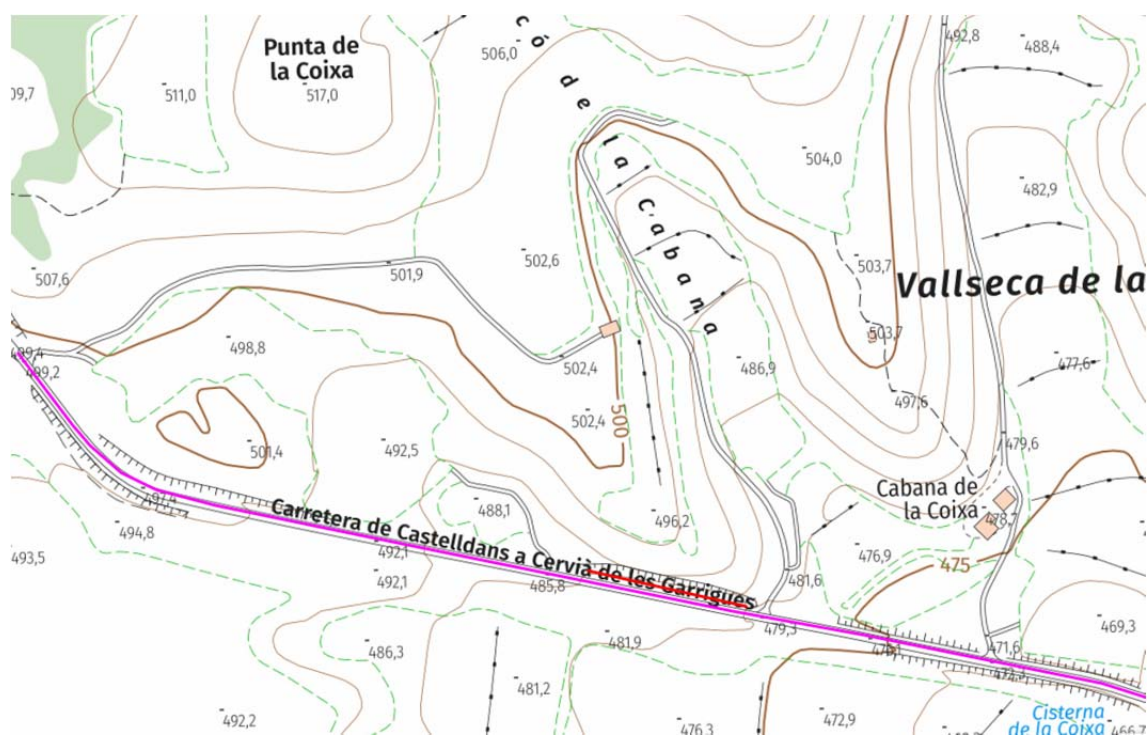
Situació tram de talús pk 5+850 en la pista a Castellldans (TM Cervià de les Garrigues)
